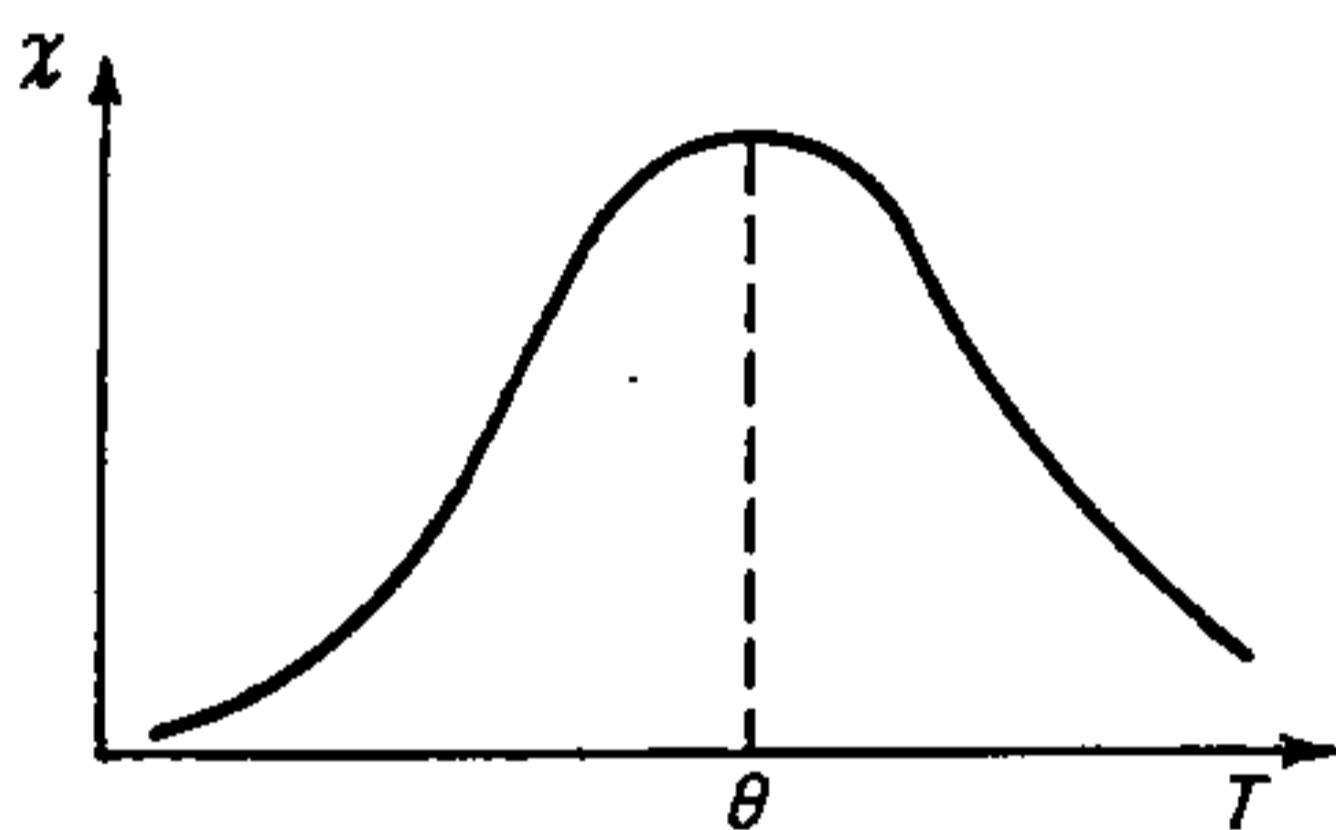
Рыс. 30.1.3. Характар тэмпературнай залежнасці магнітнай успрымальнасці антыферамагнетыка ( \theta — пункт Неэля).
