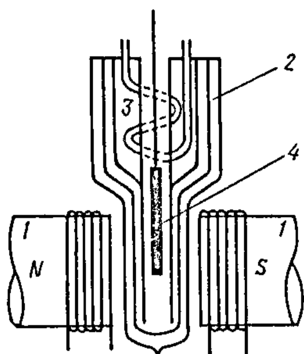
Рыс. 30.1.6. Прылада для вымярэння магнітнай успрымальнасці ў інтэрвале тэмператур ад -190 да +100 °С:
