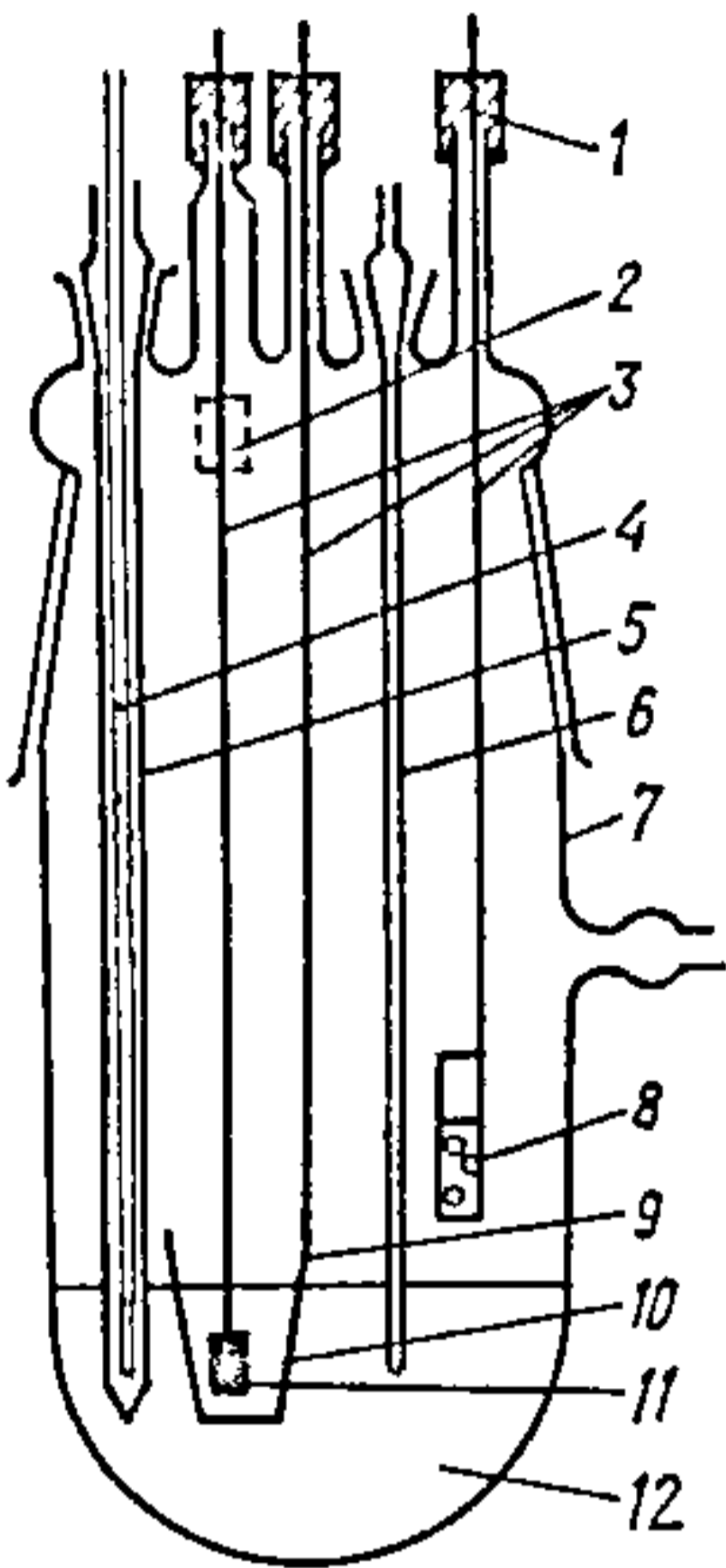
Рыс. 13.3.1. Ячэйка для вымярэння раўнаважных патэнцыялаў металаў у раўнаважных солях:
