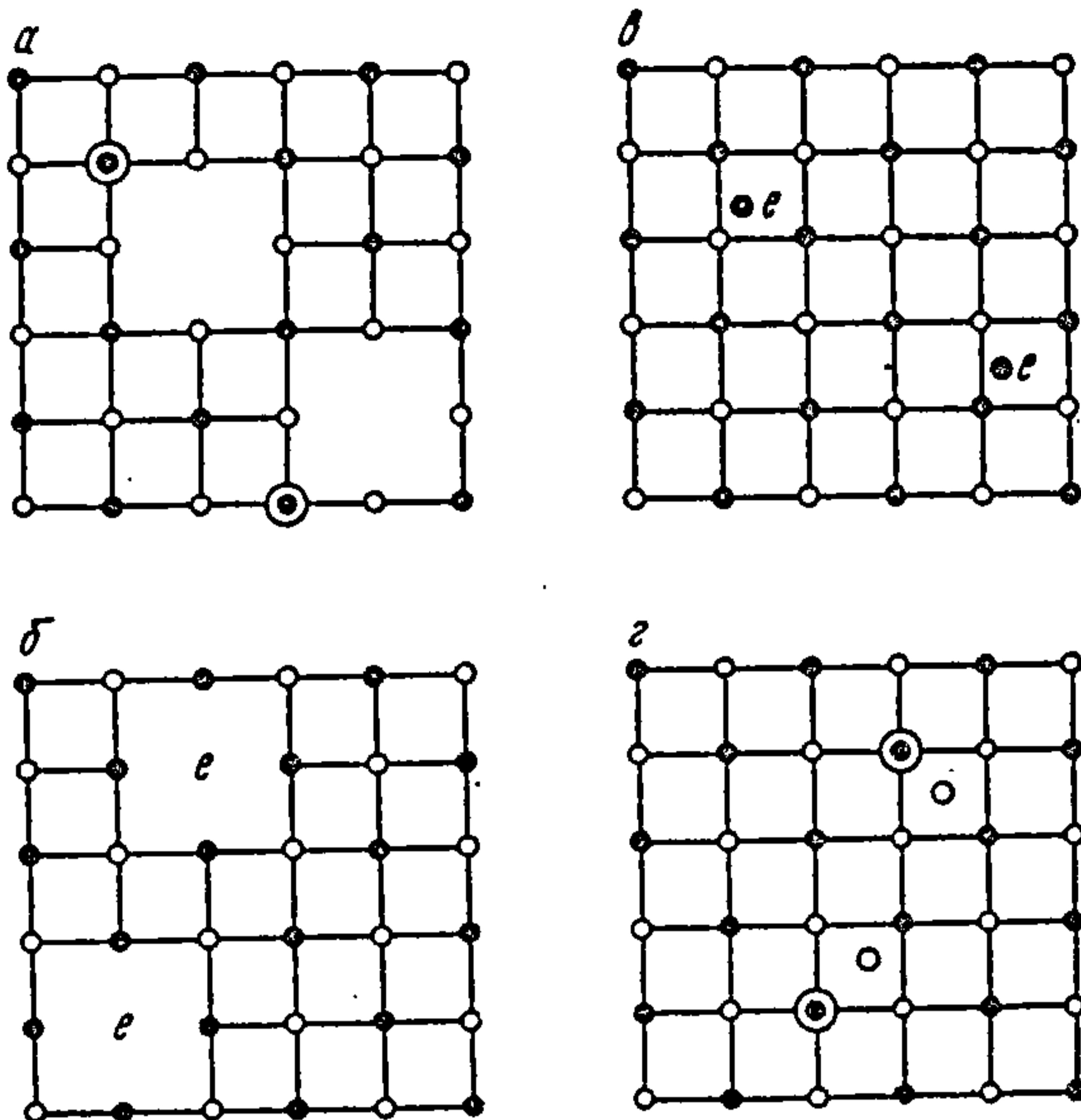
Рис. 27.2.1. Типы рашотак нестехіометричных злучэнняў: а — вакансіі катыёнаў з зарадам +1 , але некаторыя катыёны ў вузлах рашоткі маюць зарад +2 ; б — вакансіі аніёнаў з захопам электронаў e ; в — катыёны ўкаранення з захопам электронаў e ; г — аніёны ўкаранення, зарад якіх кампенсуецца часткай катыёнаў з зарадам +2 .
