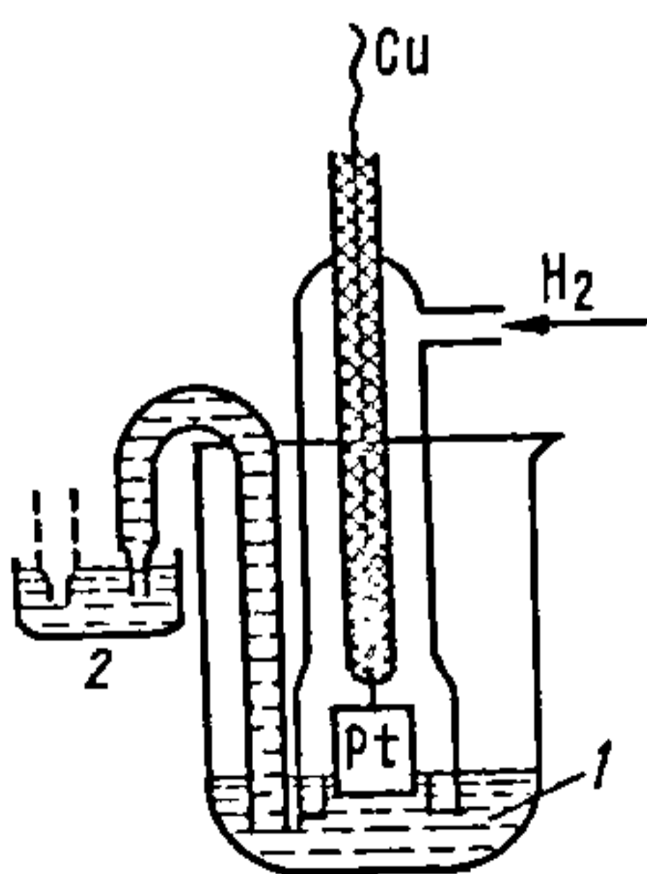
Рыс. 13.2.1. Схема вадароднага электрода:
