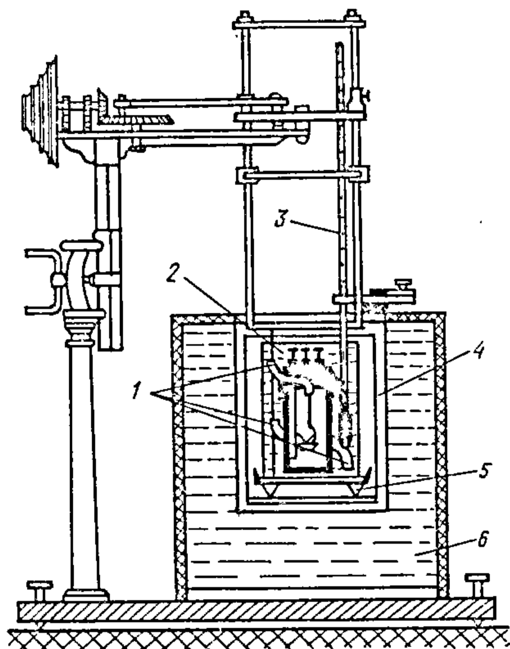
Рыс. 4.11.4. Разрэз каларыметра з бомбай спальвання: 1 — мяшалка; 2 — каларыметрычны сасуд з вадкасцю; 3 — тэрмометр; 4 — металічны стакан; 5 — эбанітавая падстаўка; 6 — абалонка.
