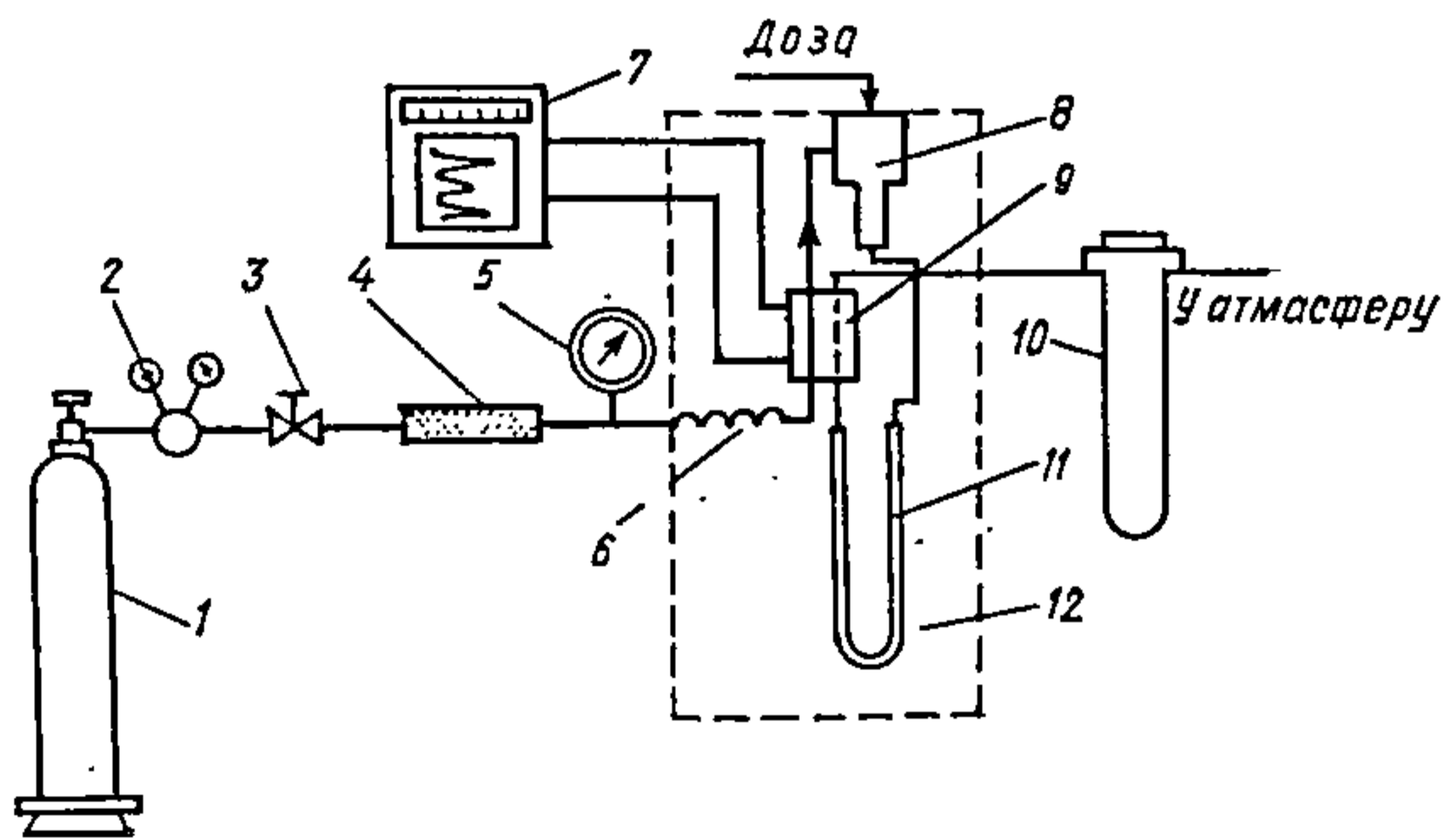
Рыс. 15.2.2. Тыповая схема лабараторнай газахраматаграфічнай устаноўкі:
