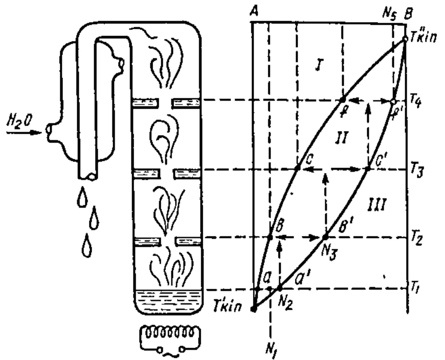
Рис. 8.4.2. Схема рэктыфікацыйнай калоны: I — вобласць іспавання вадкасці; II — раўнаважны стан вадкасць — пара; III — вобласць іспавання вадкасці.
