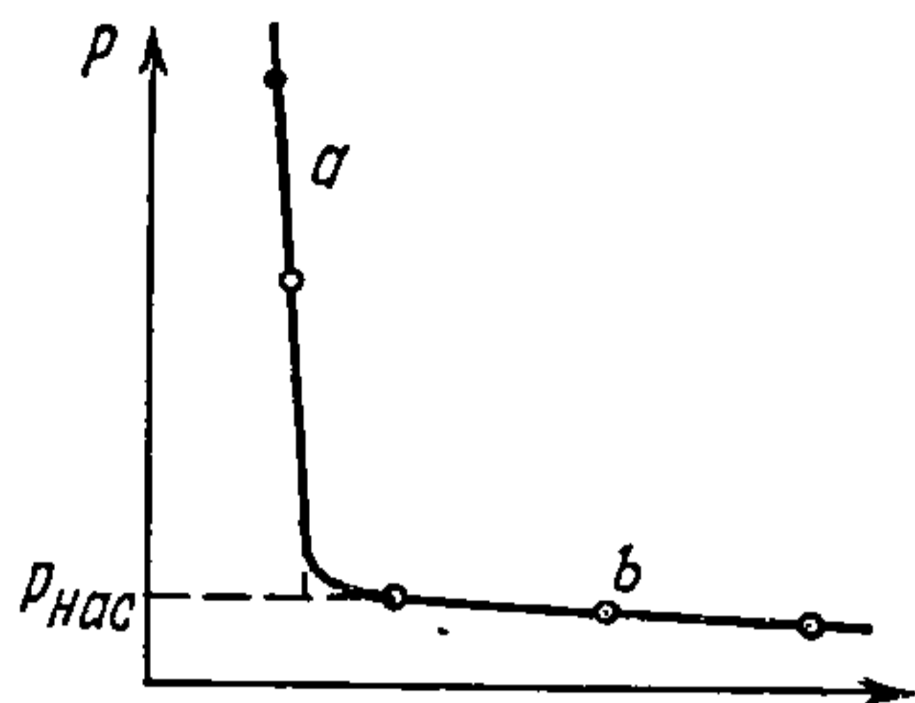
Рис. 6.5.2. Графік залежнасці ціску аргону ад паказанняў гальванометра:
