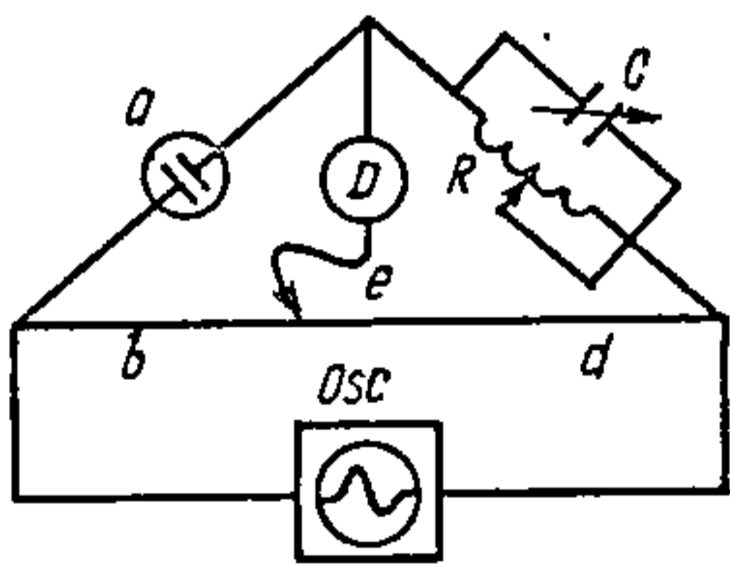
Рыс. 13.1.2. Схема маста пераменнага току:
