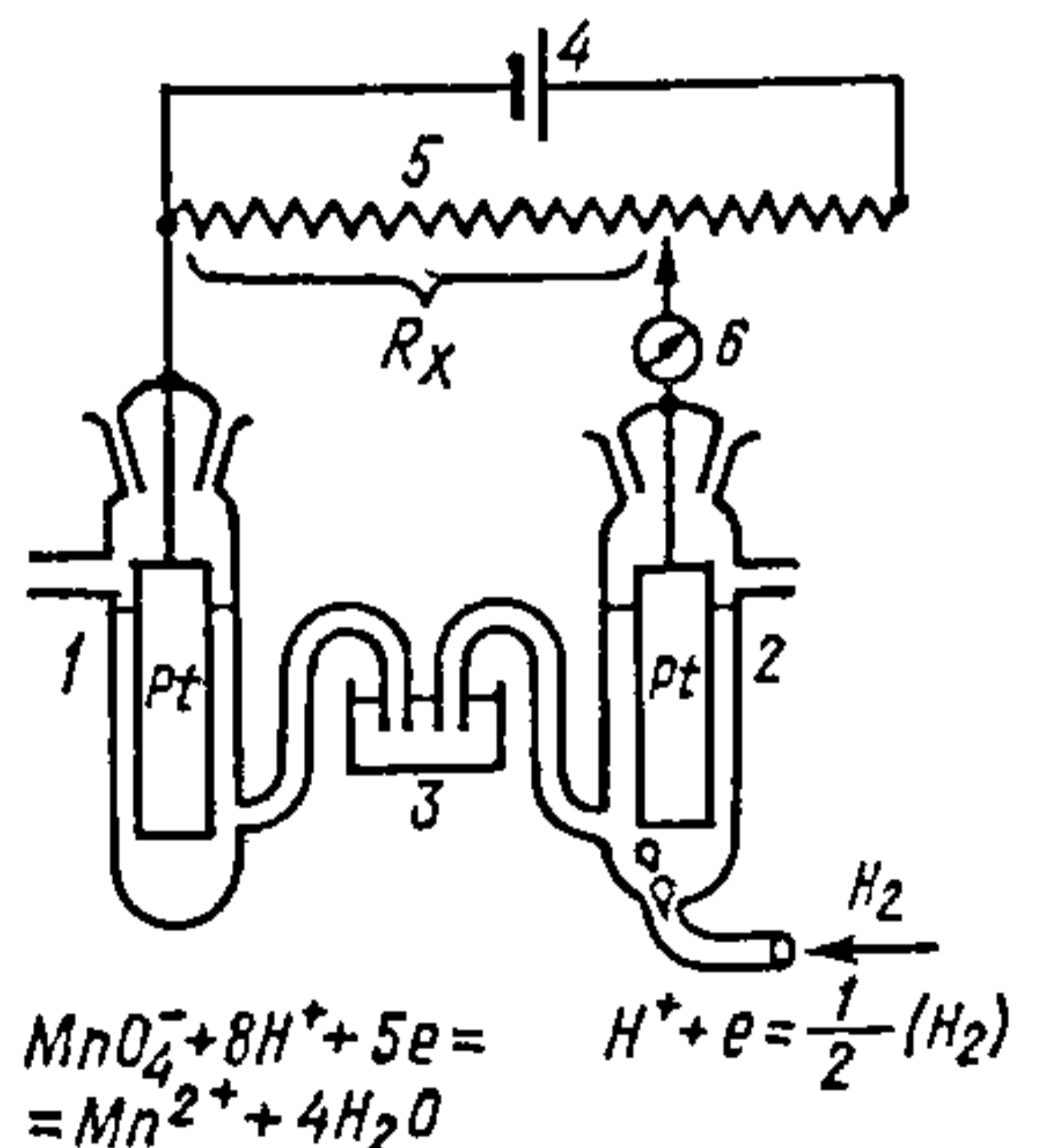
Рыс. 13.2.2. Патэнцыяметрычная схема вымярэння ЭРС гальванічнага элемента.
