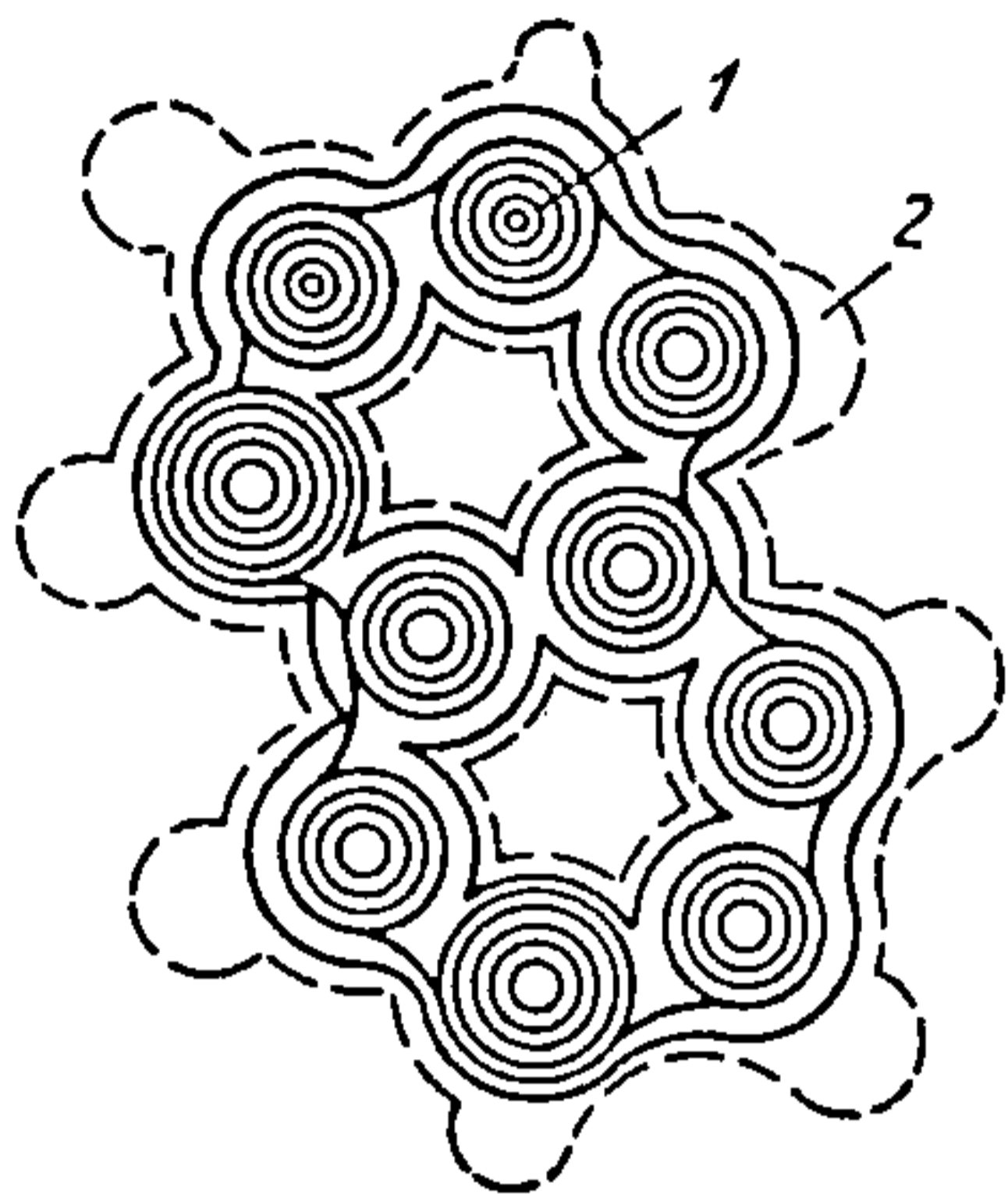
Рыс. 28.2.6. Размеркаванне электроннай шчыльнасці ў малекуле нафталіну:
