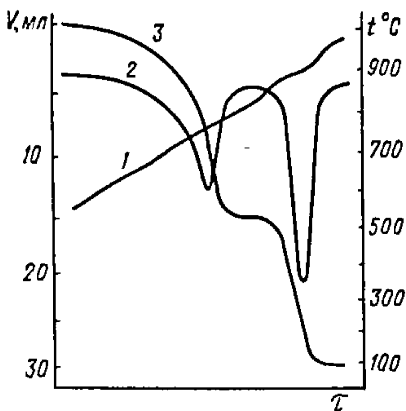
Рыс. 7.11.3. Тэрмаграма і валюмаграма раскладання \text{CaCO}_3 \cdot \text{MgCO}_3 пры награванні:
