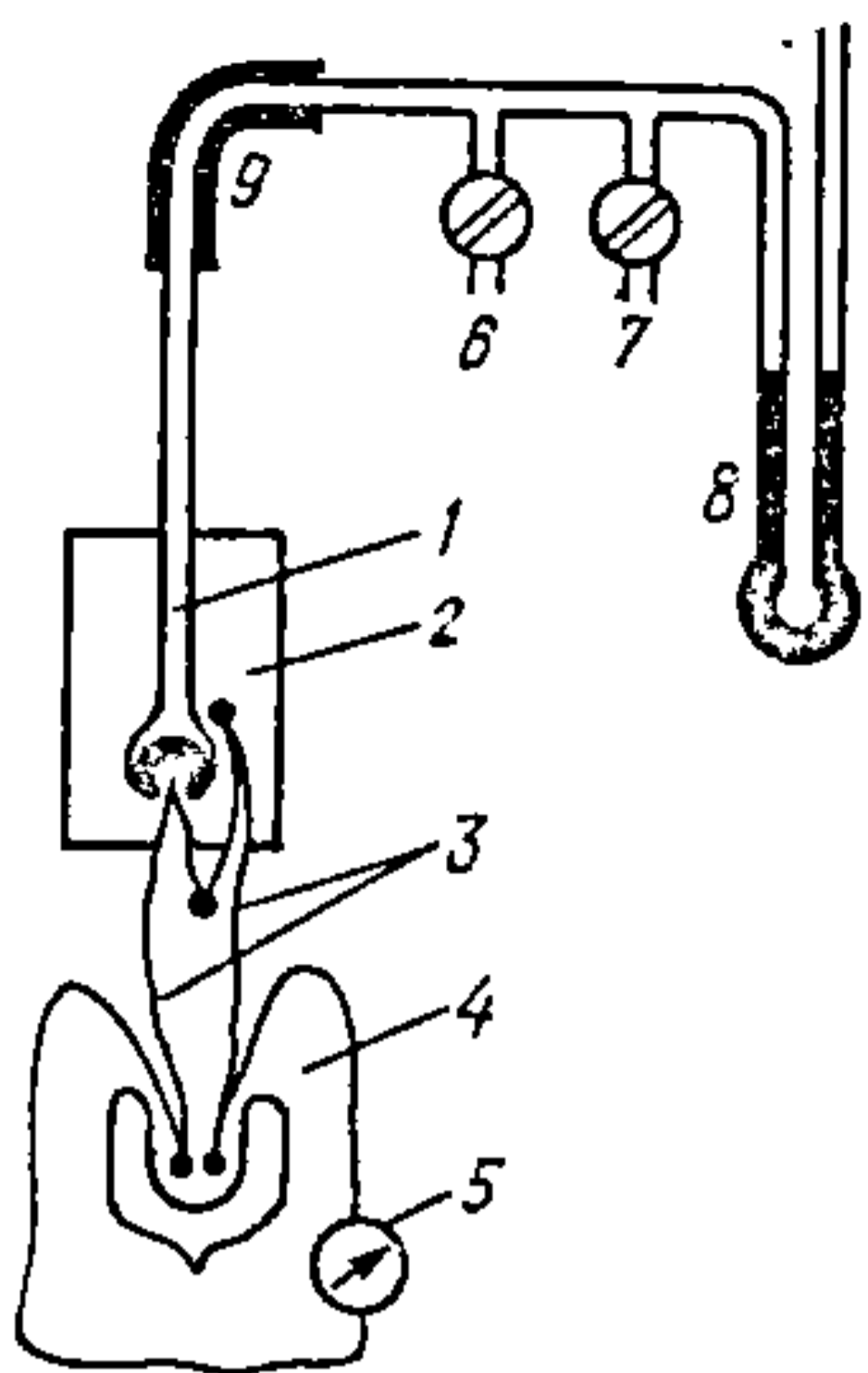
Рис. 6.5.1. Изотермичны варыянт прыбора, што працуе па метадзе пунктаў кіпення:
