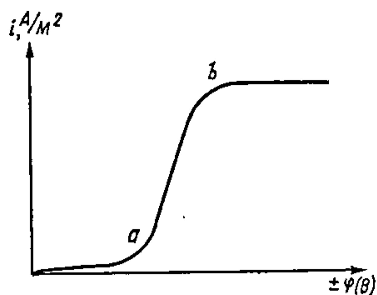
Рыс. 13.4.2. Характар палярэзацыйнай крывой.
