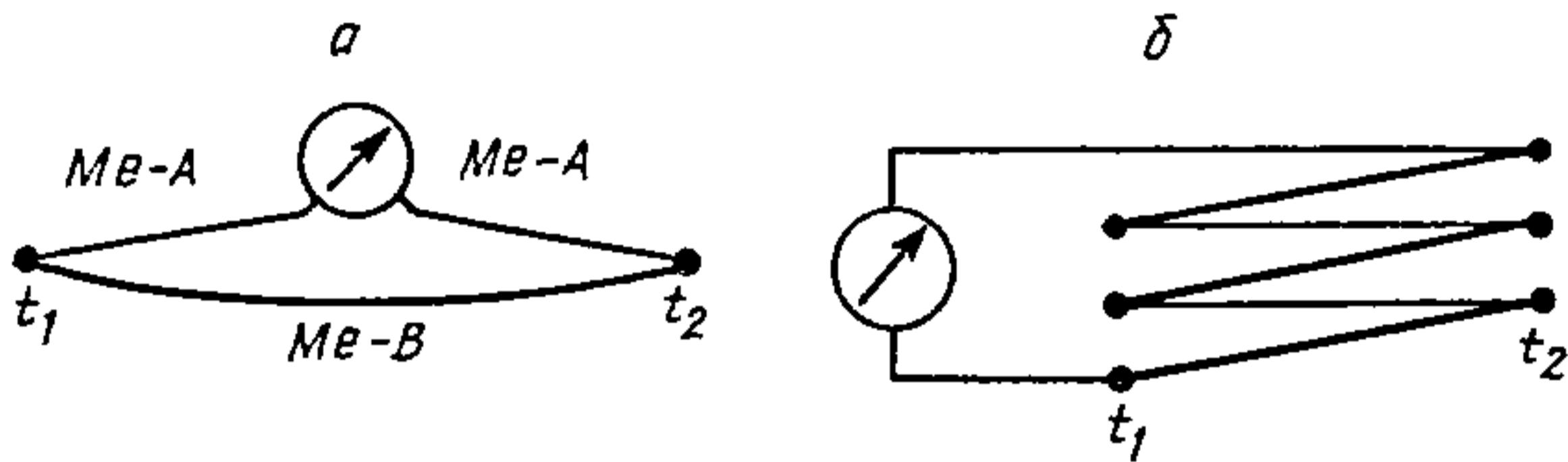
Рыс. 4.11.3. Схема тэрмапар: а — простае; б — тэрмабатарэй.
