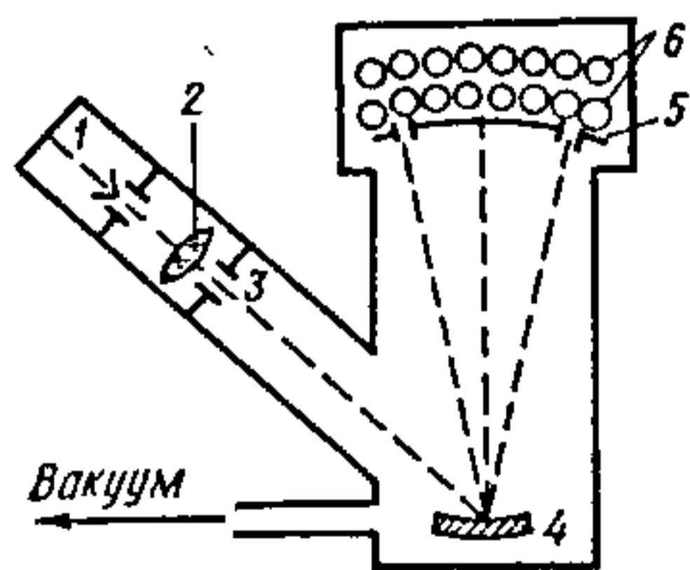
Рыс. 25.5.3. Схема вакуумнага фотаэлектрычнага спектрометра ДСФ-31 з дыфракцыйнай рашоткай: 1 — камера са штатывам; 2 — асветляльная лінза; 3 — уваходная шчыліна; 4 — дыфракцыйная рашотка; 5 — факальная паверхня з выхаднымі шчылінамі; 6 — фотамножнікі.
