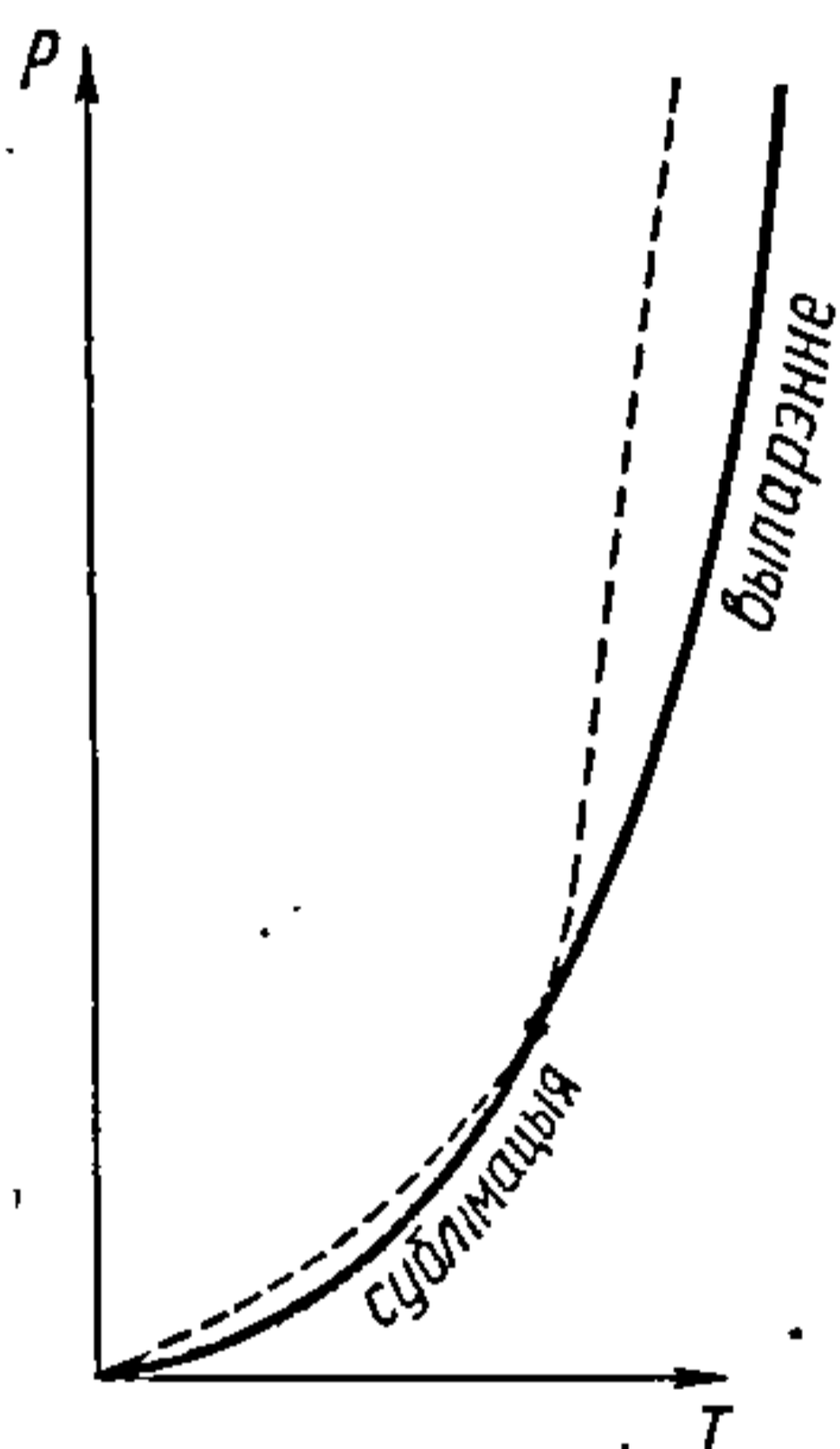
Рыс. 7.2.1. Характар залежнасці ціску насычанай пары ( p ) над цвёрдым (сублимация) і вадкім (выпарэнне) рэчывамі ад тэмпературы ( T ).
