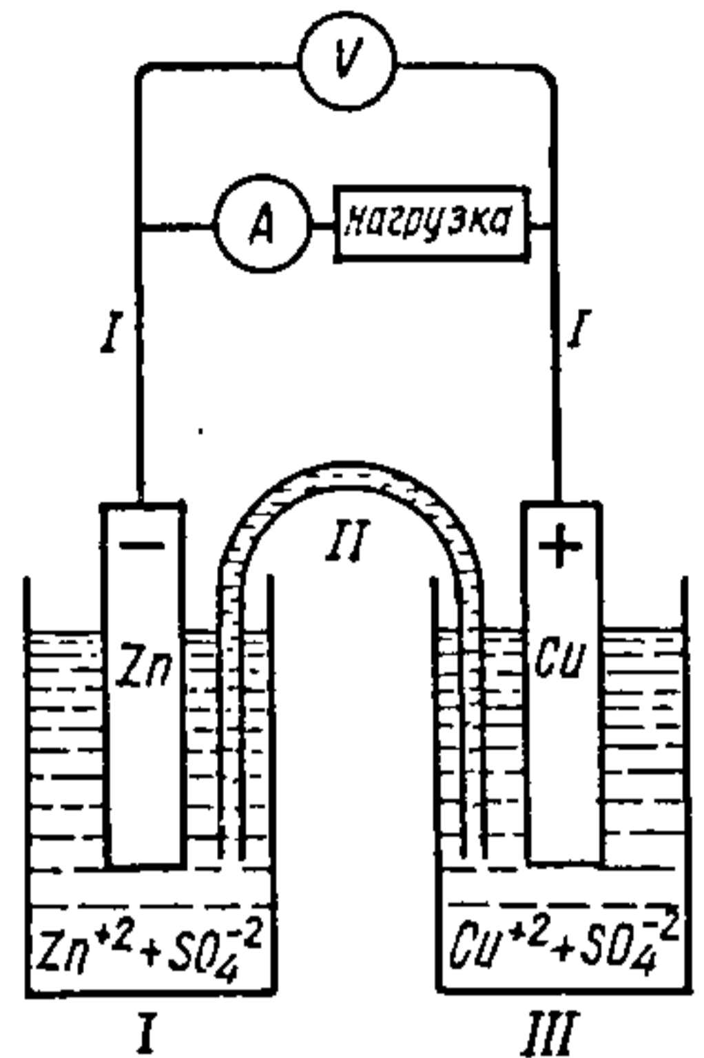
Рыс. 12.1.1. Схема гальванічнага элемента: V — прыбор для вымярэння ЭРС (патэнцыяметр або для не вельмі дакладных вымярэнняў вальтметр); A — прыбор для вымярэння сілы току (амперметр) або прыбор для вызначэння колькасці электрычнасці; I — цынкавы электрод (паўэлемент); II — электралітычны ключ (іонны праваднік); III — медны электрод (паўэлемент).
