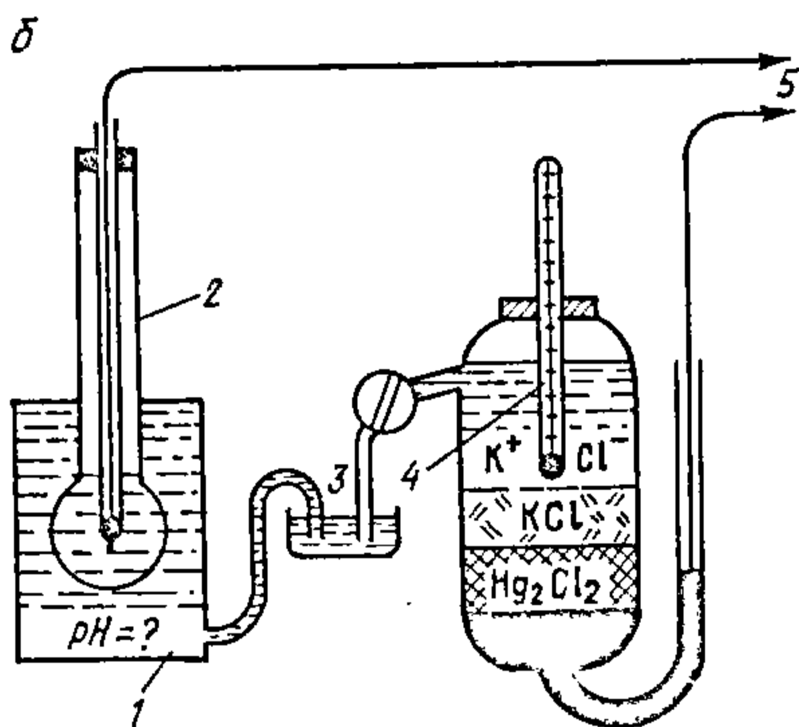
Рис. 13.2.5. Схема гальванічнага элемента са шкляным электродам для вызначэння рН:
