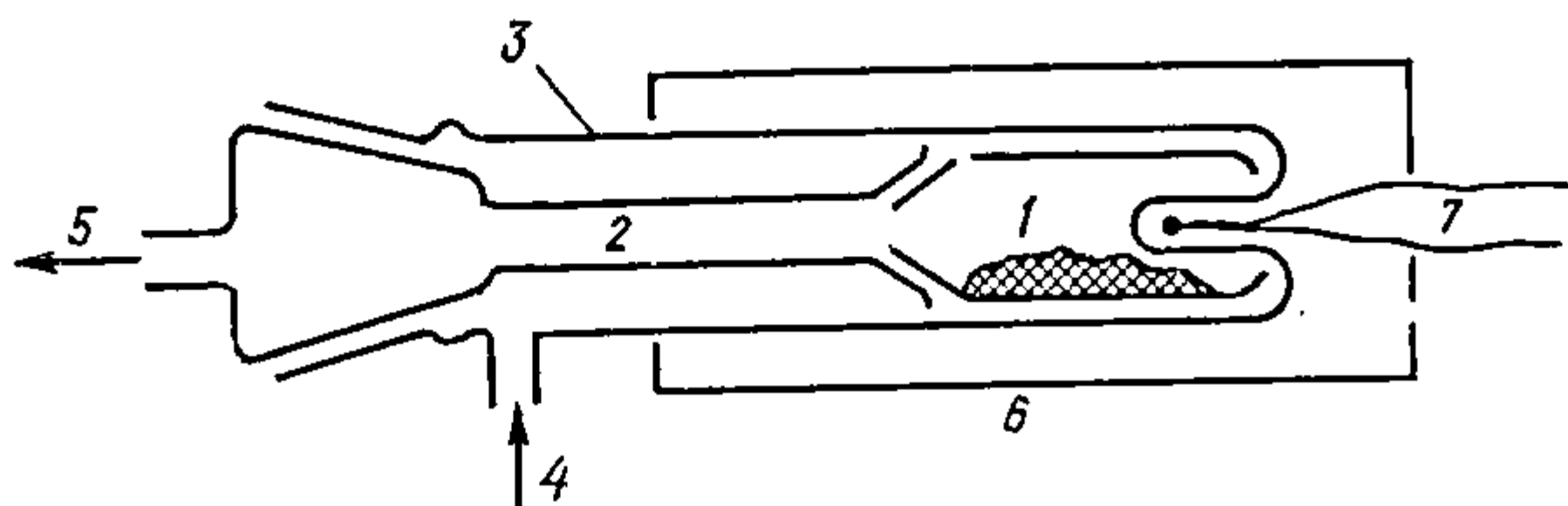
Рыс. 6.5.3. Схема прыбора, што працуе па метада газавога насычэння (патоку):
