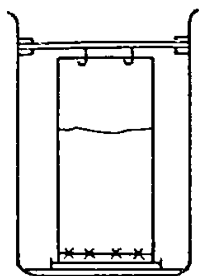
Рыс. 15.3.1. Камера для ўзыходнай ПХ з лістом храматаграфічнай паперы, падвешанай на шкляной палачцы, канцы якой замацаваны кавалачкамі жорсткай гумавай трубкі.
