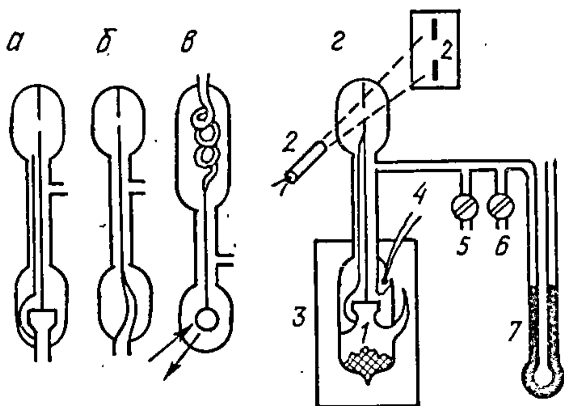
Рыс. 6.4.1. Тэнзіметр з кварцавым або шкляным нуль-манометрам: а — мембранны нуль-манометр; б — серпападобны нуль-манометр (Бурдона); в — спіральны нуль-манометр; г — тэнзіметрычная ўстаноўка: 1 — нуль-манометр; 2 — аптычнае ўстройства; 3 — тэрмастат; 4 — тэрмапара; 5, 6 — кранавая сістэма; 7 — манометр.
