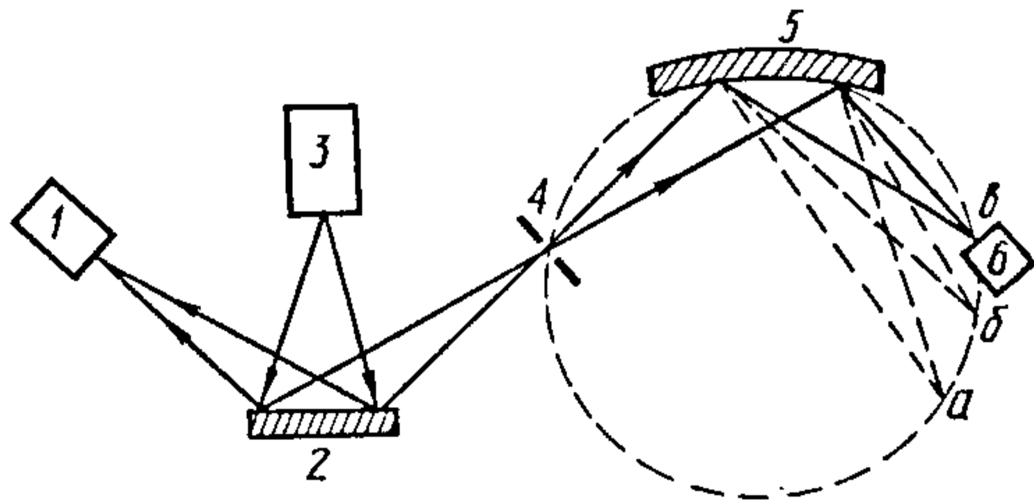
Рыс. 28.4.1. Прынцыповая схема рэнтгенаўскага спектрометра з выгнутым крышталём:
