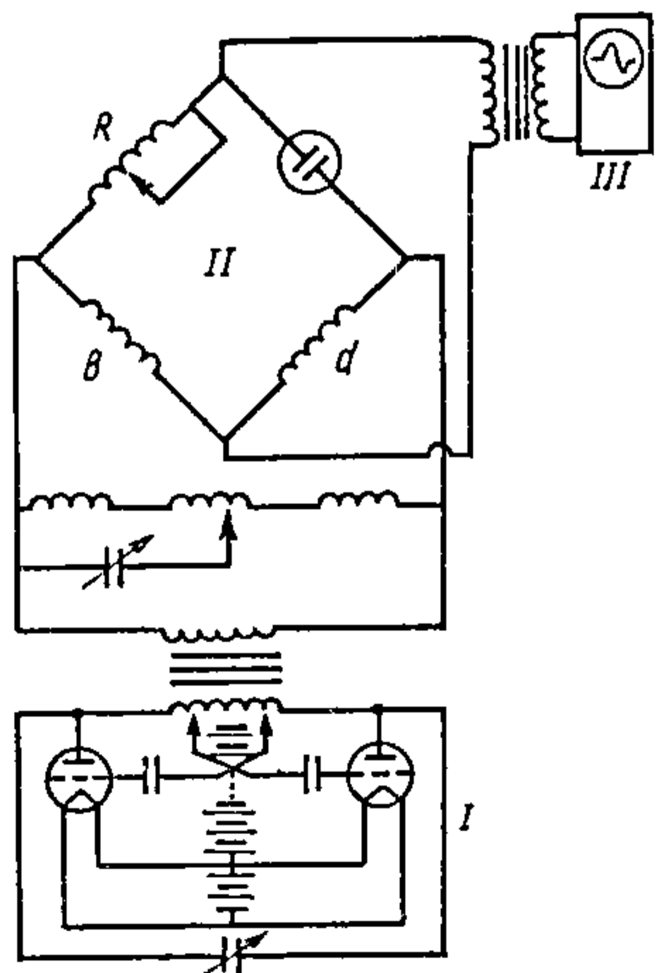
Рыс. 13.1.3. Схема маста пераменнага току (абазначэнні тыя ж, што і на рыс. 13.1. 2).
