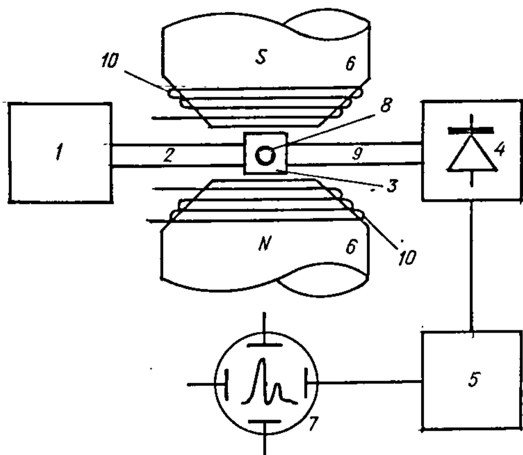
Рыс. 30.3.7. Блок-схема найпрасцейшага радыёспектрометра: 1 — генератар ваганняў ЗВЧ; 2, 9 — хваляводы; 3 — аб'ёмны рэзанатар; 4 — дэтэктар ЗВЧ; 5 — узмацняльнік; 6 — электрамагніт; 7 — рэгіструючы прыбор; 8 — узор у аб'ёмным рэзанатары; 10 — катушка мадуляцыі.
