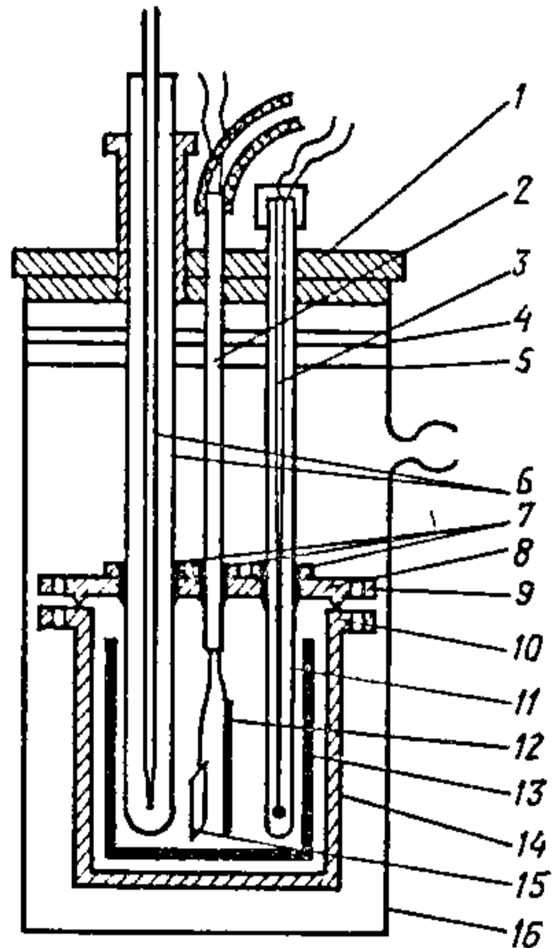
Рыс. 13.3.2. Ячэйка для вымярэння раўнаважных акісляльна-аднаўленчых патэнцыялаў у расплавах:
