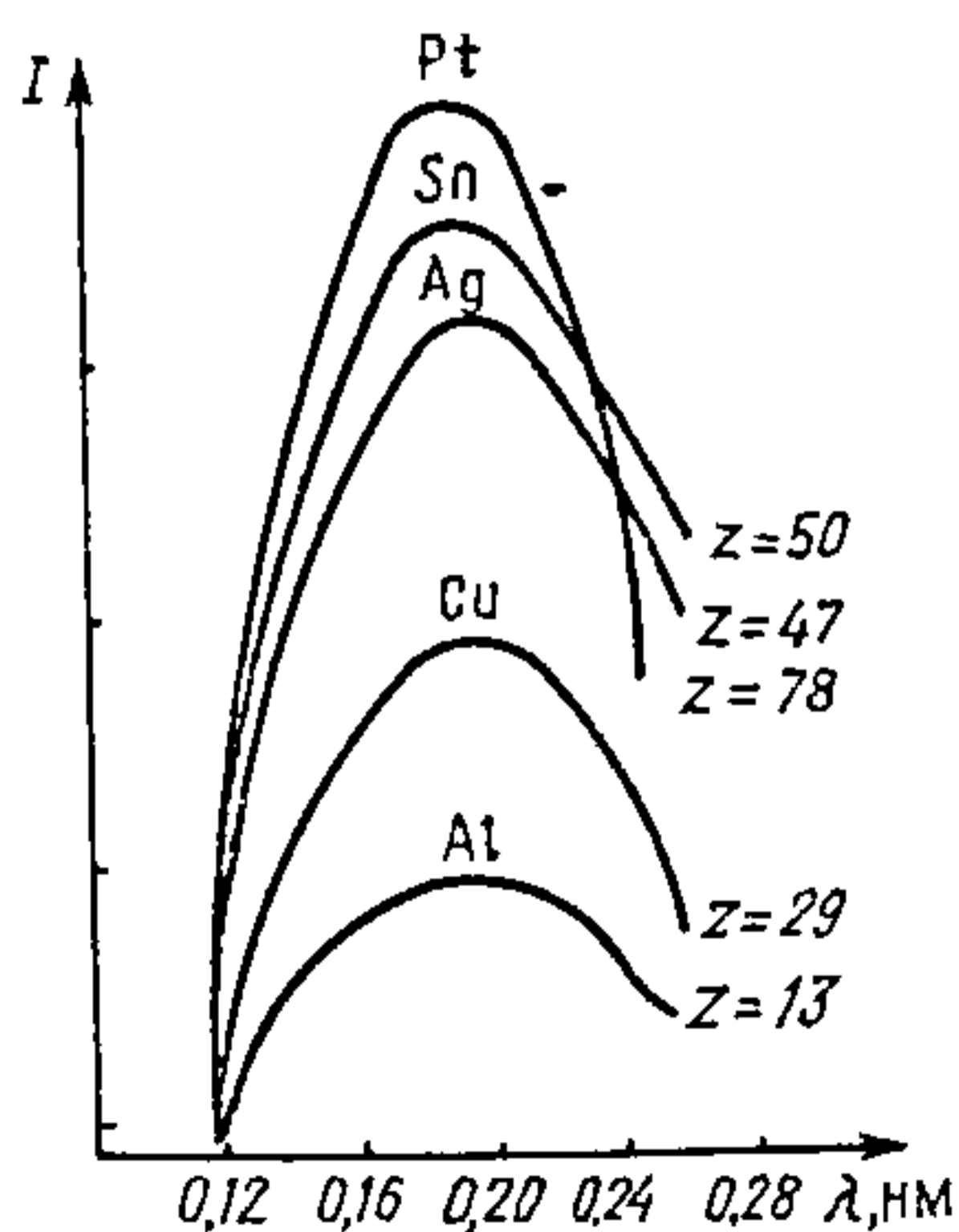
Рыс. 28.1.1. Выгляд залежнасці інтэнсіўнасці суцэльнага спектра тармажэння.
