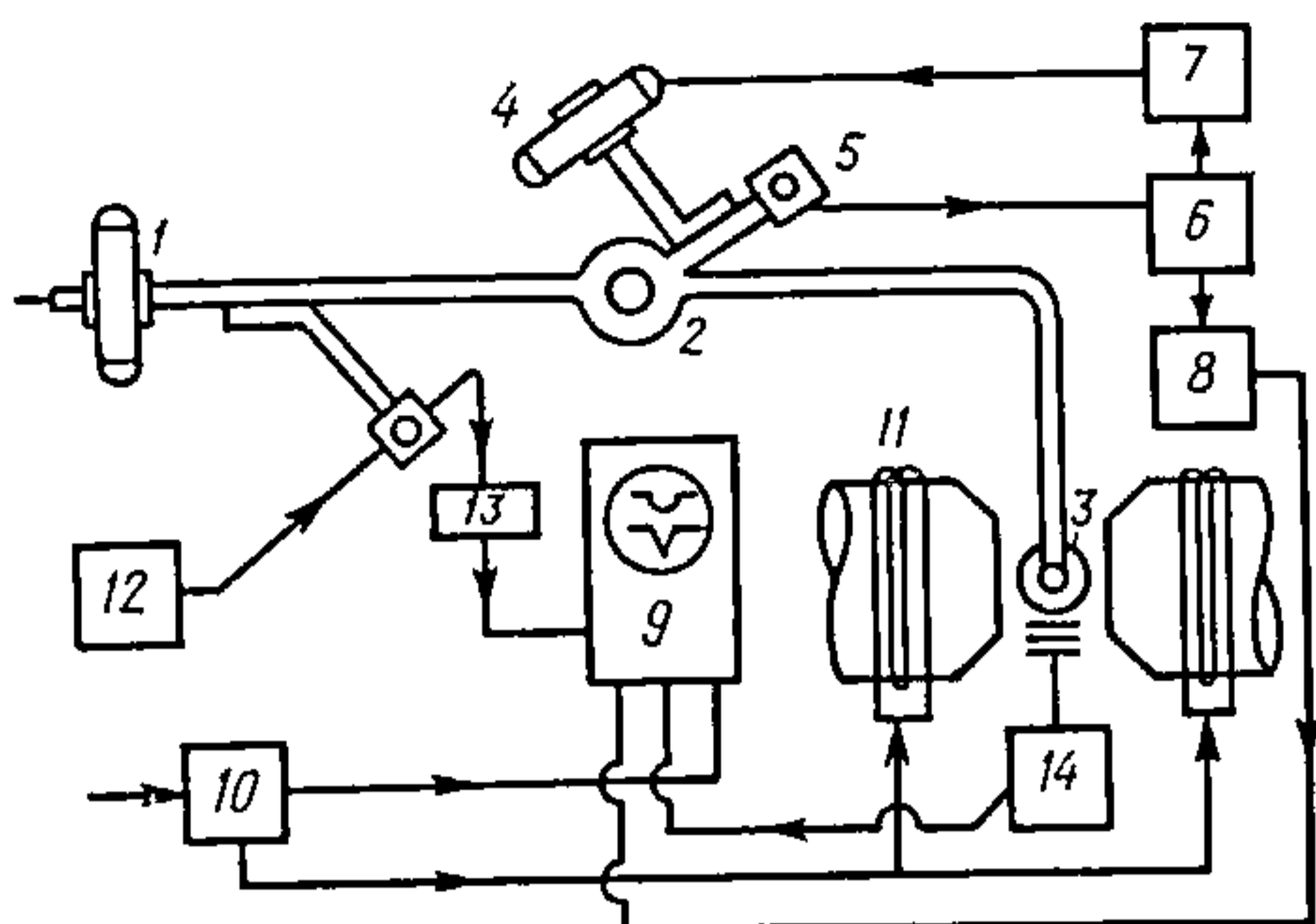
Рыс. 30.3.9. Схема мікрахвалевага спектраскопа, які працуе па супергетэрадзінным метады:
