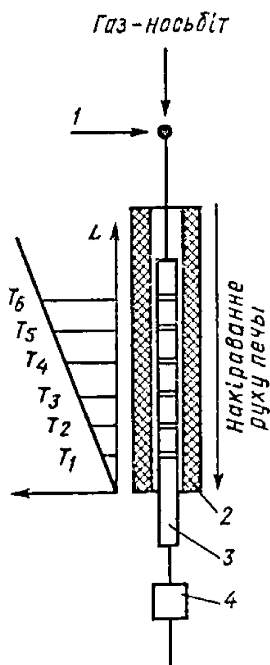
Рыс. 15.1.3. Прынцыповая схема хромаграфічнага раздзялення: 1 — увод пробы; 2 — рухомая электрапеч з градыентам тэмпературы па даўжыні; 3 — адсарбцыйная калонка; 4 — дэтэктар; T = f(L) — размеркаванне тэмпературы ўздоўж пачы, T_1 \dots T_6 — выхадныя тэмпературы кампанентаў раздзяляемай многакампанентнай сумесі (рысачкі на калонцы абазначаюць размяшчэнне зон іх уздоўж калонкі).
