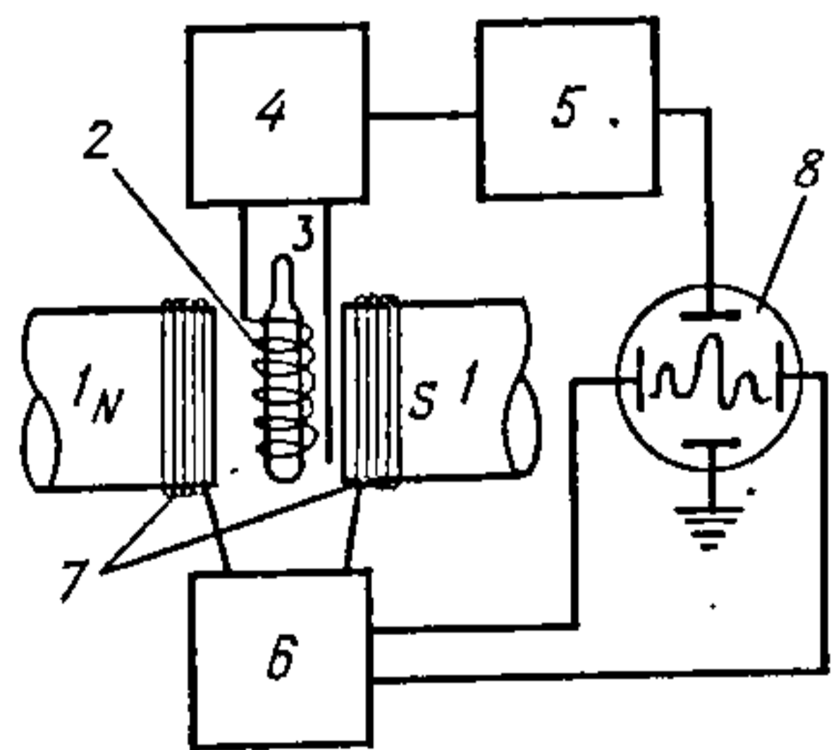
Рыс. 30.4.3. Схематычны відарыс устаноўкі для назірання ЯМР: 1 — магніт; 2 — ВЧ катушка; 3 — ампула з узорам рэчыва; 4 — генератар высокай частаты; 5 — прыёмнік (узмацняльнік і дэтэктар); 6 — генератар магнітнай разгорткі; 7 — катушкі магнітнай разгорткі; 8 — катодны асцылограф.
