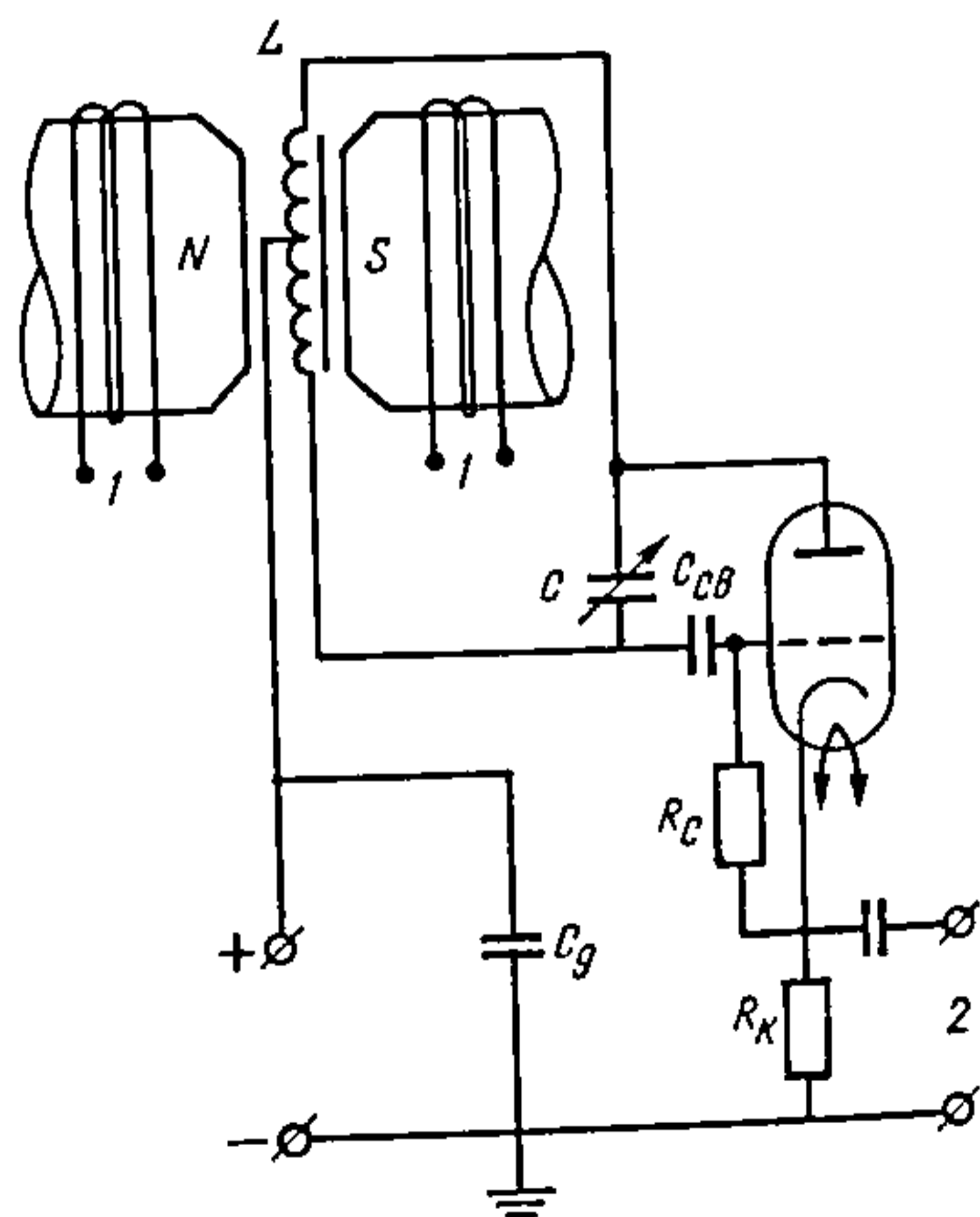
Рыс. 30.3.10. Схема вымярэння сігналу рэзананснага паглынання ў радыёчастотным дыяпазоне: 1 — катушкі мадуляцыі; 2 — выхад да нізкачастотнага ўзмацняльніка.
