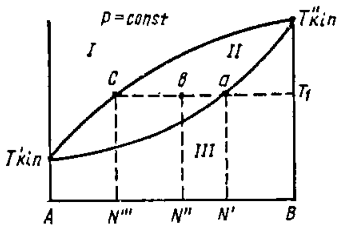
Рис. 8.4.1. Характер дьяграмы T_{кин} = f(N) для раўнавагі вадкасць — пара.
