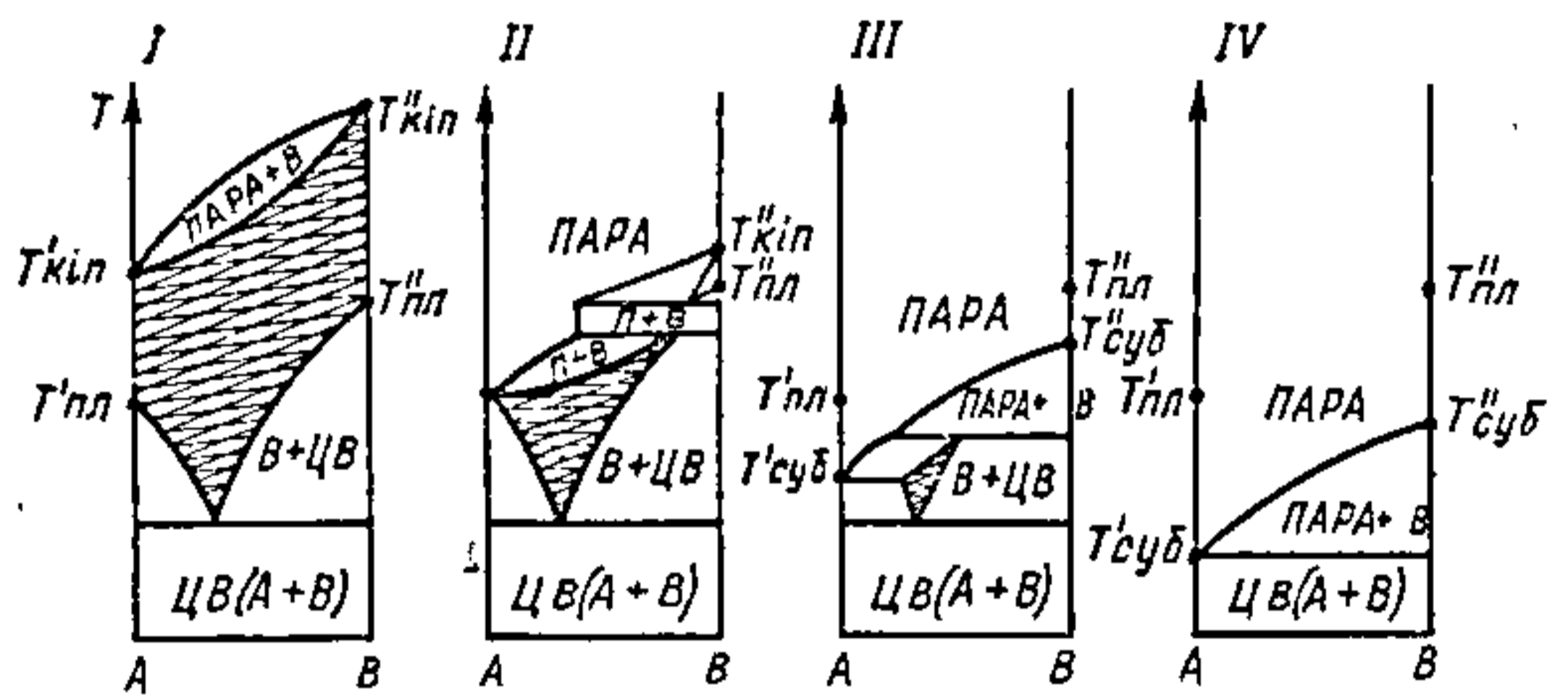
Рыс. 8.4.4. Уплыў ціску на выгляд дыяграмы T = f(N) , якая адлюстроўвае раўнавагу цвёрдае цела — вадкасць — пара ў двухкампанентнай сістэме. Заштрыхавана вобласць вадкага стану: I — p_1 ; II — p_2 < p_1 ; III — p_3 < p_2 ; IV — p_4 < p_3 .
