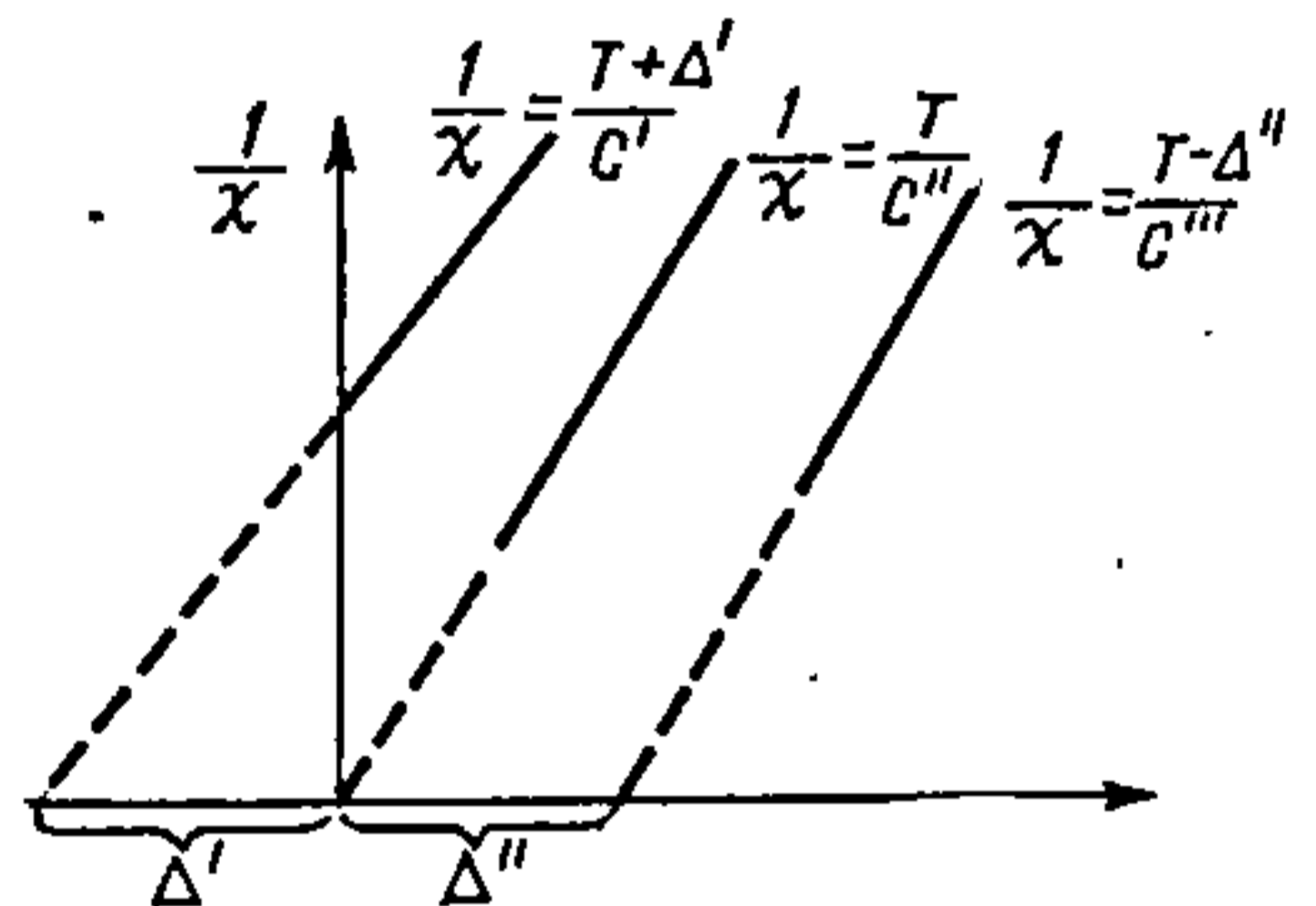
Рыс. 30.1.4. Графік залежнасці 1/\chi = f(T) для разліку магнітных момантаў і значэнняў \Delta .
