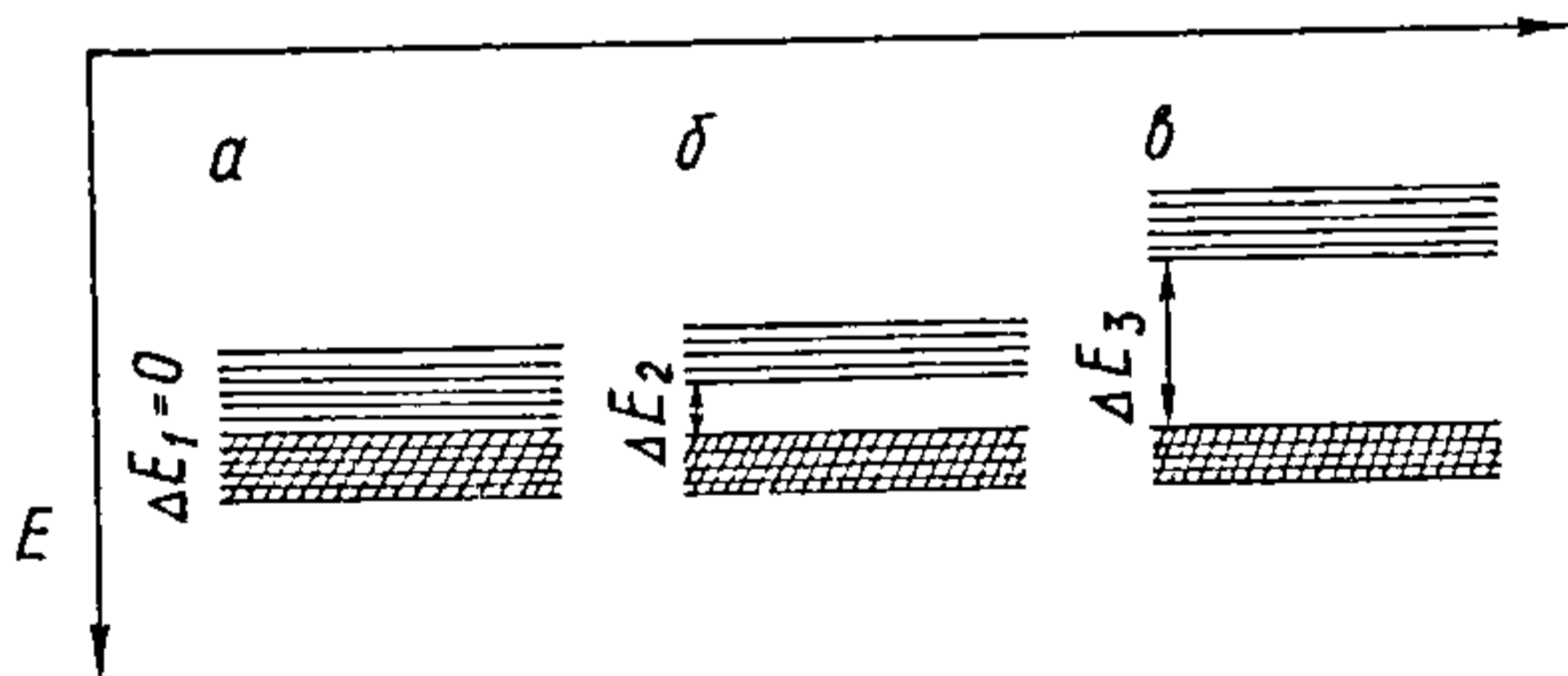
Рыс. 27.3.2. Схема энергетычных зон у атамах металаў, паўправаднікоў і ізалятараў.
