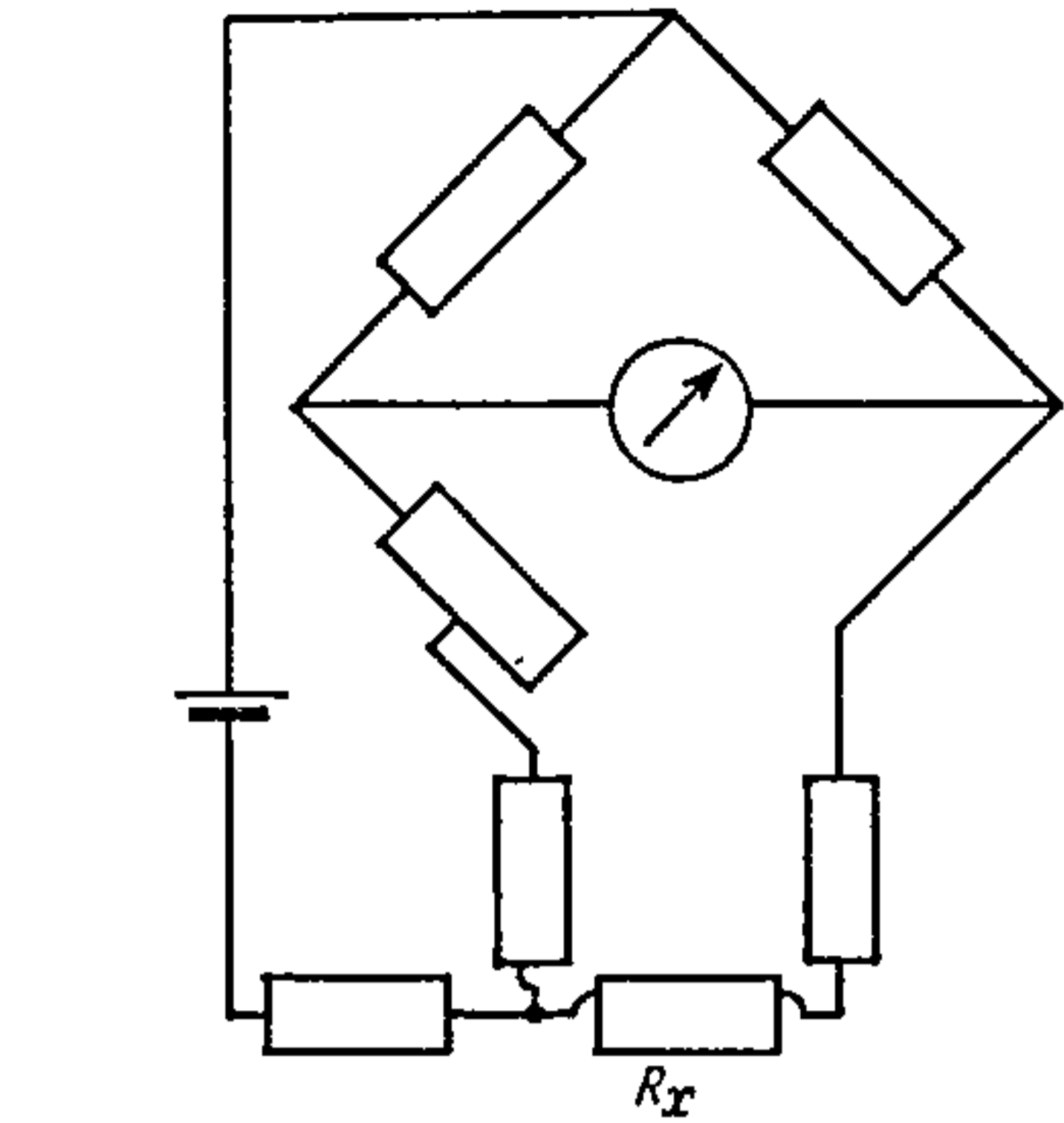
Рыс. 4.11.2. Схема маста для вымярэння супраціўлення драцянога тэрмометра.
