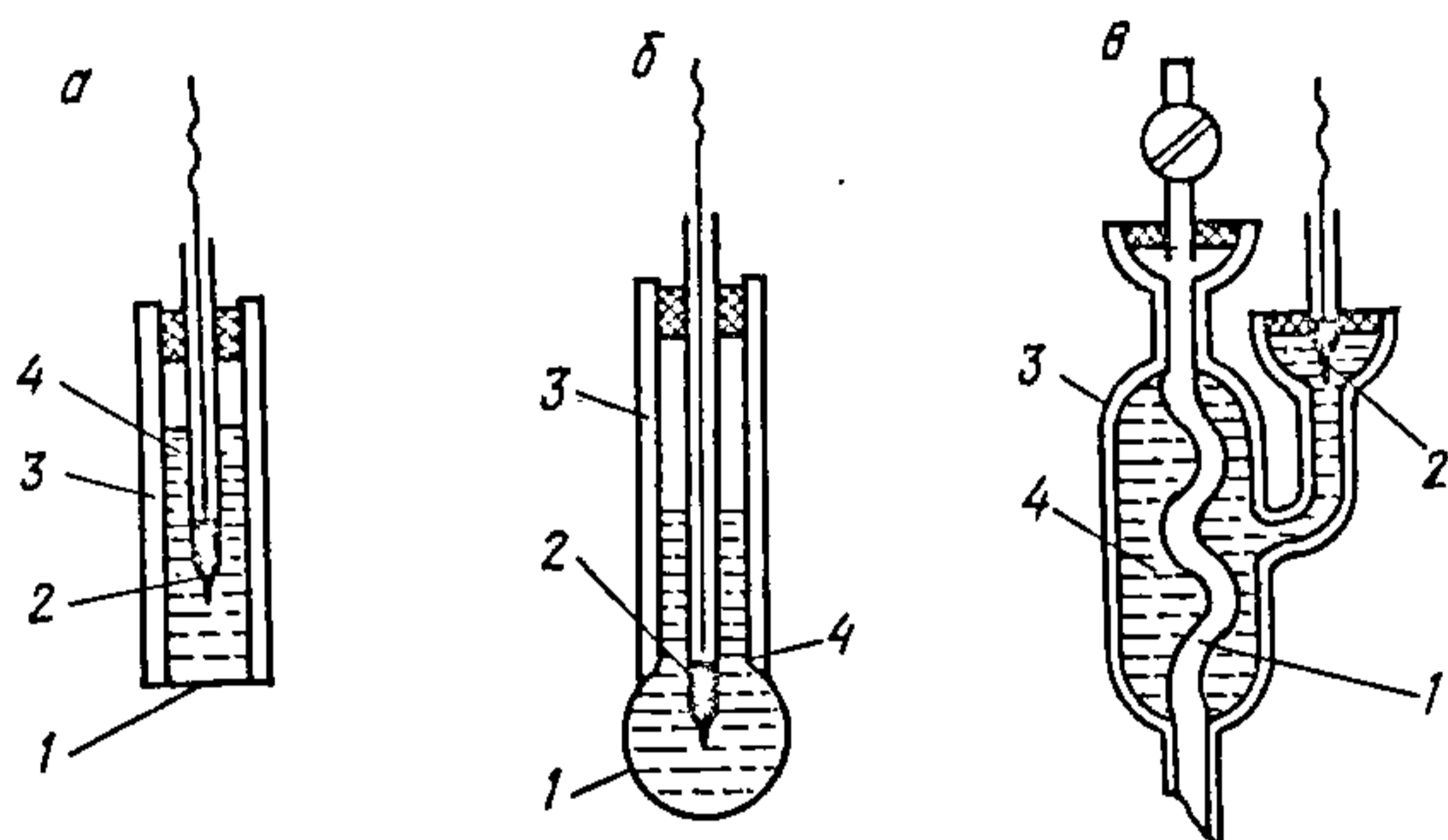
Рыс. 13.2.4. Розныя тыпы шклянога электрода: а — з плоскай шкляной мембранай; б — з шарыкавай; в — з трубчастай; 1 — мембрана са спецыяльнага электроднага шкла; 2 — хлорсярэбраны электрод; 3 — шкляны корпус электрода; 4 — раствор 0,1 \text{ кмоль} \cdot \text{м}^{-3} \text{ HCl} .
