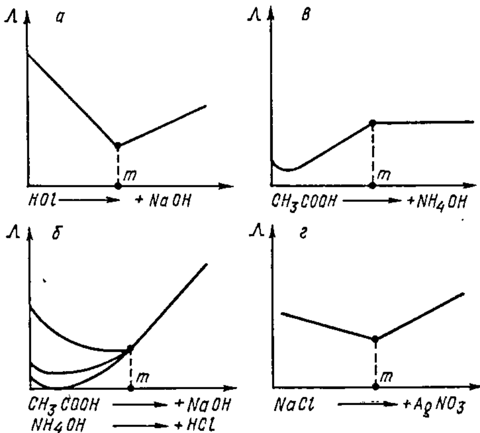
Рыс. 13.1.4. Крывыя кандуктаметрычнага цітравання:
