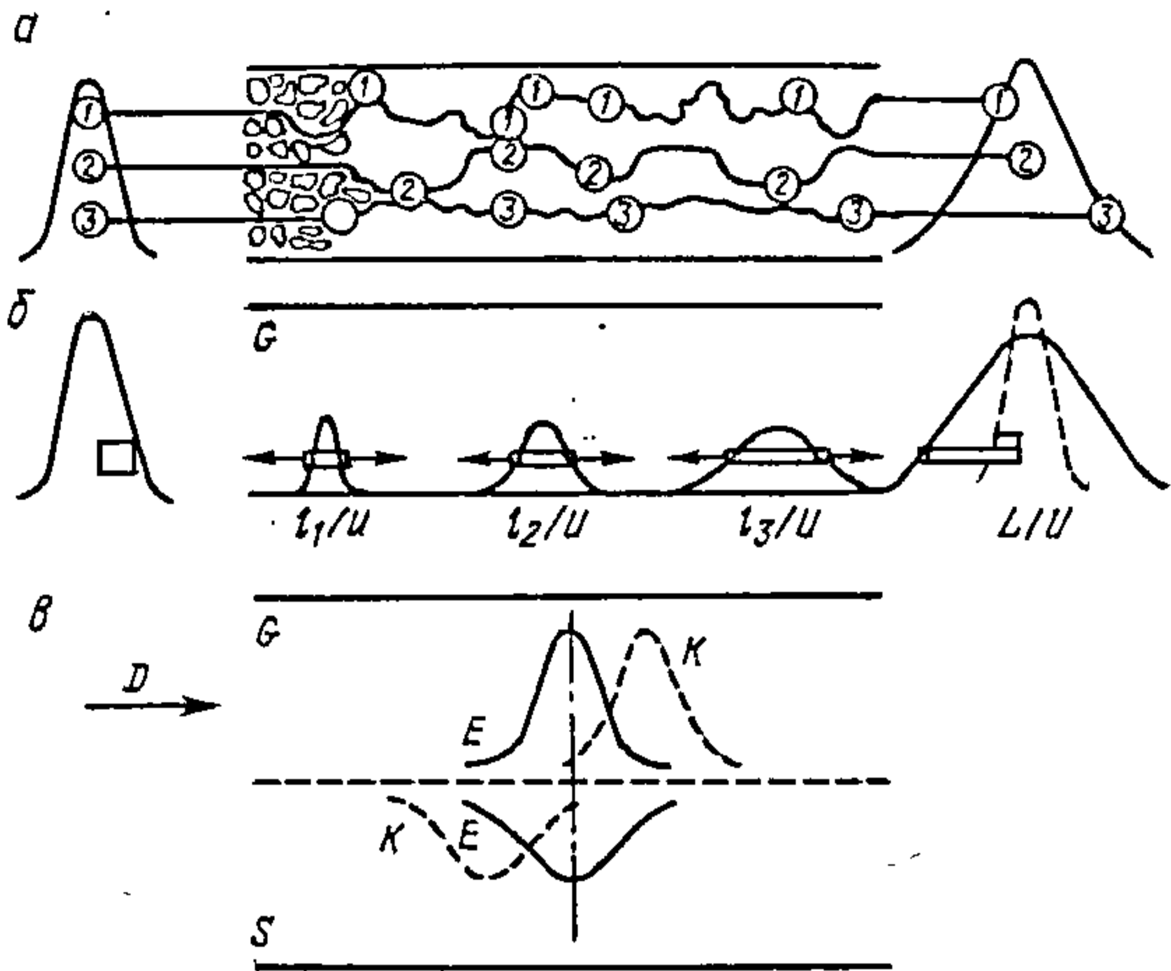
Рыс. 15.2.4. Схема дыфузійных працэсаў у храматаграфіі: a — віхравая дыфузія; b — дыфузія ў газавай фазе; в — міжфазны масаперанос; D — напрамак патоку газавай фазы; E — раўнаважны стан; G — газавая фаза; K — сапраўдная канцэнтрацыя; l — даўжыня калонкі па ардынаце; L — поўная даўжыня калонкі; S — нерухомая фаза; 1-3 — фракцыі аналізуемых злучэнняў.
