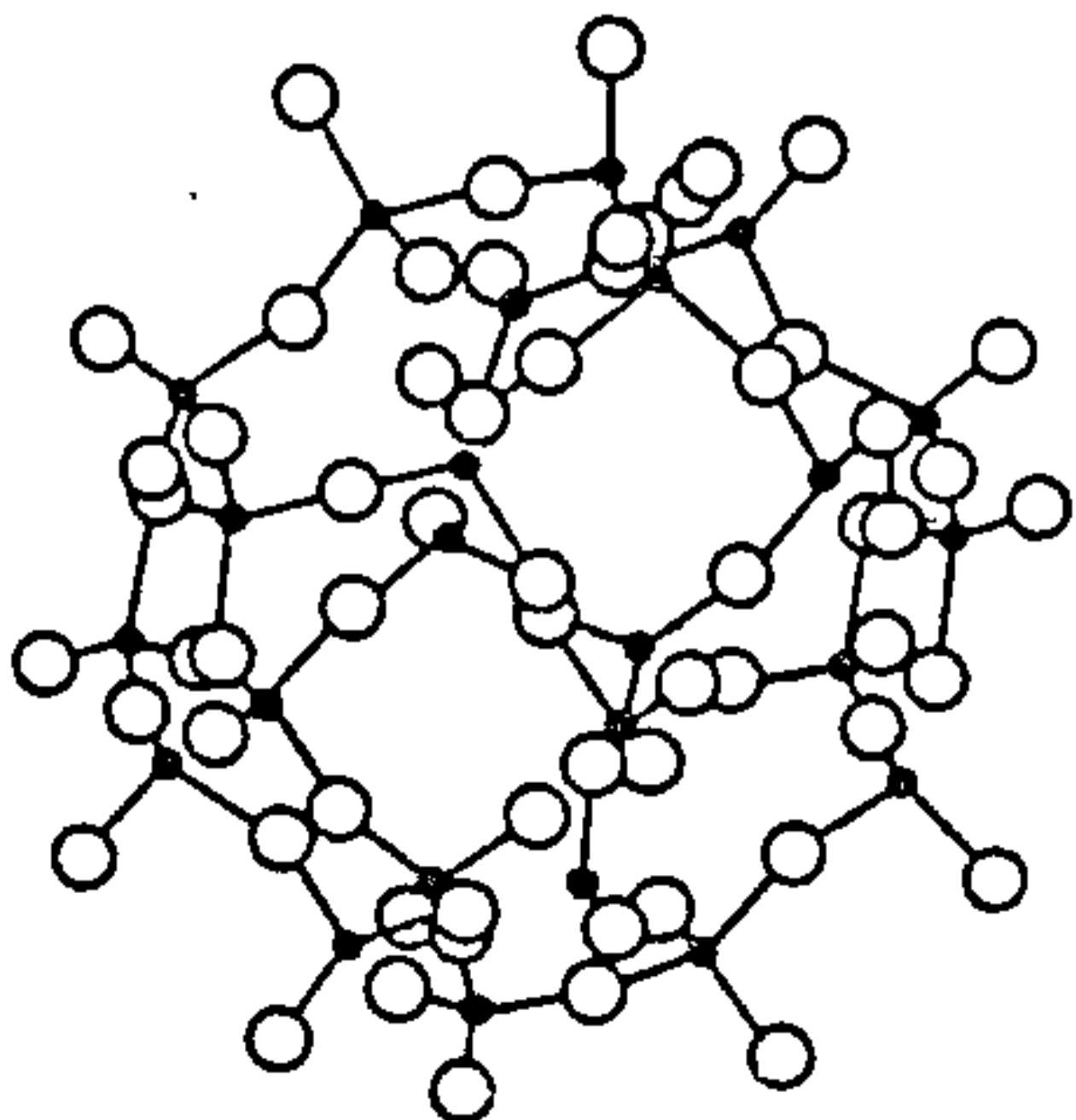
Рыс. 29.4.1. Структура «поласці» цэаліту, утворанай тэтраэдрамі AlO_4 і SiO_4 : светлыя кружкі — атамы кіслароду; чорныя — атомы Si або Al.
