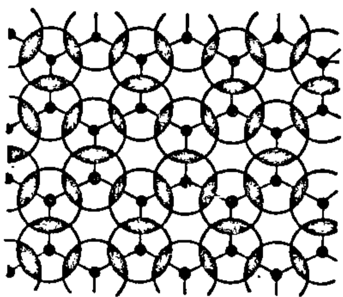
Рыс. 21.5.2. Структура плоскай сеткі крышталю графіту.
