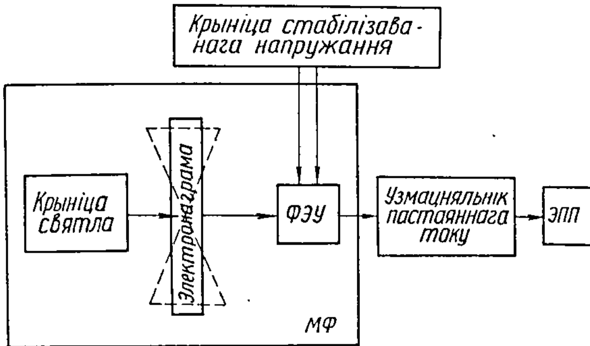
Рыс. 18.4.2. Блок-схема мікрафотаметрычнай устаноўкі.
