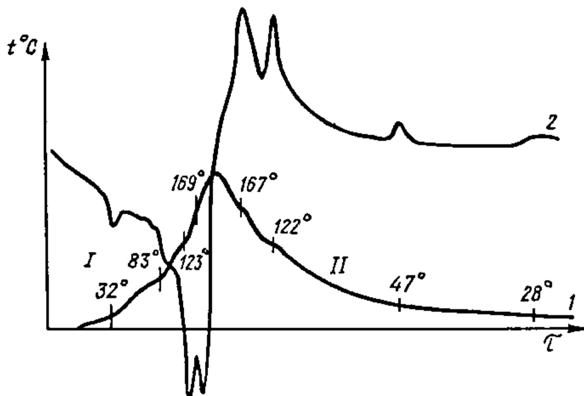
Рыс. 7.9.1. Крывыя нагрэву (I) і ахаладжэння (II) \text{NH}_4\text{NO}_3 , атрыманыя пры дапамозе прастай (1) і дыферэнцыяльнай (2) тэрмапар.
