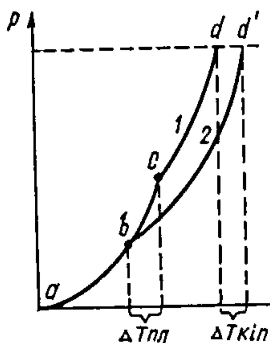
Рыс. 8.2.1. Залежнасць p=f(T) для растваральніка A і раствора \{A+B\} : a, b, c — наяўнасць у сістэме індыўідуальных крышталёў растваральніка; c, d — чысты растваральнік N_d у вадкім стане; b, d' — вадкі раствор.
