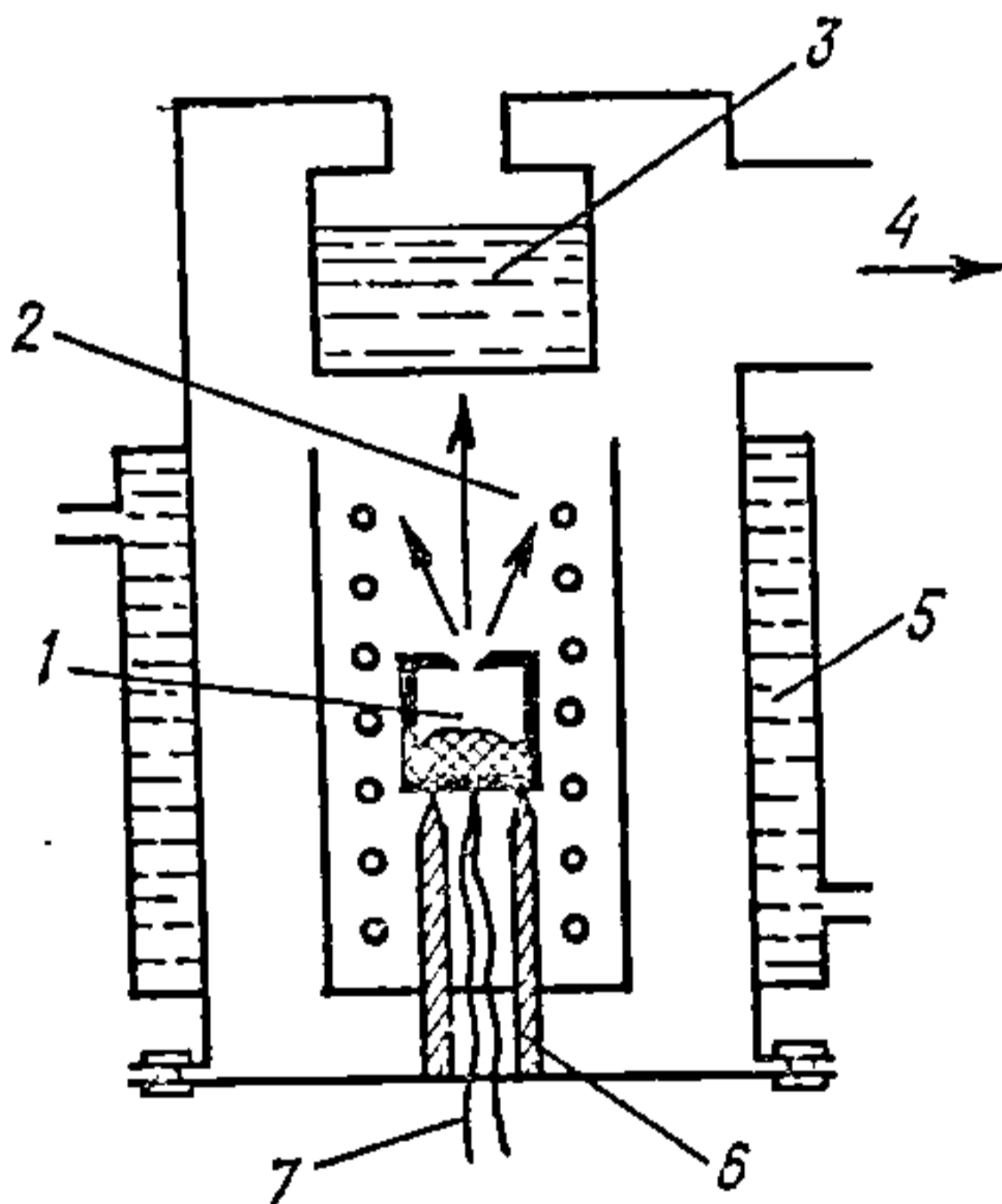
Рыс. 6.5.4. Схема прыбора, што працуе па метадзе Кнудсена:
