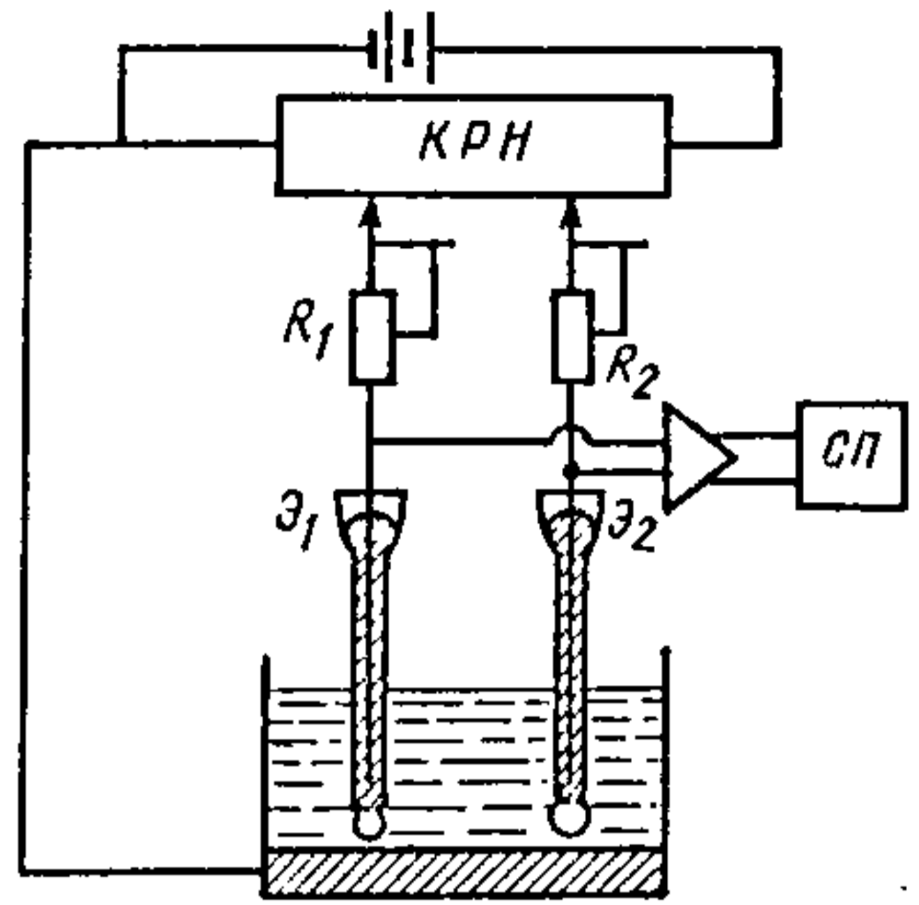
Рис. 13.6.2. Схема диференціальнонага палярографа пастаяннага току:
