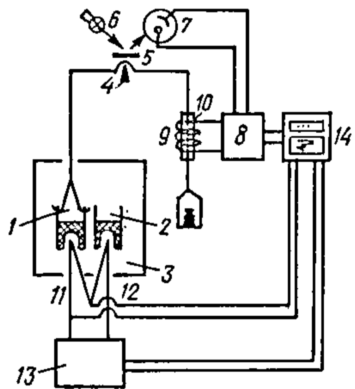
Рыс. 7.11.4. Схема тэрмагравіметрычнай устаноўкі:
