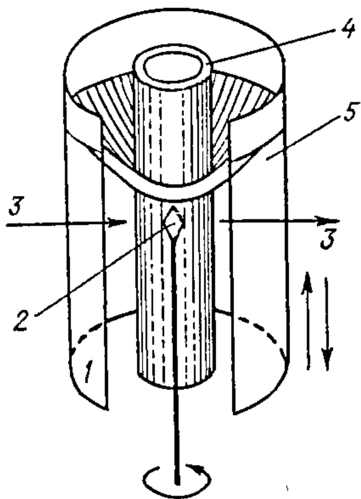
Рис. 28.2.4. Схема рентгенаганіометра Вайсенберга:
