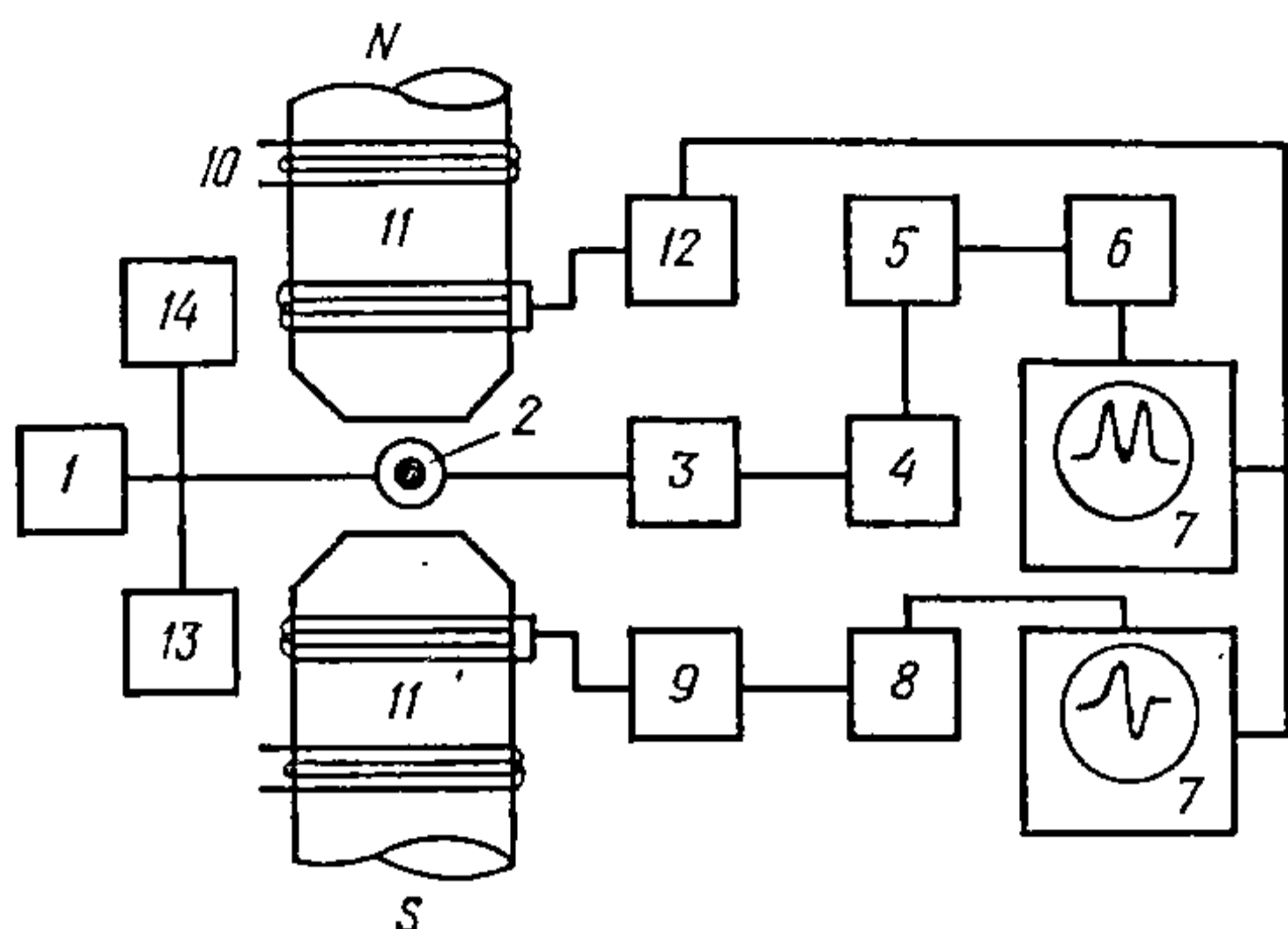
Рис. 30.3.8. Схема мікрахвалевага спектраскопа з двойной мадуляцыяй поля:
