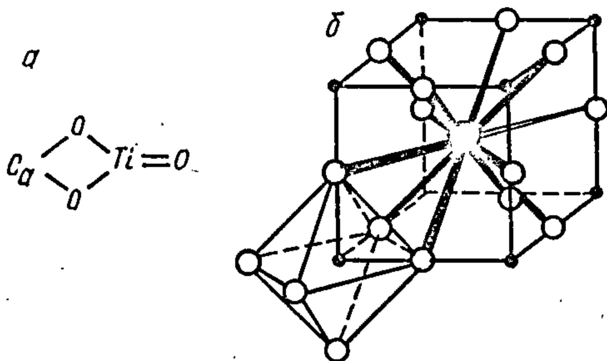
Рис. 26.1.2. Фрагмент (ячейка) кристалічної ґратки мінералу пераїтиту \text{CaTiO}_3 :
