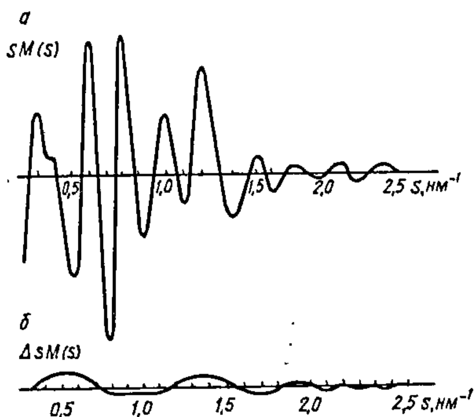
Рыс. 18.5.9. Эксперыментальная кривая sM малекулы \text{WOBr}_4 , удакладненая метадам найменшых квадратаў у супастаўленні sM_{\text{тэар}}(s) з sM_{\text{эксп}}(s) .
