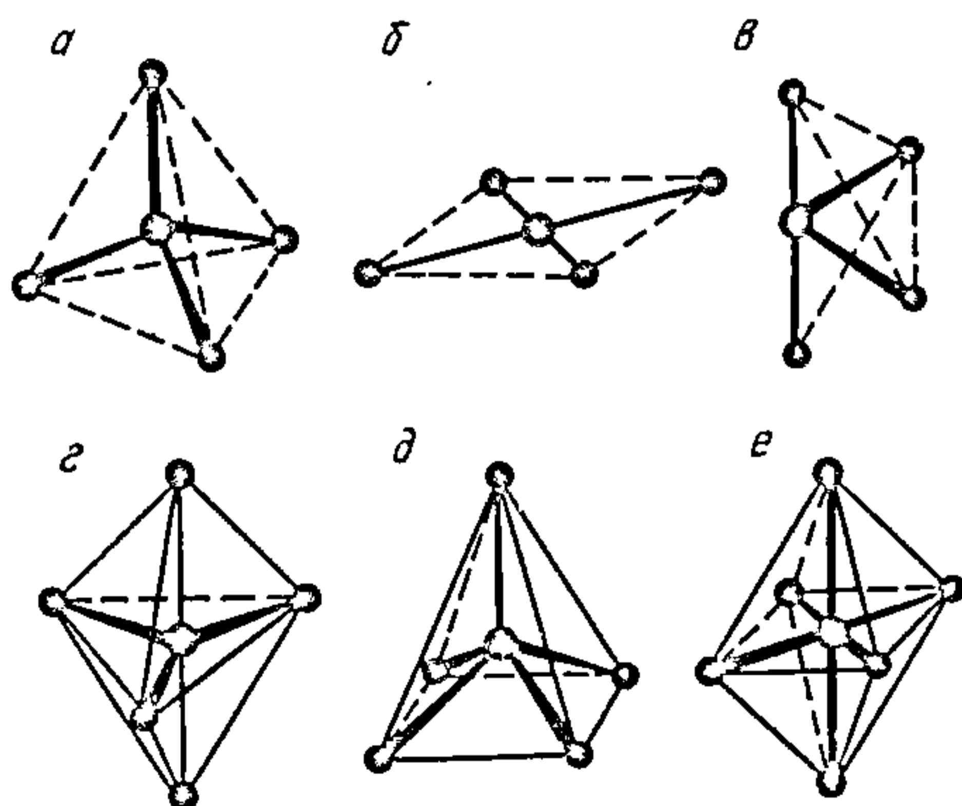
Рыс. 22.1.1. Найбольш характэрныя формы каардынацыі лігандаў каля атама (іона)-комплексаўтваральніка: а — тэтраэдрычная ( sp^3 -гібрыдызацыя); б — плоскаквadratная ( sd^3 -гібрыдызацыя); в — седлападобная (гіперсувязь — 1); г — трыганальна-біпірамідальная ( sp^2 + sp -гібрыдызацыя); д — тэтраганальна-пірамідальная; е — актаэдрычная ( d^2sp^3 -гібрыдызацыя).
