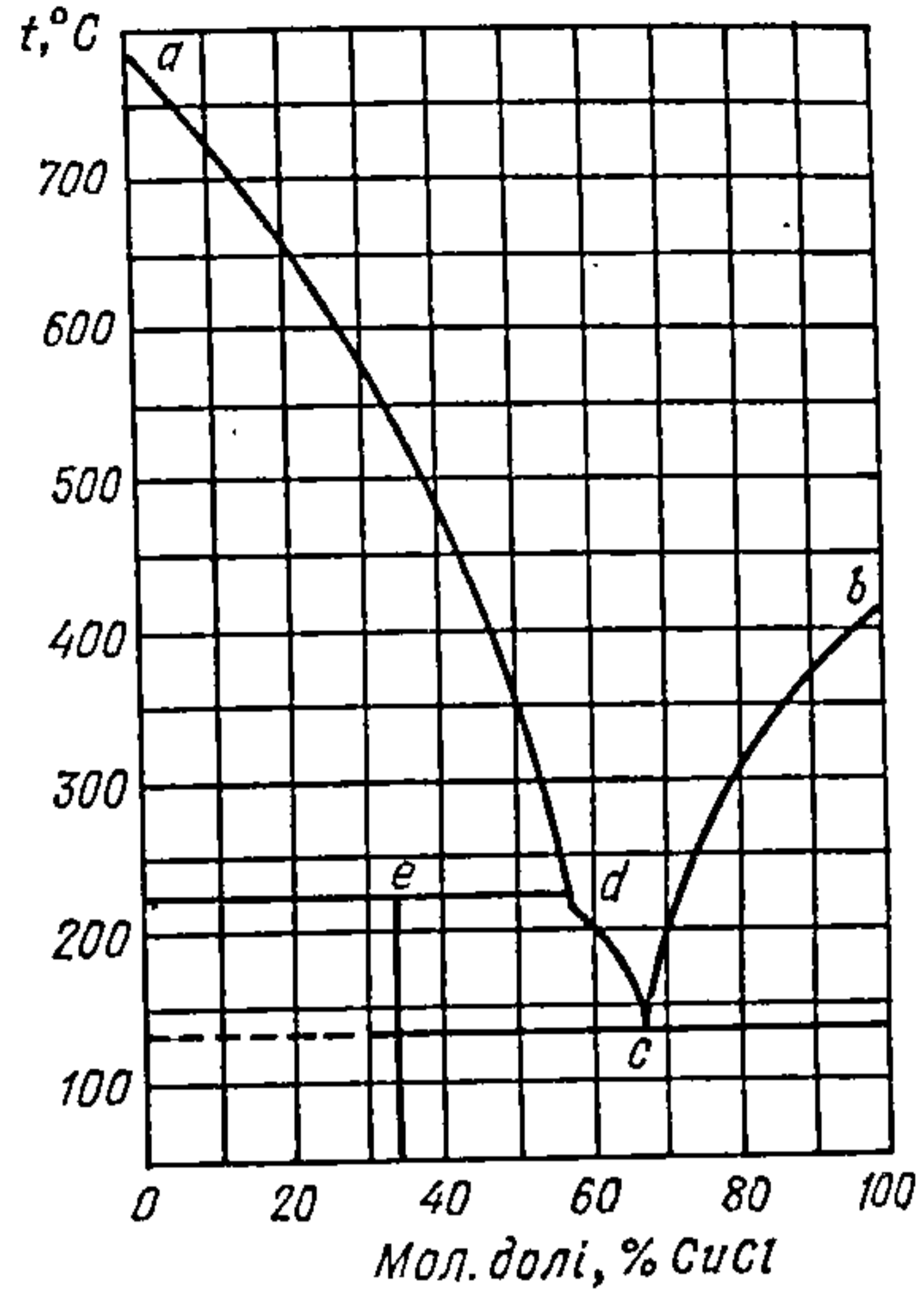
\text{CuCl} - \text{KCl}
