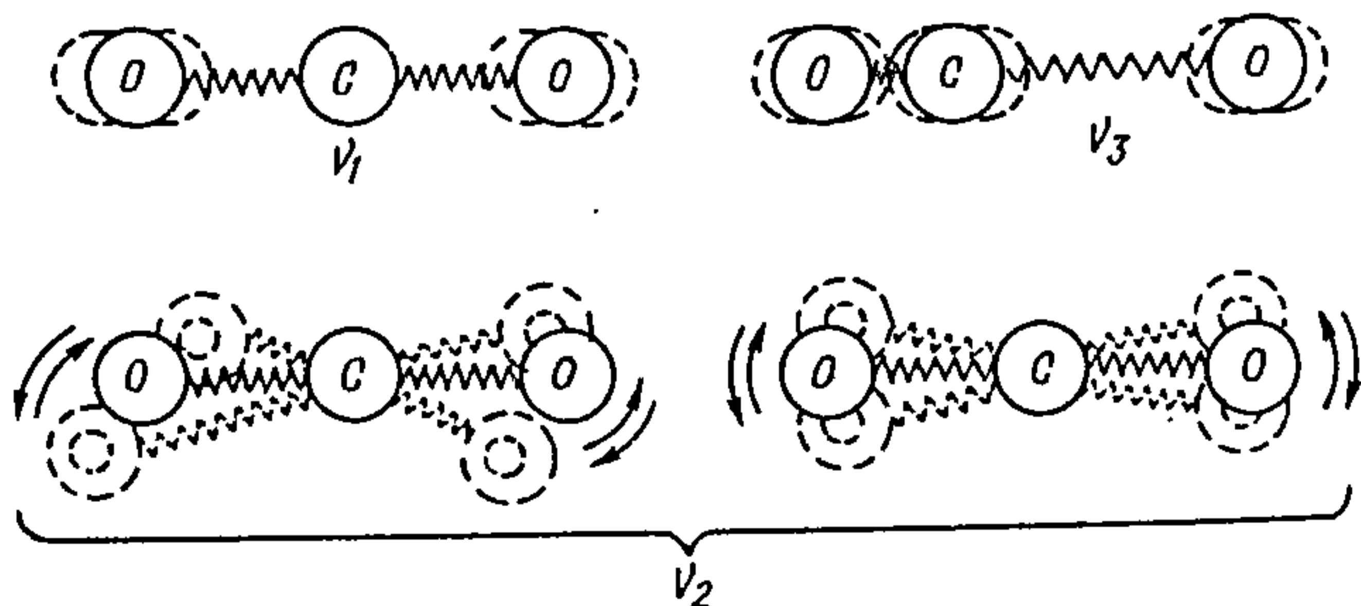
Рис. 25.2.4. Чатыры нормальныя ваганні молекулы \text{CO}_2 : \nu_1 — симетрычнае валентнае з частотой 1340 \text{ см}^{-1} ; \nu_3 — антисиметрычнае валентнае з частотой 2349 \text{ см}^{-1} ; \nu_2 — два дэформацыйных выраджаных з частотой 667 \text{ см}^{-1} .
