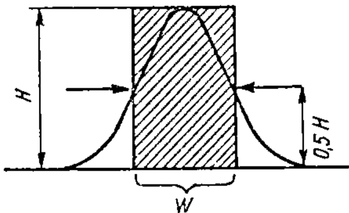
Рыс. 15.2.10. Вымярэнне плошчы храматаграфічнага піка шляхам звядзення плошчы трохвугольніка да плошчы прамавугольніка (гл. заштрыханую вобласць): H — вышыня трохвугольніка (і прамавугольніка); W — шырыня прамавугольніка.
