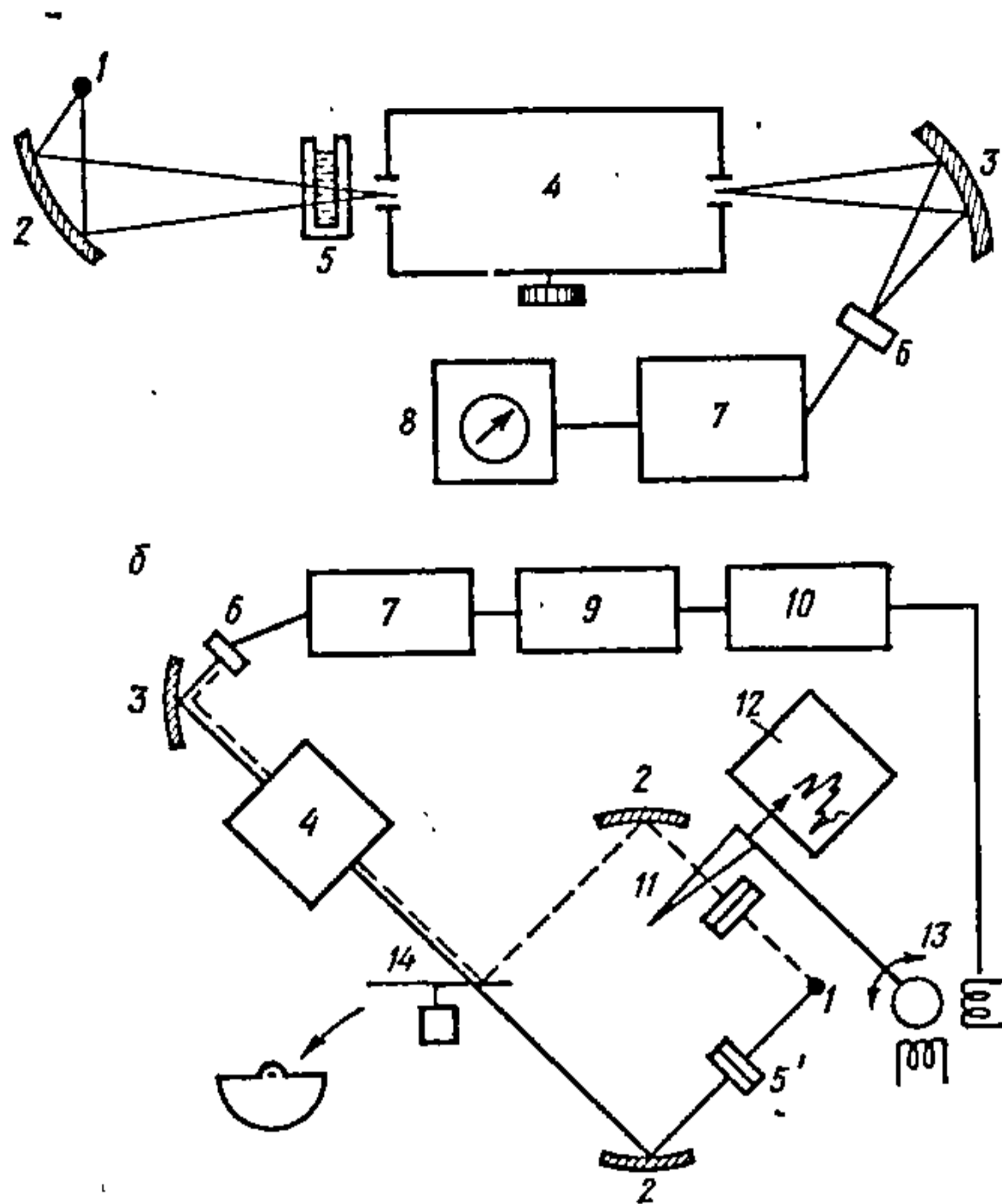
Рис. 25.7.1. Схематичні відарис ІЧ-спектрометраў аднапрамянёвага (а) і двухпрамянёвага (б) тыпаў:
