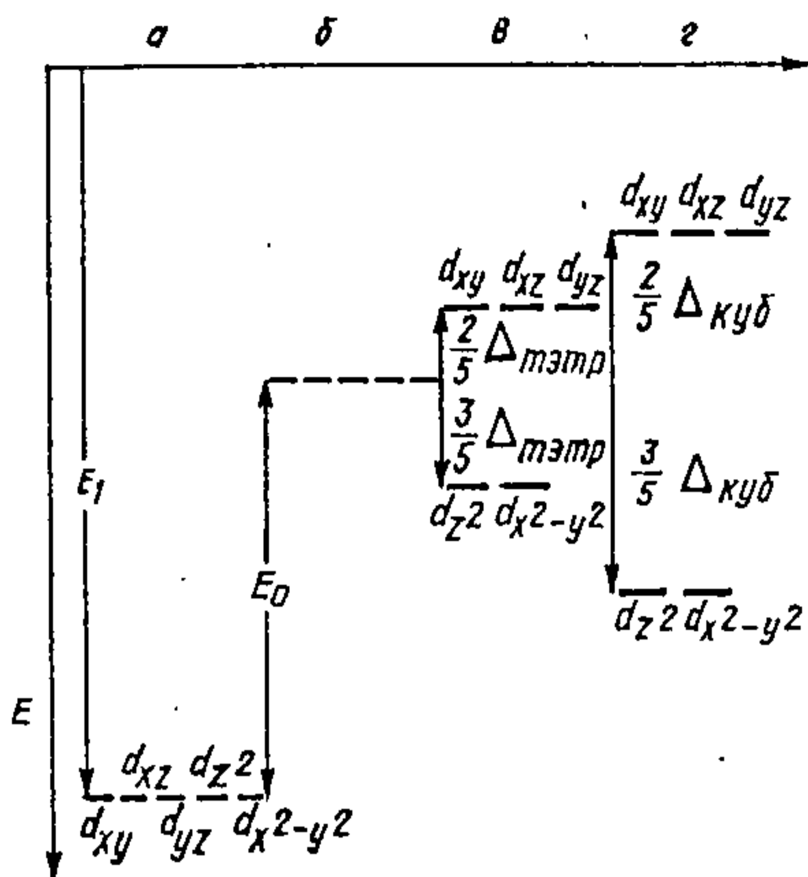
Рыс. 22.3.9. Параўнальная характарыстыка расщеплення d -тэрмаў цэнтральнага іона ў полі лігандаў:
