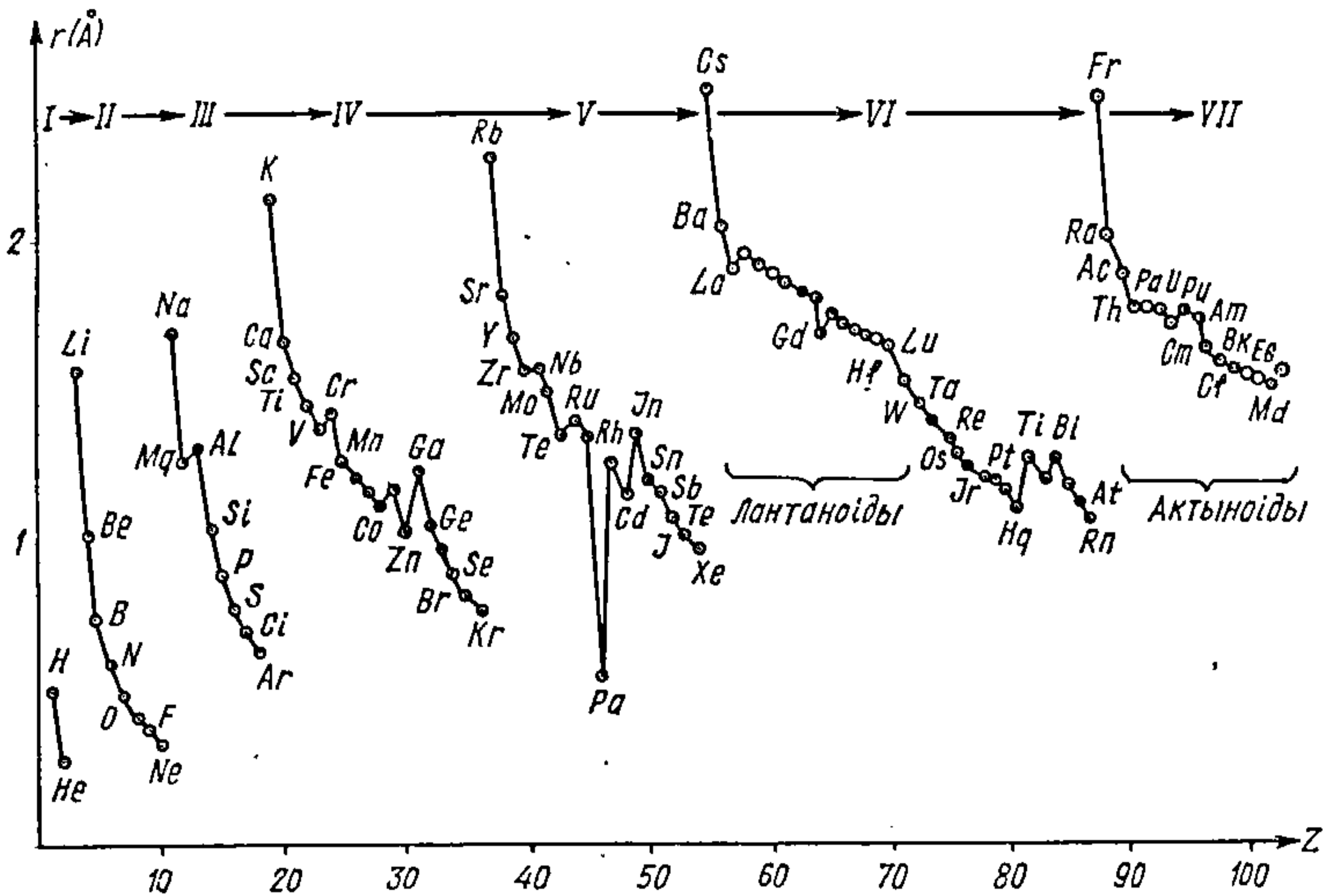
Рис. 19.3.1. Залежнась радуса атамаў ад зараду ядра.
