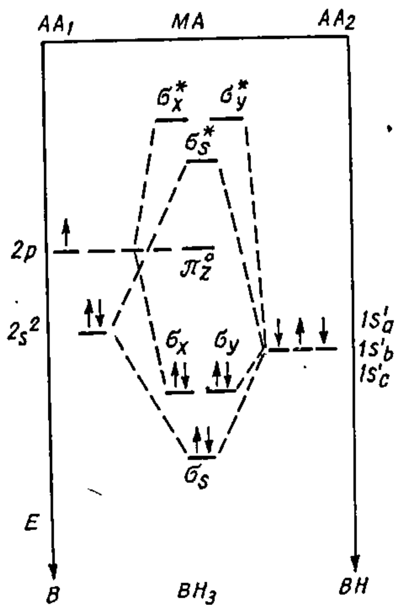
Рыс. 24.3.2. Энергетычная дыяграма МА манамернай малекулы \text{BH}_3 .
