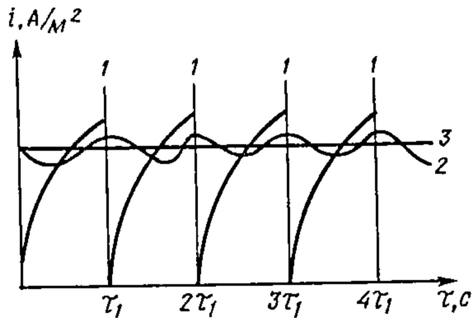
Рыс. 13.4.4. Залежнасць дыфузійнага току ад часу для ртутнага кропельнага электрода:
