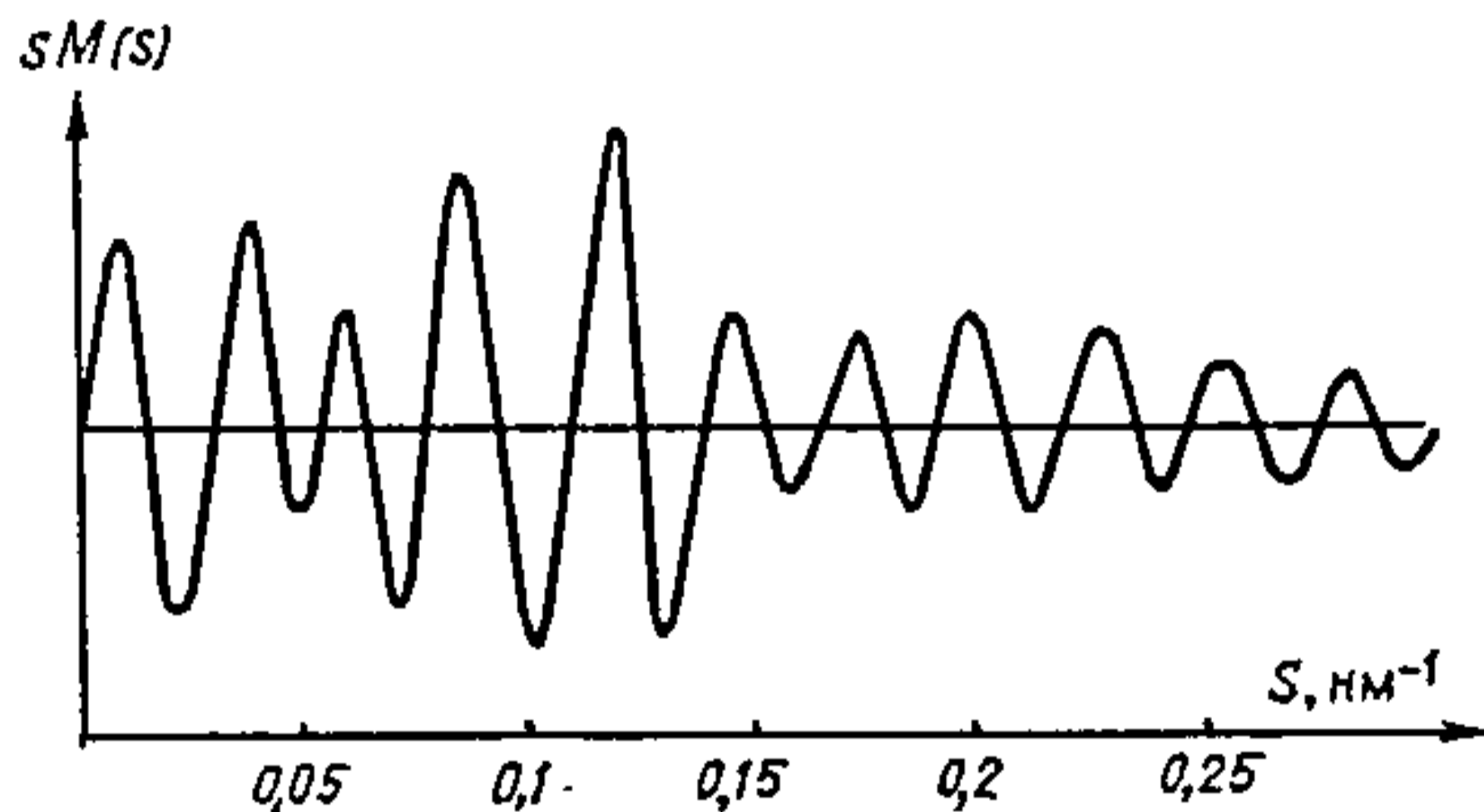
Рис. 18.5.6. Кривая sM_{\text{эксп}}(s) для малекулы \text{WOBr}_4 .
