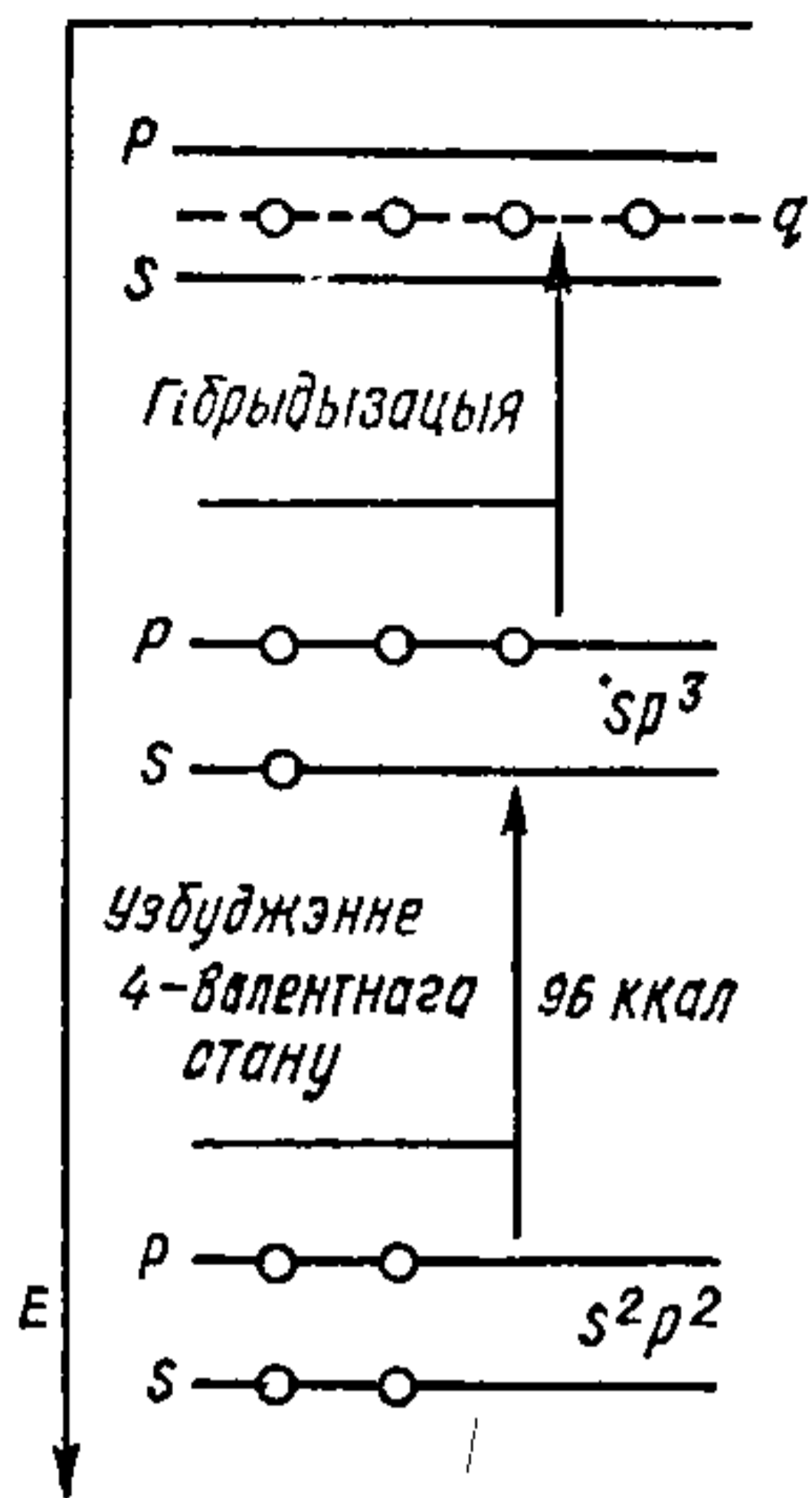
Рыс. 21.3.1. Схема ўзбуджэння гібрыднага стану арбіталей у атаме вугляроду.
