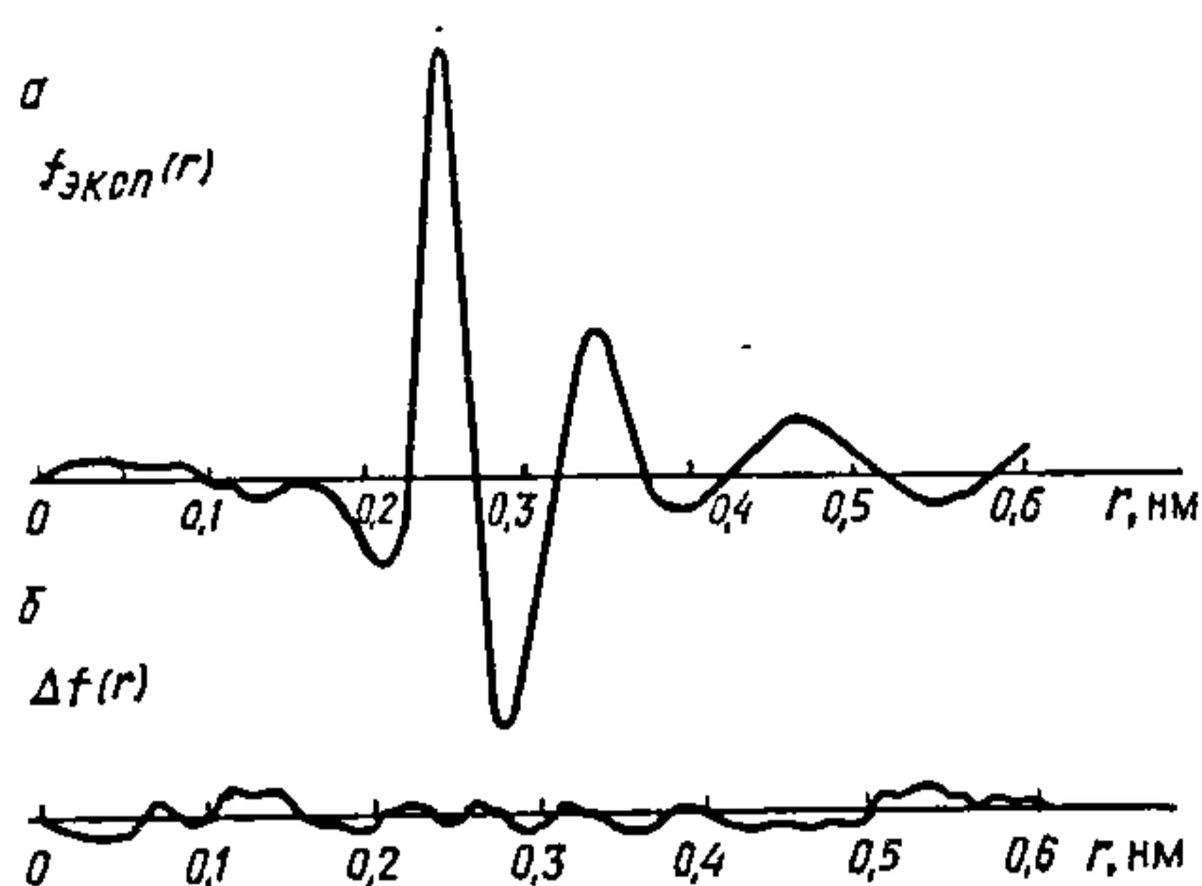
Рыс. 18.5.7. Кривая радыяльнага размеркавання f_{\text{эксп}}(r) для малекулы \text{WOBr}_4 .
