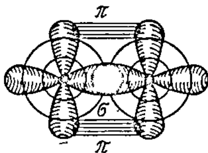
Рыс. 21.1.5. Схема малекулы \text{C}_2 .
