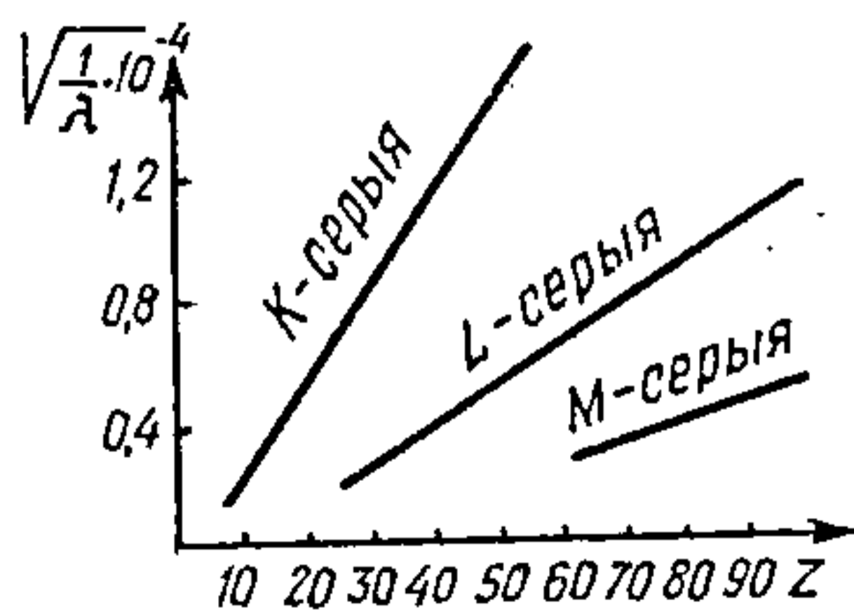
Рыс. 28.1.2. Відарыс да закону Г. Мозлі.
