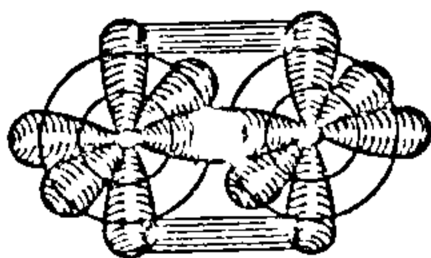
Рыс. 21.1.7. Схема малекулы O_2 .
