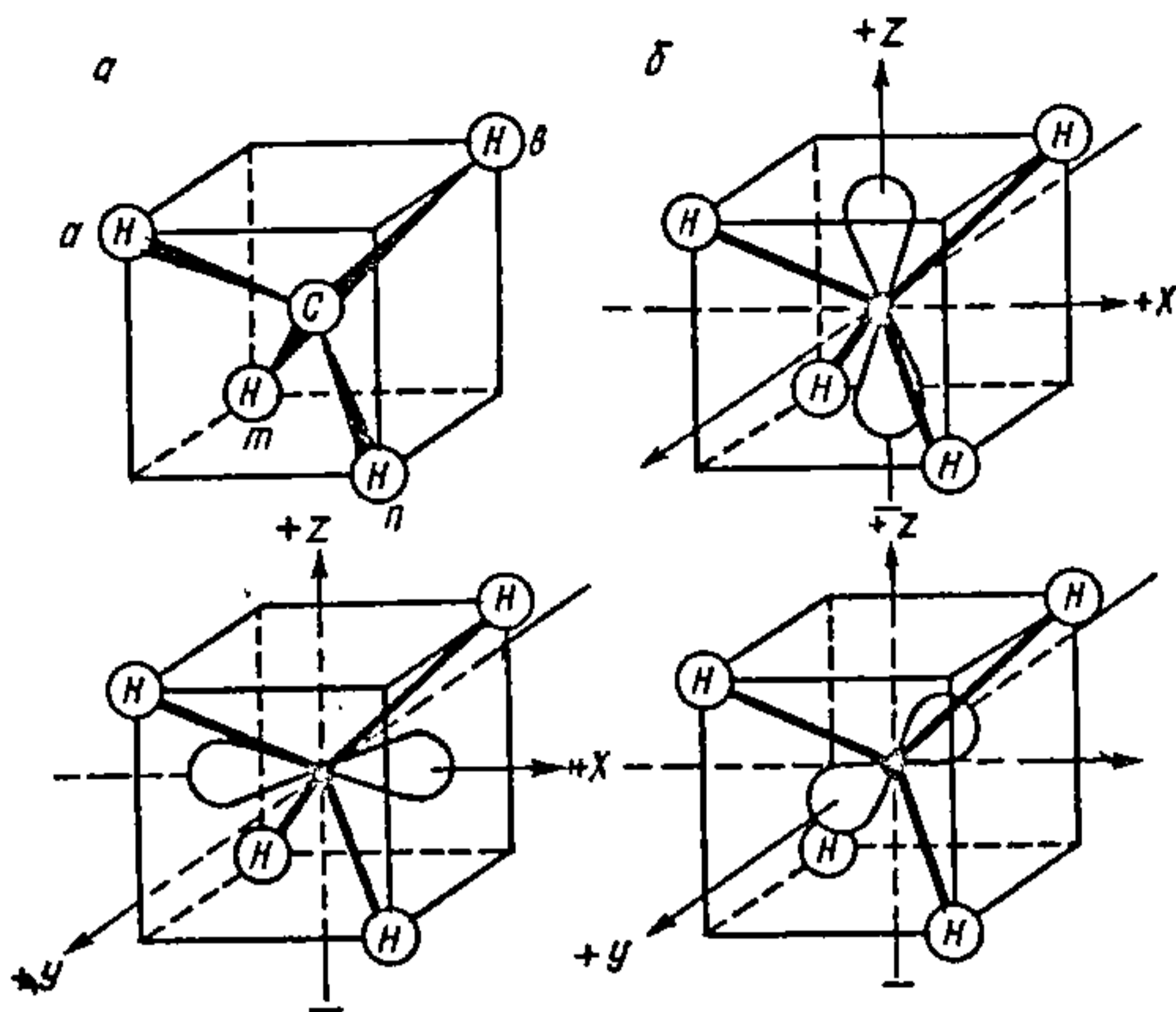
Рис. 24.4.1. Схема зближення чотырох атомаў вадароду з атомам вугляроду пры ўтварэнні малекулы \text{CH}_4 .
