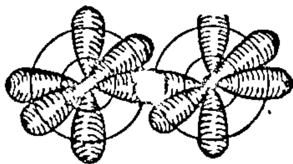
Рыс. 21.1.8. Схема малекулы F_2 .
