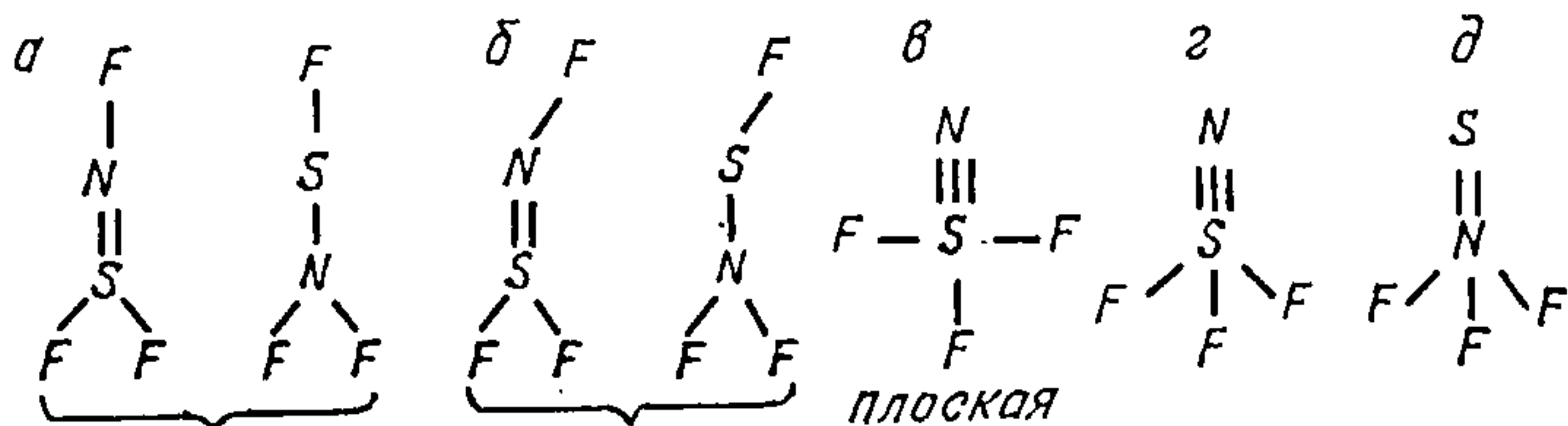
Рис. 25.7.5. Допускаемые структуры \text{NSF}_3 .
