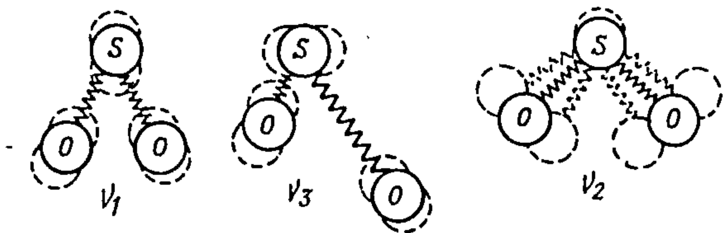
Рис. 25.2.3. Три нормальні ваганні молекули \text{SO}_2 : \nu_1 — симетричне валентне з частотою 1151 \text{ см}^{-1} ; \nu_3 — антисиметричне валентне з частотою 1361 \text{ см}^{-1} ; \nu_2 — деформаційне з частотою 519 \text{ см}^{-1} .
