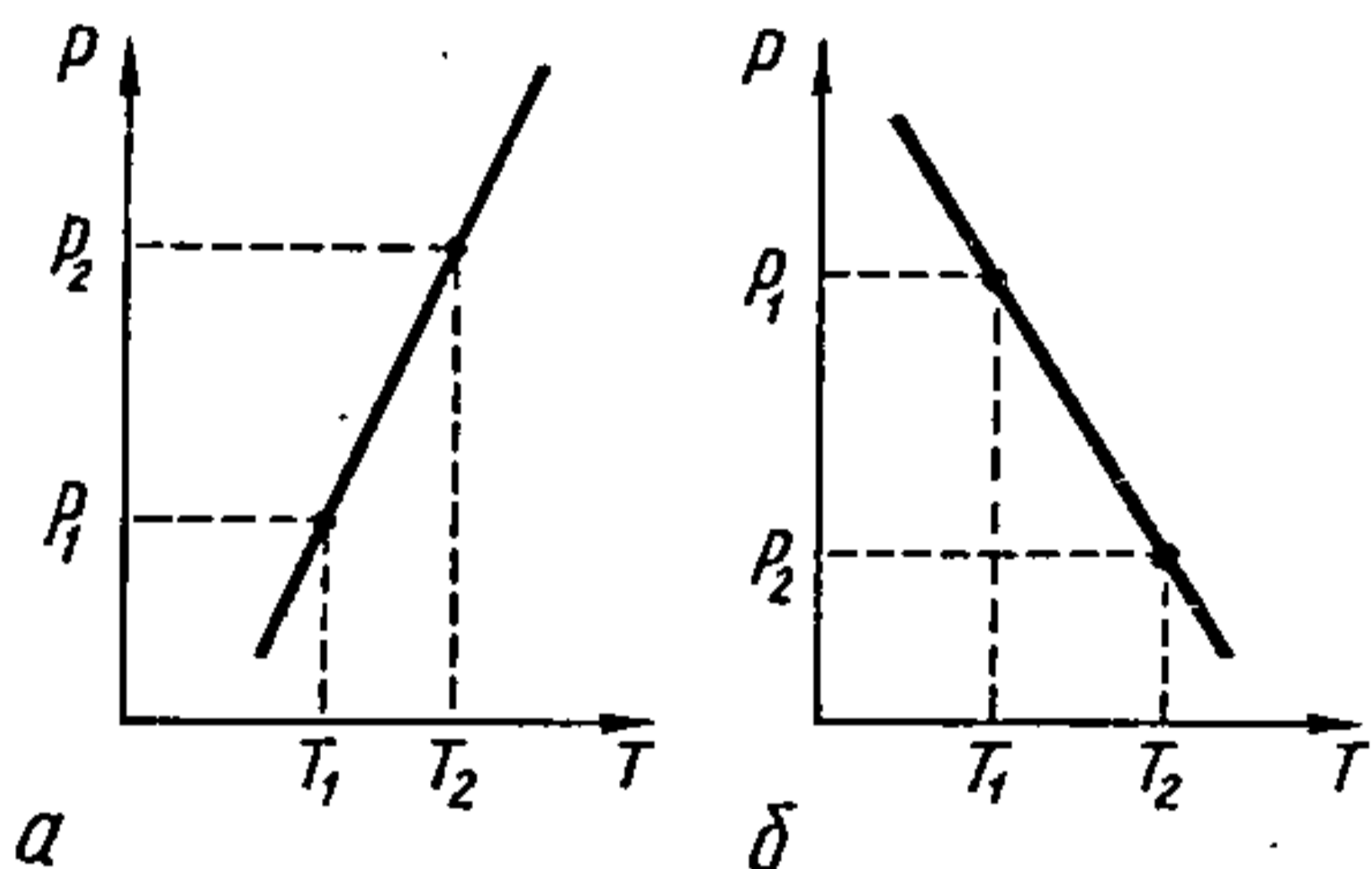
Рыс. 7.2.2. Змяненне характару нахілу лініі залежнасці p=f(T) пры розных суадносінах удзельных аб'ёмаў цвёрдага рэчыва і яго расплаву: а — калі V_{\text{в}} > V_{\text{цв}} , то p_2 > p_1 , б — калі V_{\text{в}} < V_{\text{цв}} , то p_2 < p_1 .
