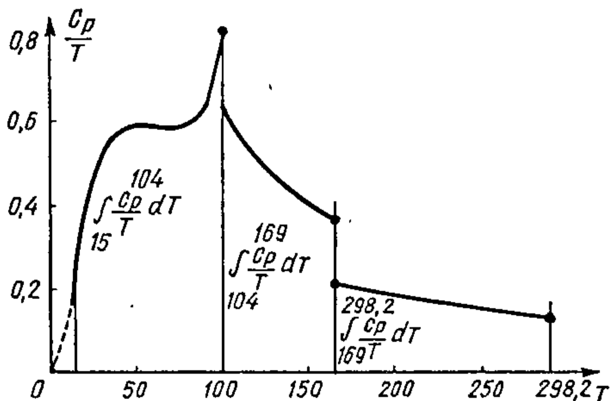
Рыс. 5.5.2. Вызначэнне стандартнай энтрапіі газападобнага этылену па даных аб цеплаёмістасці.
