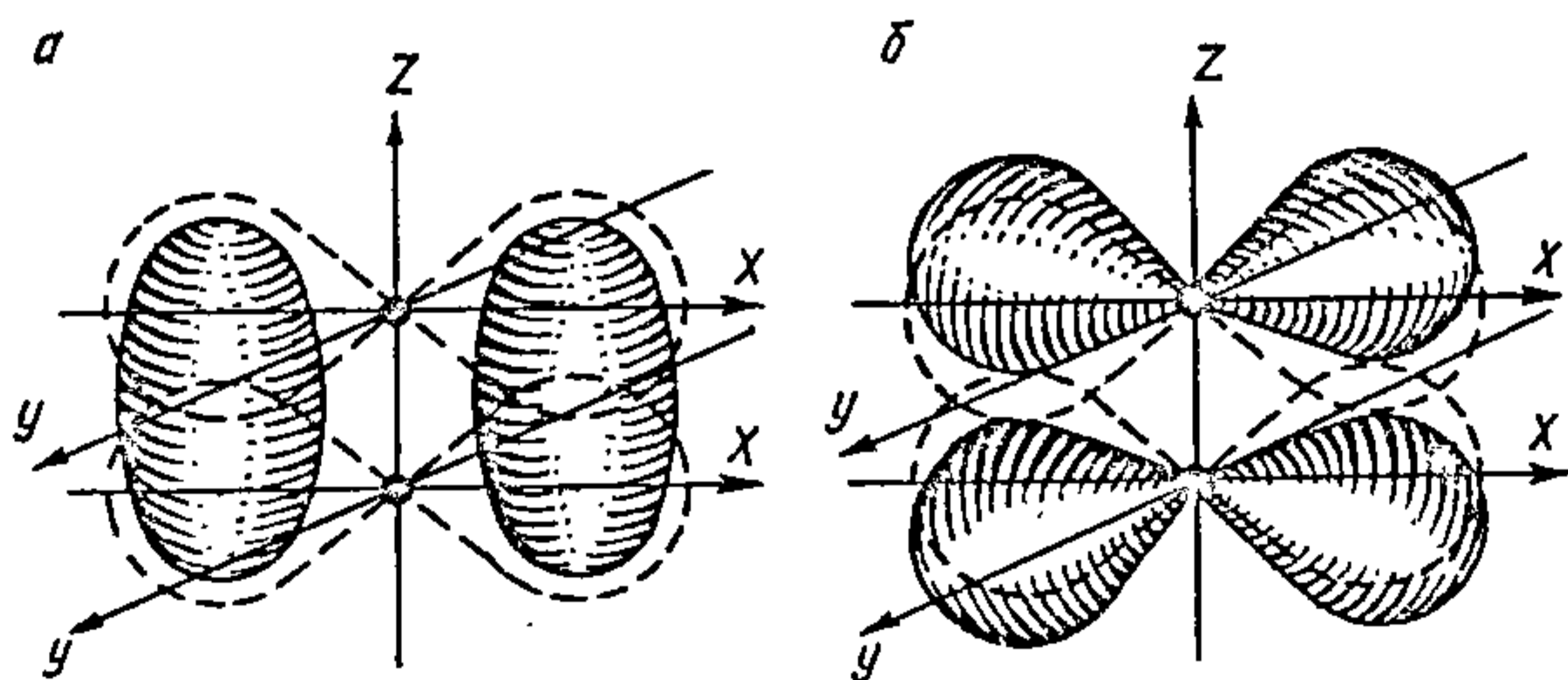
Рыс. 23.4.2. Утварэнне малекулярных \pi -арбіталей у двухатамных малекулах гомазлучэнняў.
