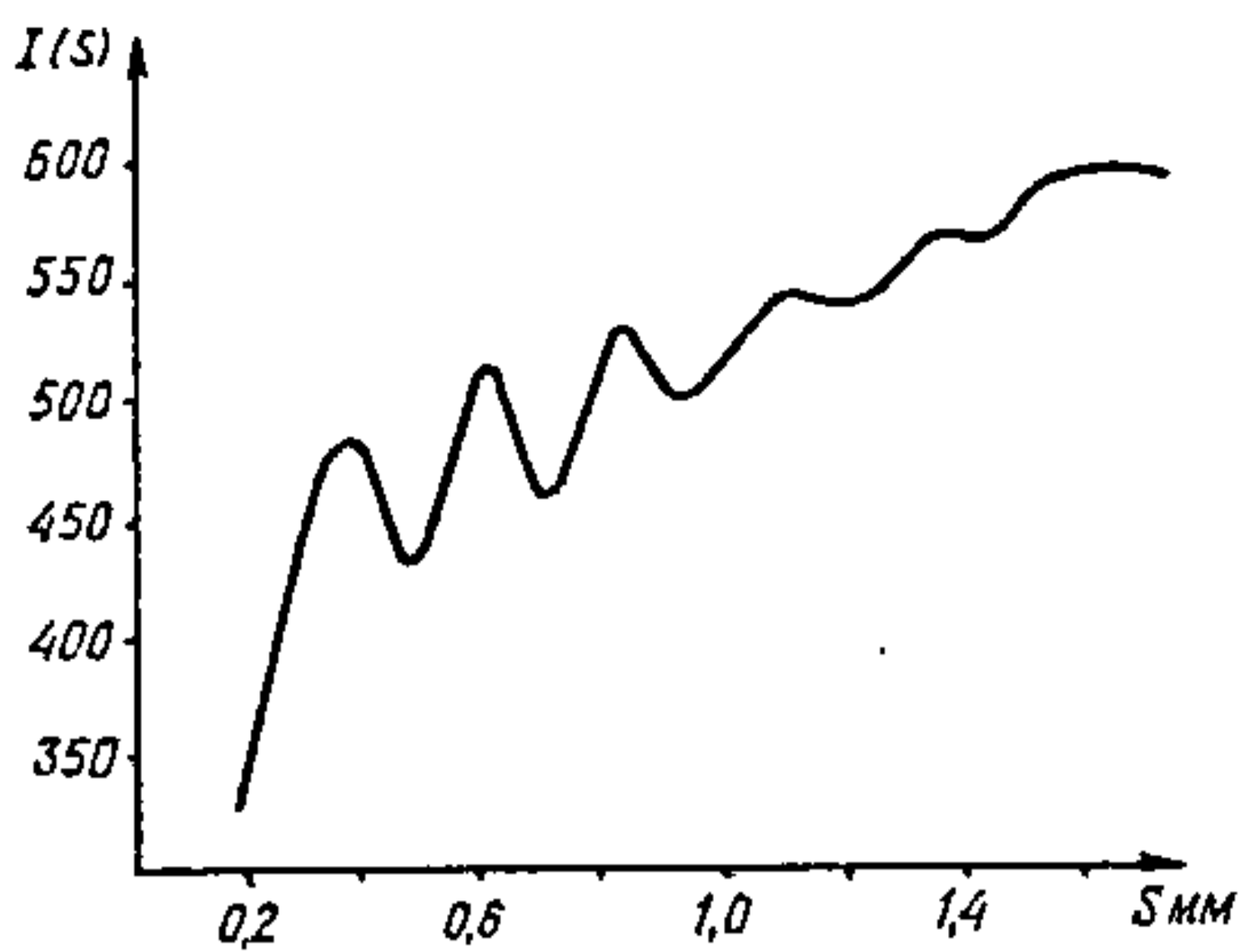
Рис. 18.5.4. Поўная кривая інтэнсіўнасці рассеяння I_{\text{эксп}}(s) малекулы \text{WOBr}_4 .
