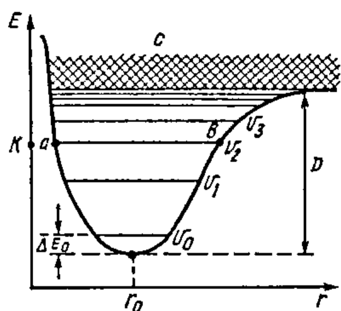
Рыс. 25.1.4. Залежнасць патэнцыяльнай энергіі E двухатамнай малекулы ад між'ядзернай адлегласці r :
