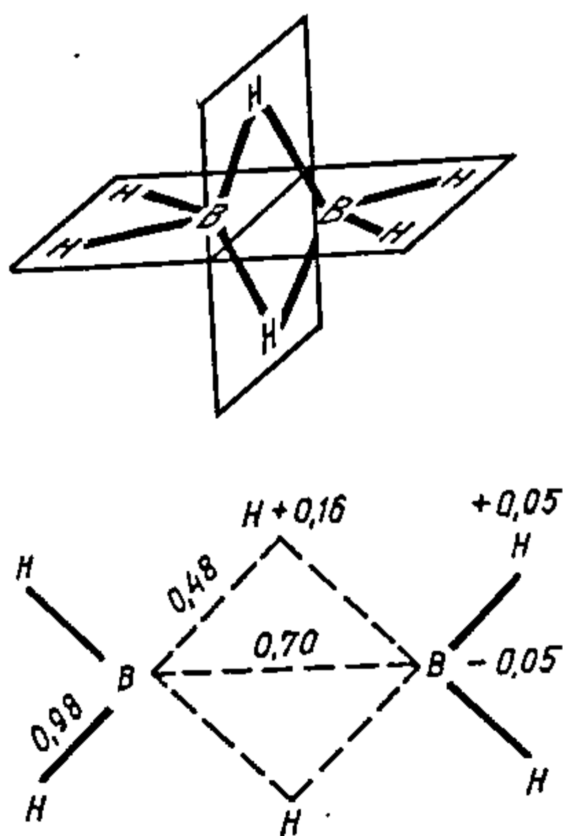
Рыс. 24.3.1. Структура малекулы дыбарану \text{B}_2\text{H}_6 .
