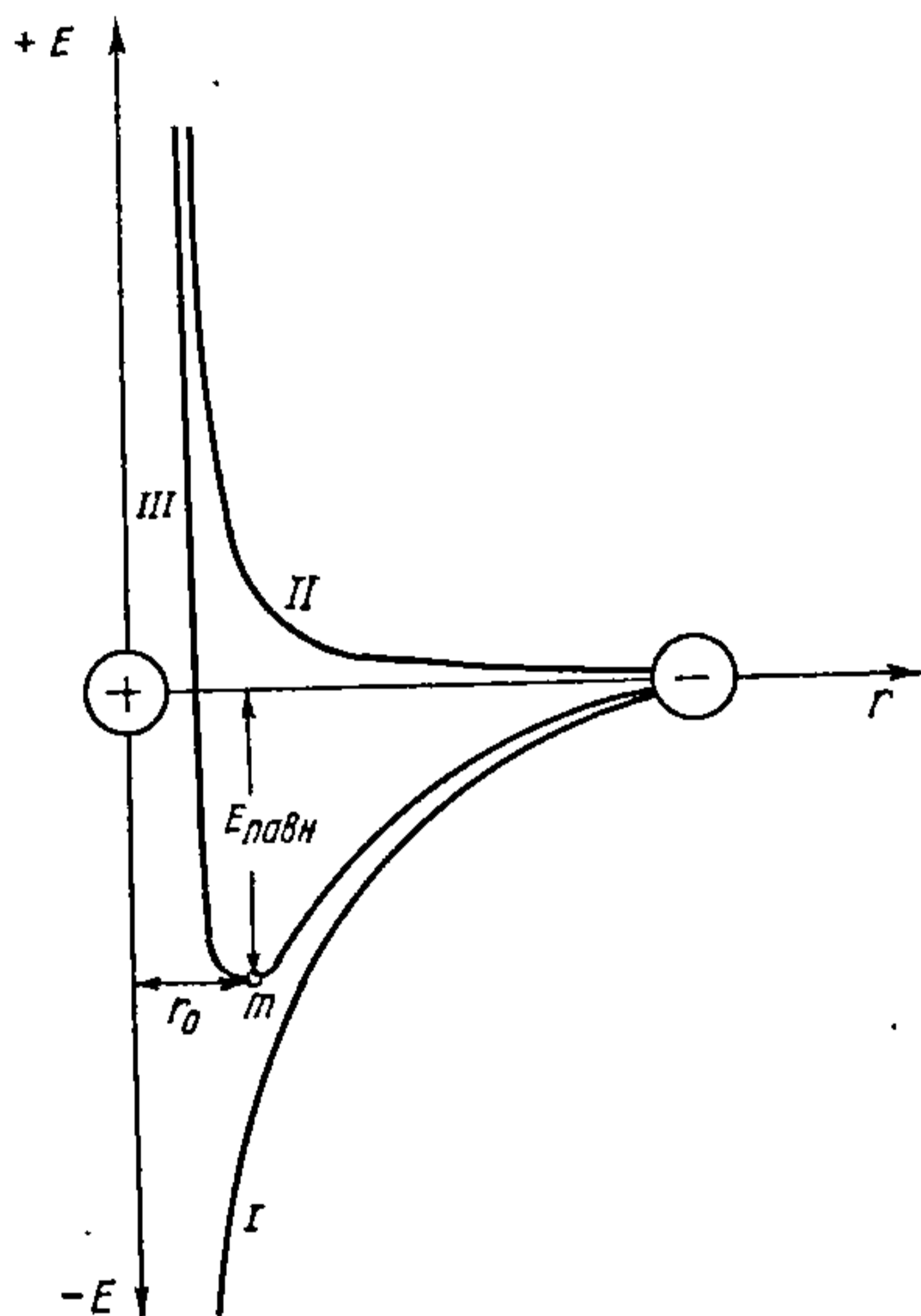
Рыс. 26.2.1. Крывыя патэнцыяльнай энергіі ўзаемадзеяння двух атамаў або супрацьлегла зараджаных іонаў: I — E'(r) ; II — E''(r) ; III — E(r) = E'(r) + E''(r) .
