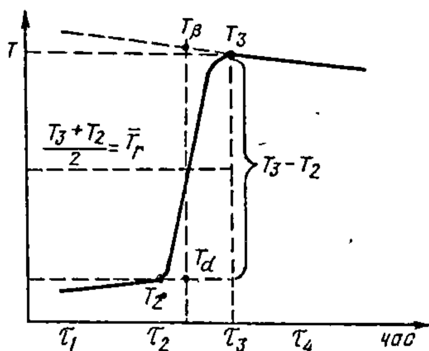
Рыс. 4.11.5. Кривая «тэмпература — час» у каларыметрычным доследзе: T_1 — T_2 — пачатковы перыяд; T_2 — T_3 — галоўны; T_3 — T_4 — канечны.
