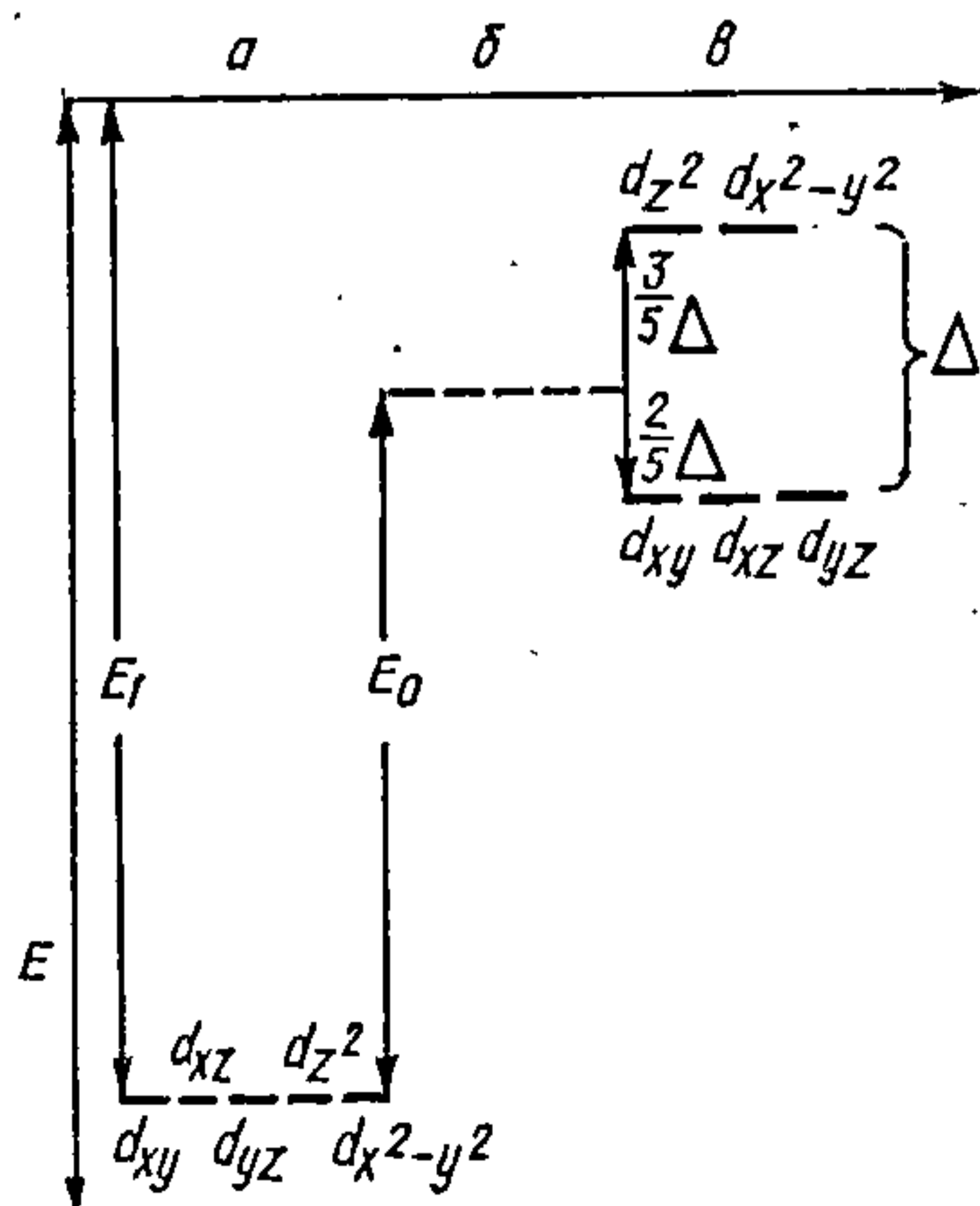
Рыс. 22.3.1. Схема расшчаплення ўзроўню энергіі d -арбіталей цэнтральнага атама пад дзеяннем электростатычнага поля лігандаў (актаэдрычнага):
