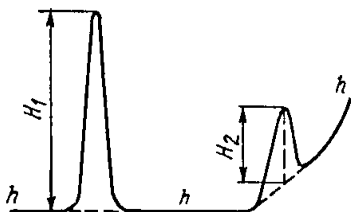
Рыс. 15.2.9. Вымярэнне вышыні піка: H_1, H_2 — вымераная вышыня; h — нулявая лінія.
