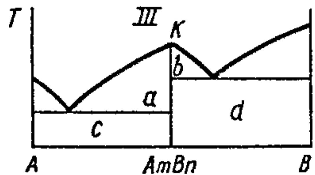
Рыс. 7.6.3. Дыяграма плаўкасці з утварэннем у крышталічнай фазе дваінога злучэння A_mB_n з кангруэнтным пунктам плаўлення: a, b, c, d — двухфазныя вобласці разрыву суцэльнасці; I-II — двухкампанентныя сістэмы з адным агульным кампанентам; III — сумешчаная двухкампанентная сістэма; K — тэмпература кангруэнтнага плаўлення.
