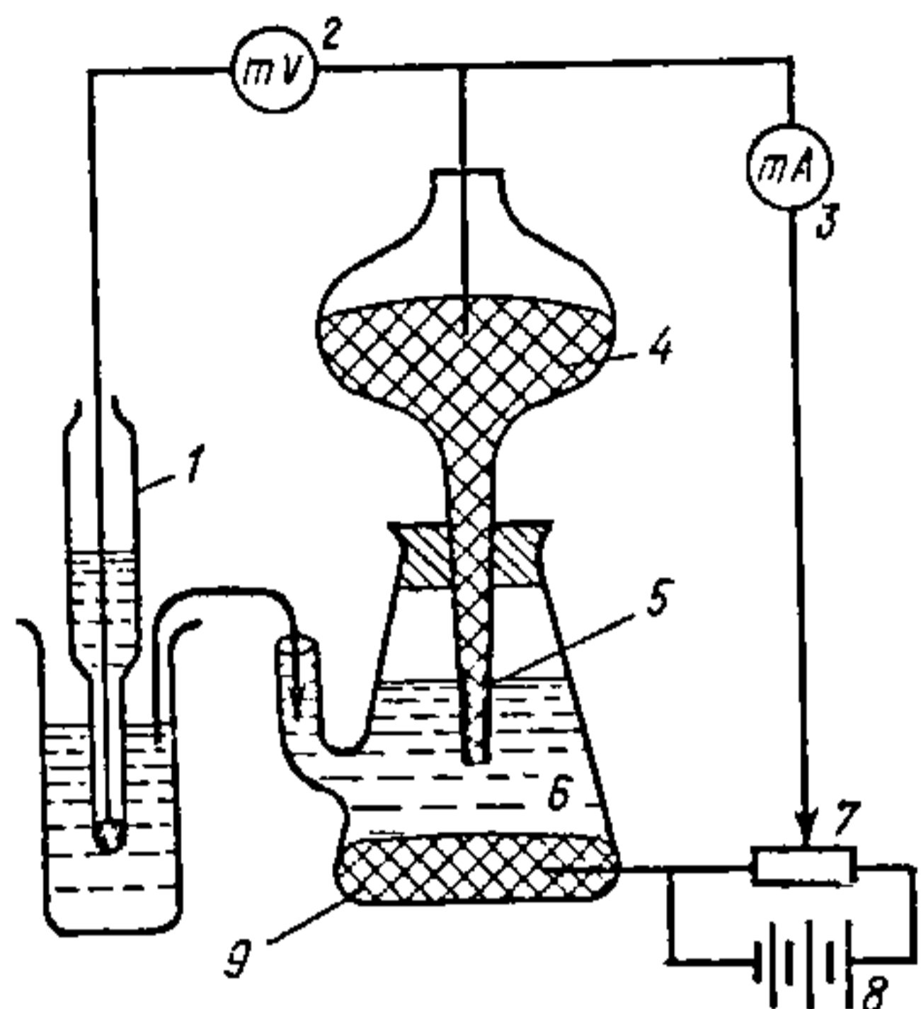
Рыс. 13.4.1. Схема найпрасцейшага палярографа.
