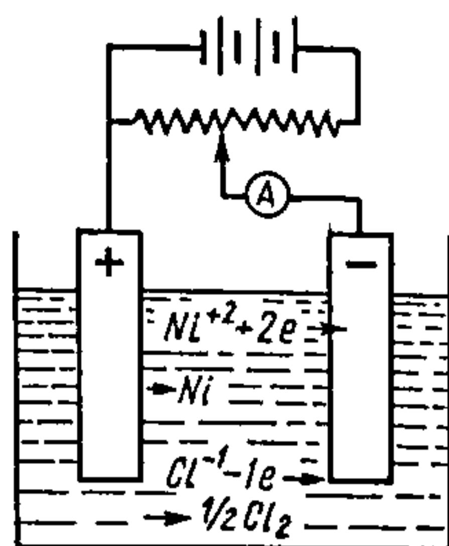
Рис. 12.5.2. Электроліз воднага раствора хларыду нікелю: А — вымяральны прыбор для вызначэння колькасці электрычнасці.
