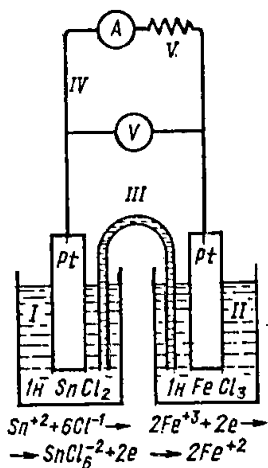
Рис. 12.3.2. Схема гальванічнага элемента, у акісляльна-аднаўленчай рэакцыі якога матэрыял электродаў не прымае ўдзелу.
