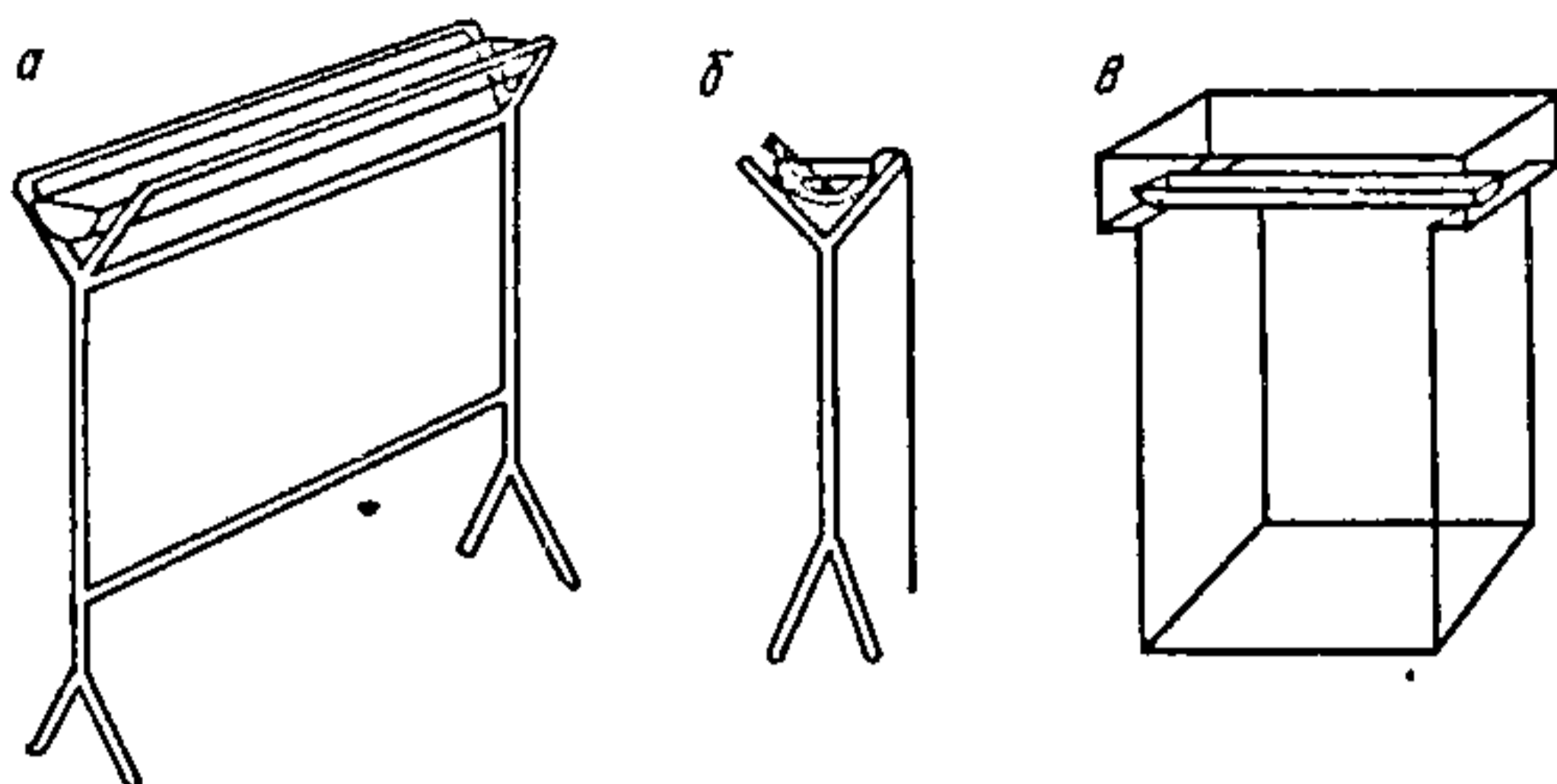
Рыс. 15.3.2. Апаратура для зыходнай ПХ: а — стойка з латком; б — прылада для зыходнай храматаграфіі ў сабраным выглядзе; в — стандартная камера з латком.
