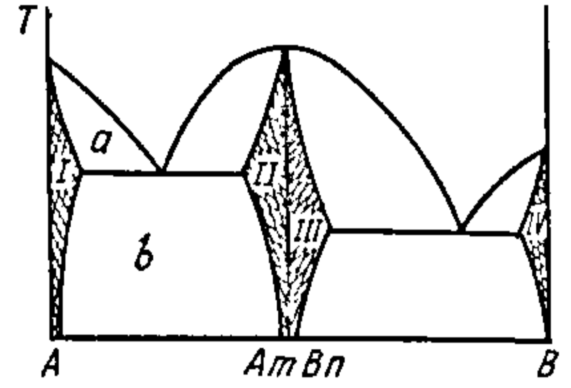
Рис. 7.6.5. Дыяграма плаўкасці з абмежаванай растваральнасцю кампанентаў у цвёрдых фазах: I — IV — вобласці цвёрдых раствораў; a, b — двухфазныя вобласці разрыву суцэльнасці.
