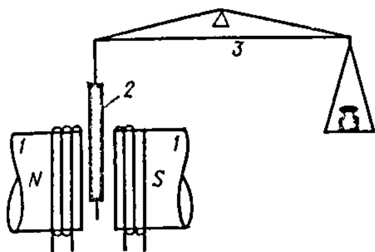
Рыс. 30.1.5. Схематычны відарыс магнітных вагаў Гуі:
