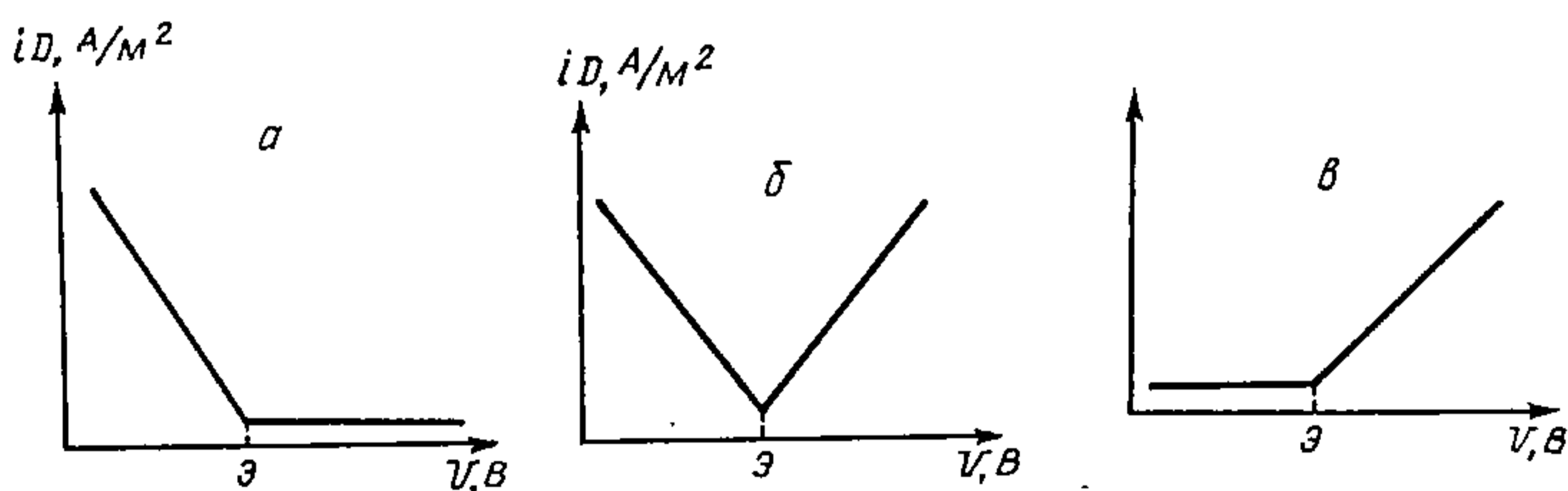
Рыс. 13.5.1. Крывая ампераметрычнага цітравання:
