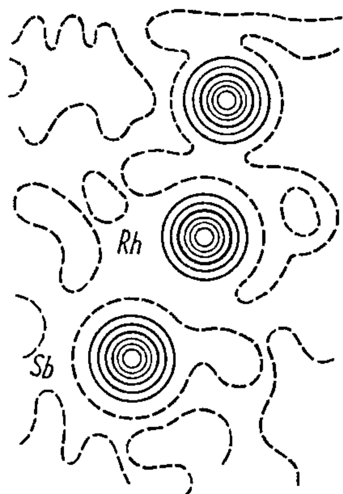
Рис. 28.2.5. Размеркаванне электроннай шчыльнасці ў крышталі RhSb_2 .
