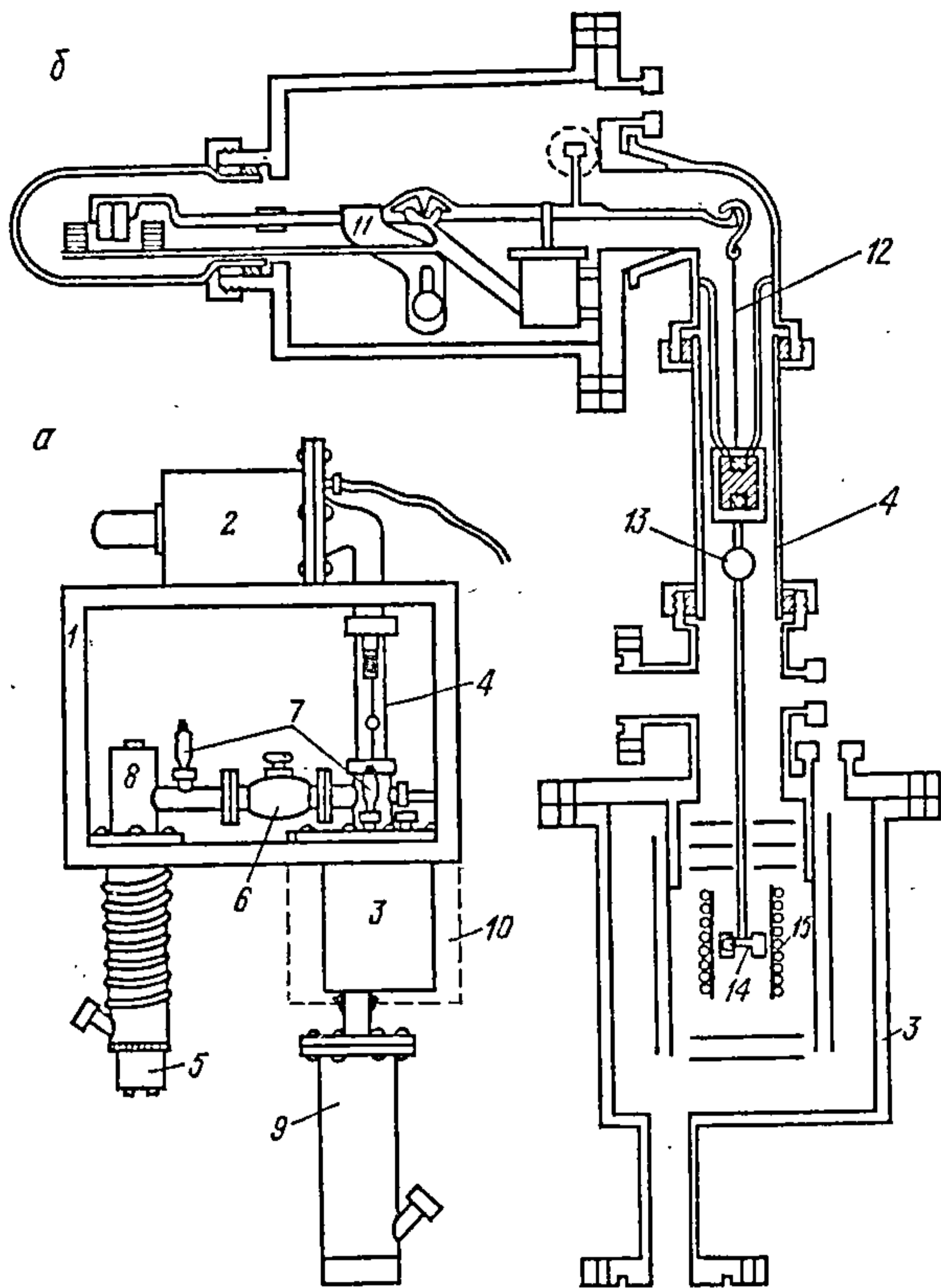
Рис. 6.5.5. Эфузійно-тарзійенная ўстаноўка:
