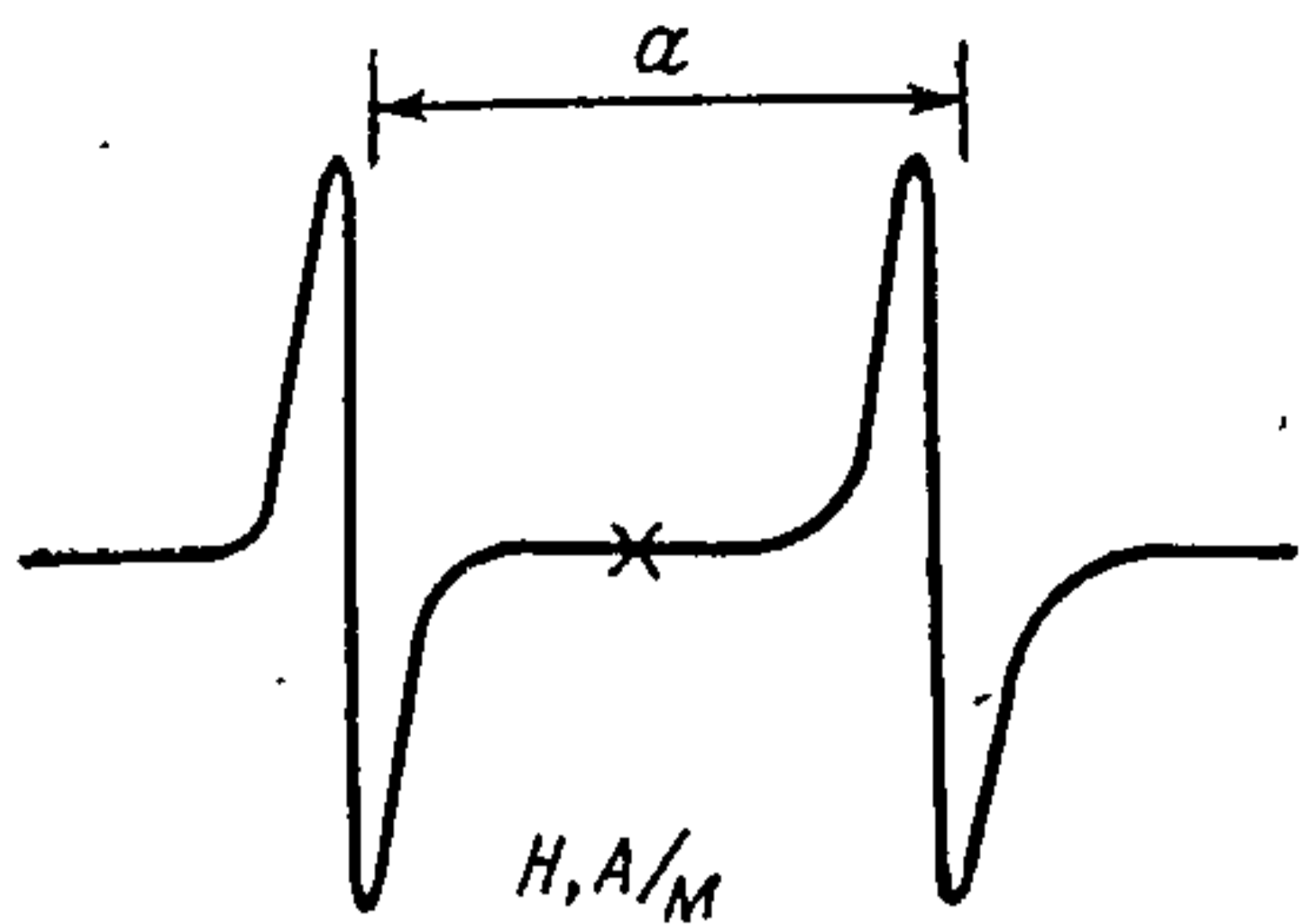
Рис. 30.3.3. Спектр ЭПР атома водорода.
