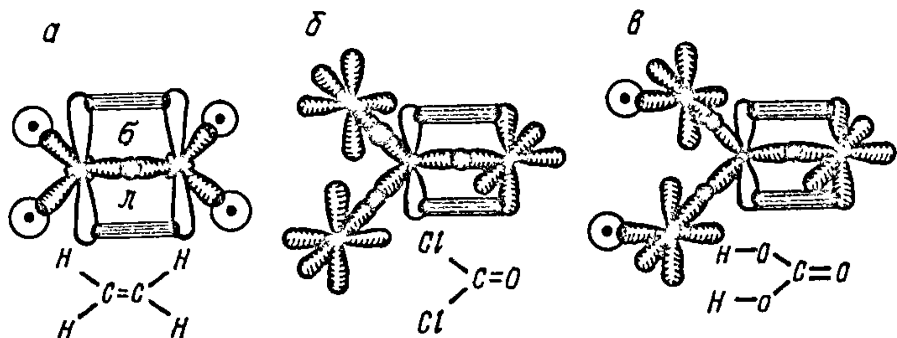
Рис. 21.3.3. Схема молекул з \sigma - і \pi -св'язямі пры наяўнасці sp^2 -гібрыдызацыі.
