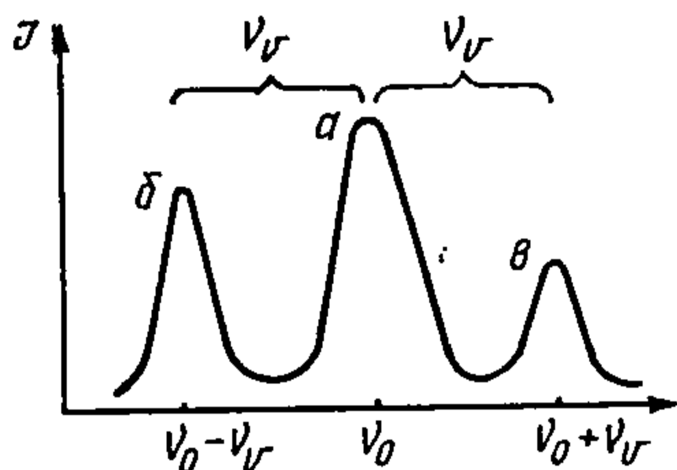
Рыс. 25.3.2. Схематычны відарыс ліній у спектры КР святла: а — лінія рэлеўскага рассеяння з частатой \nu_0 ; б — стоксава лінія з частатой \nu_0 - \nu_v ; в — антыстоксава лінія з частатой \nu_0 + \nu_v .
