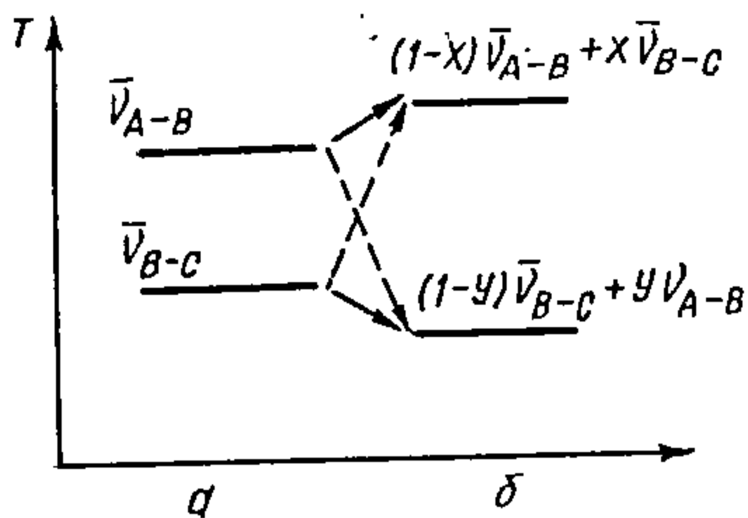
Рис. 25.2.5. Энергетическая схема (термы) взаимодействия нормальных колебаний у молекулы ABC: а — термы не взаимодействующих нормальных колебаний у групп А — В и В — С; б — смешанные термы.
