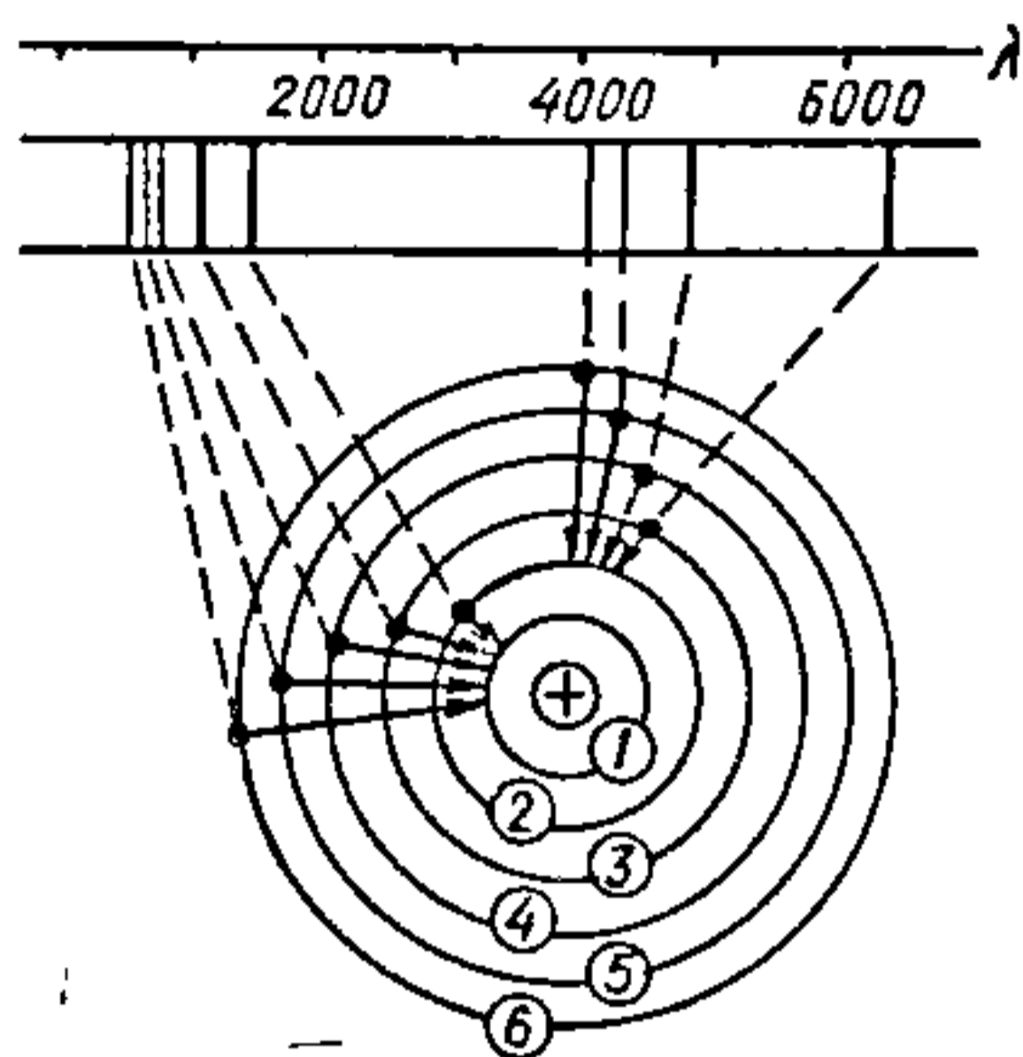
Рыс. 16.1.1. Спектр некаторых пераходаў электрона ў атаме вадароду.
