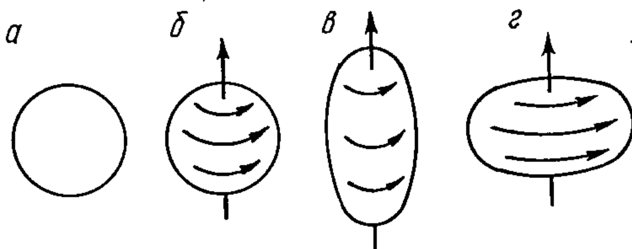
Рыс. 30.4.1. Тыпы ядзер:
