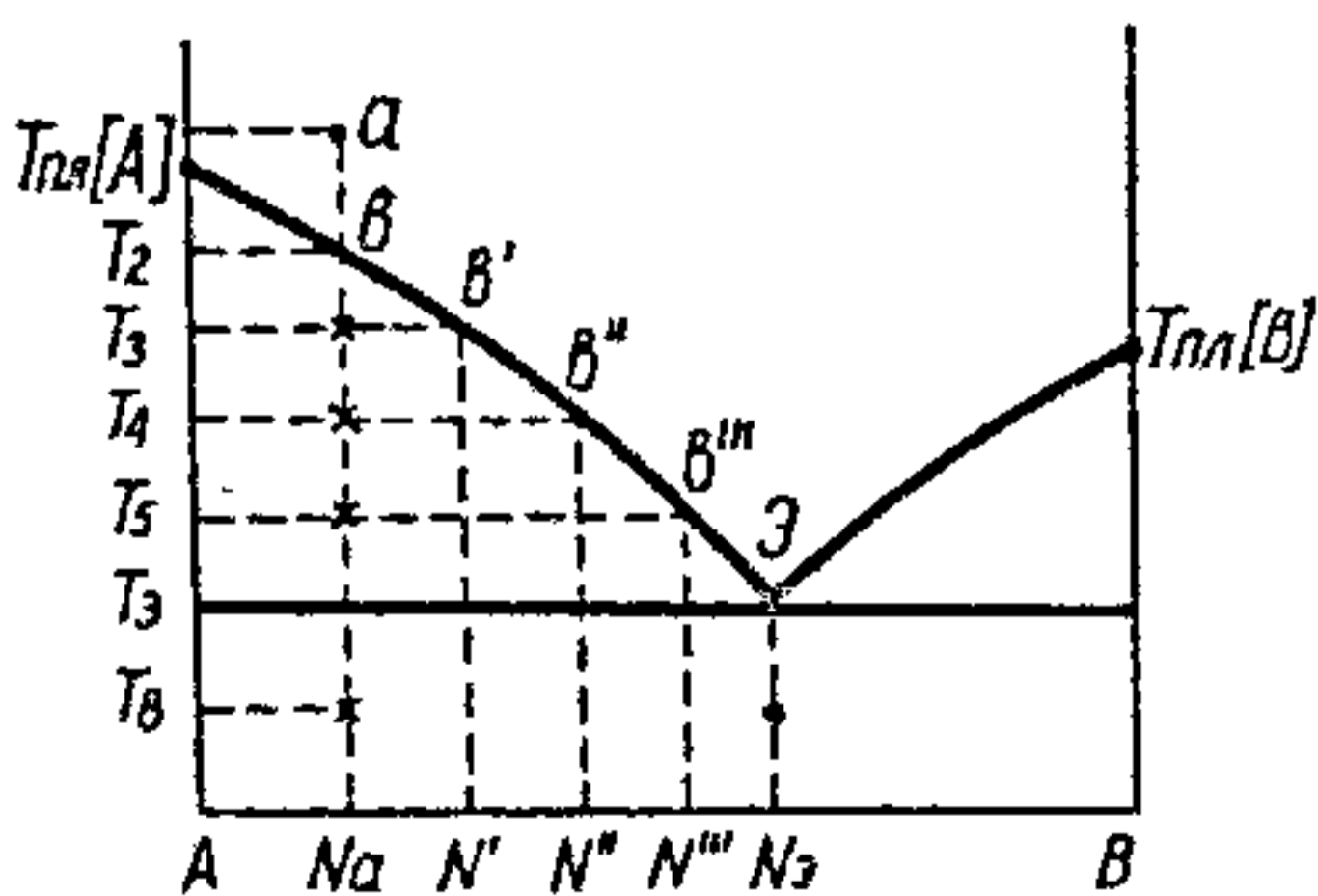
Рыс. 7.6.2. Аналіз дыяграмы плаўкасці з адной эўтэктыкай.
