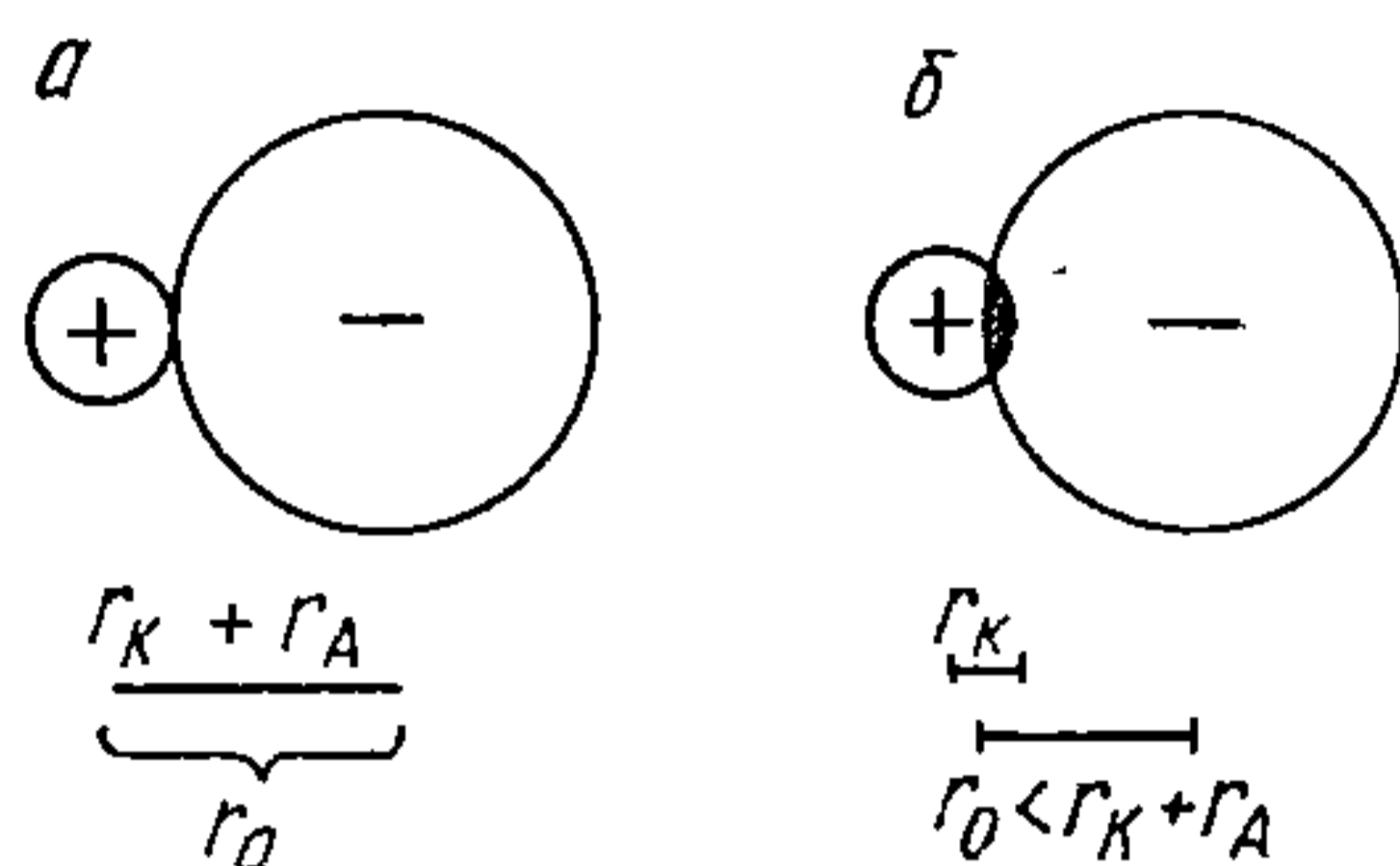
Рыс. 26.3.1. Палярызацыя іонаў.
