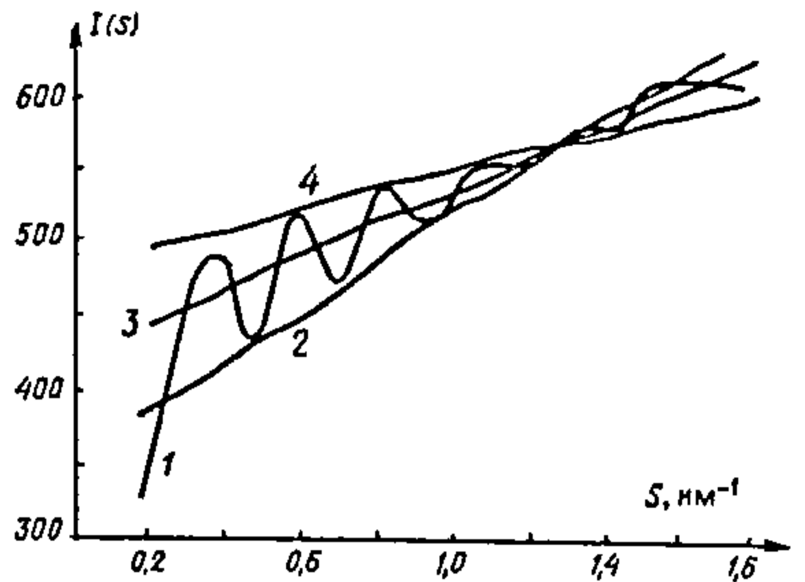
Рис. 18.5.5. Лінія фону G(s) , праведзеная па методыцы агібаючых крывой I_{\text{эксп}}(s) малекулы \text{WOBr}_4 : 1 — кривая I_{\text{эксп}}(s) ; 2, 4 — агібаючыя I_{\text{эксп}}(s) ; 3 — лінія фону G(s) .
