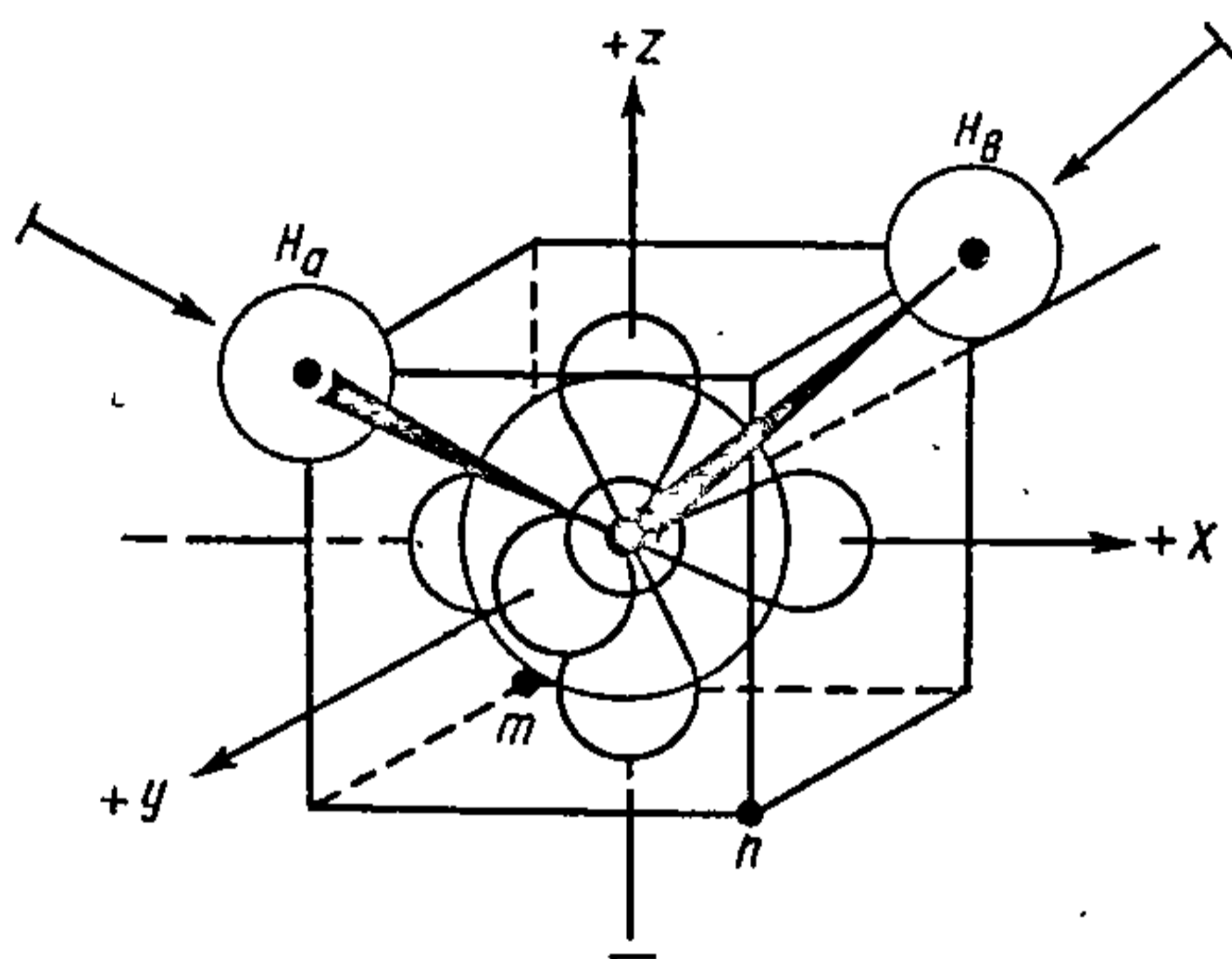
Рыс. 24.6.1. Схема збліжэння двух атамаў вадароду з атамамі кіслароду пры ўтварэнні малекулы \text{H}_2\text{O} .
