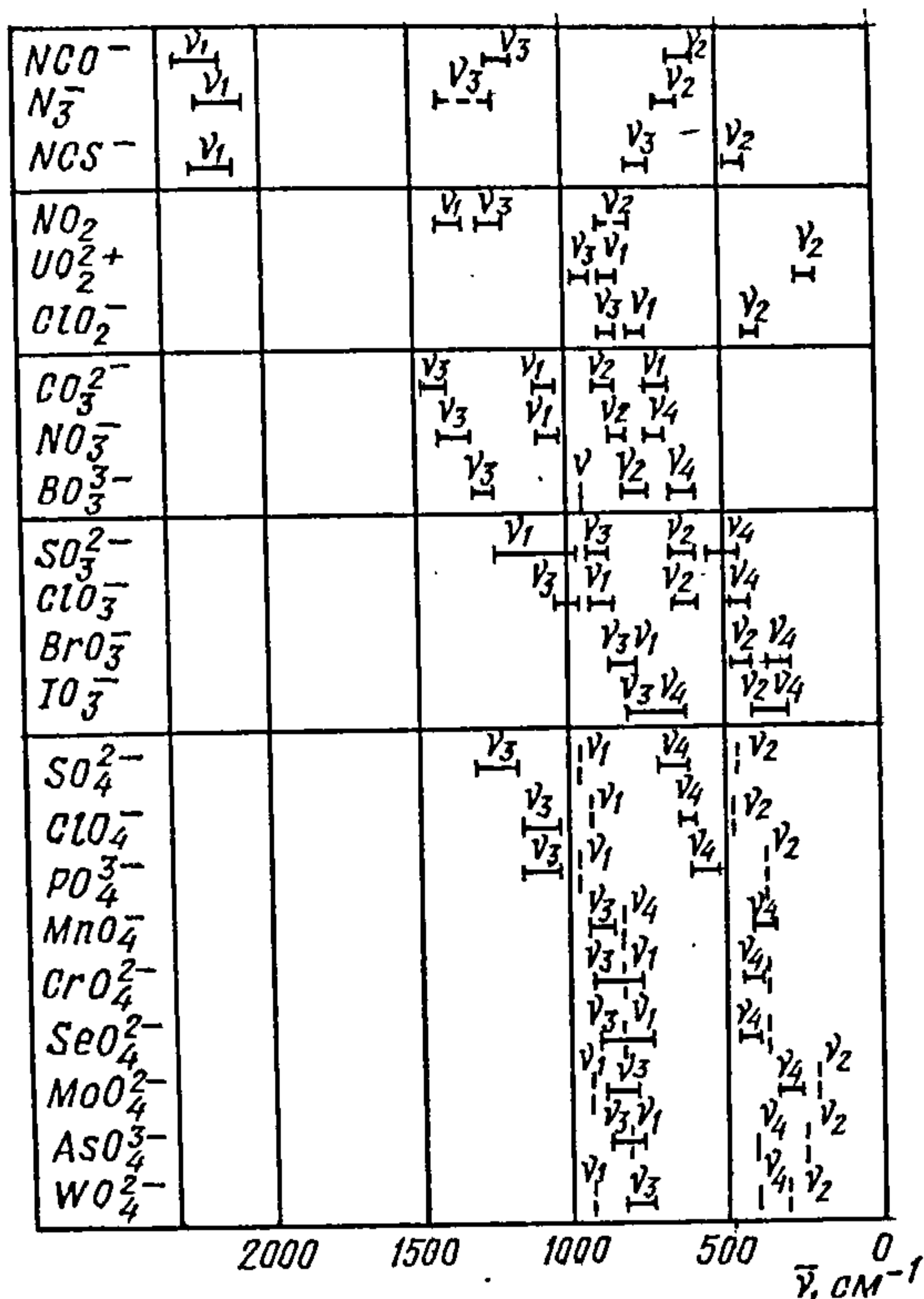
Рис. 25.7.3. Диапазоны ИЧ-частот некоторых наибольших распаёсуджаних неорганических ионау.
