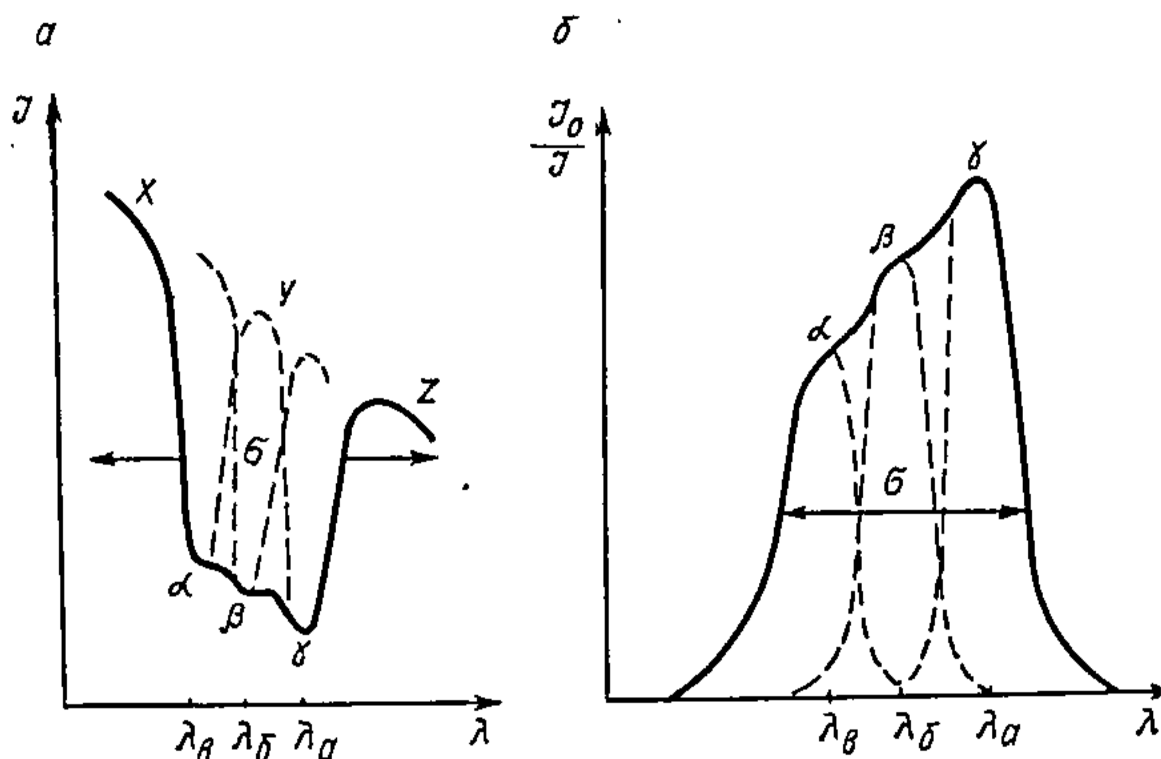
Рыс. 25.1.6. Спектр паглынання, які адпавядае крывым патэнцыяльнай энергіі на рыс. 25.1.5 у каардынатах (а) I=f(\lambda) і (б) I_0/I=f'(\lambda)\zeta : лінія x, y, z — ход інтэнсіўнасці I неперапыннага спектра крыніцы святла; \alpha, \beta, \gamma — тонкая вагальная структура на піку паглынання пры \lambda_a, \lambda_b, \lambda_c , што адпавядае электронным пераходам a, b, c на рыс. 25.1.5; \delta — пік паглынання, які задавальняе электроннаму пераходу e \rightarrow e' .
