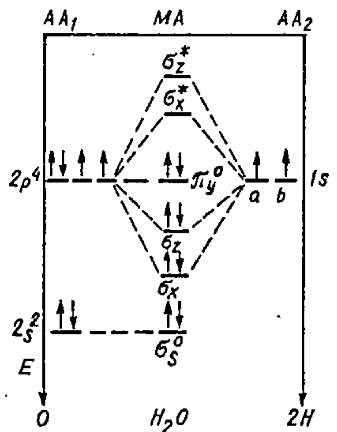
Рыс. 24.6.2. Энергетычная дыяграма МА малекулы \text{H}_2\text{O} .
