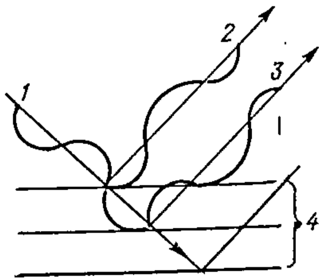
Рис. 28.1.4. Схема ўзнікнення эфекту гашэння рассеянай крышталём хвалі:
