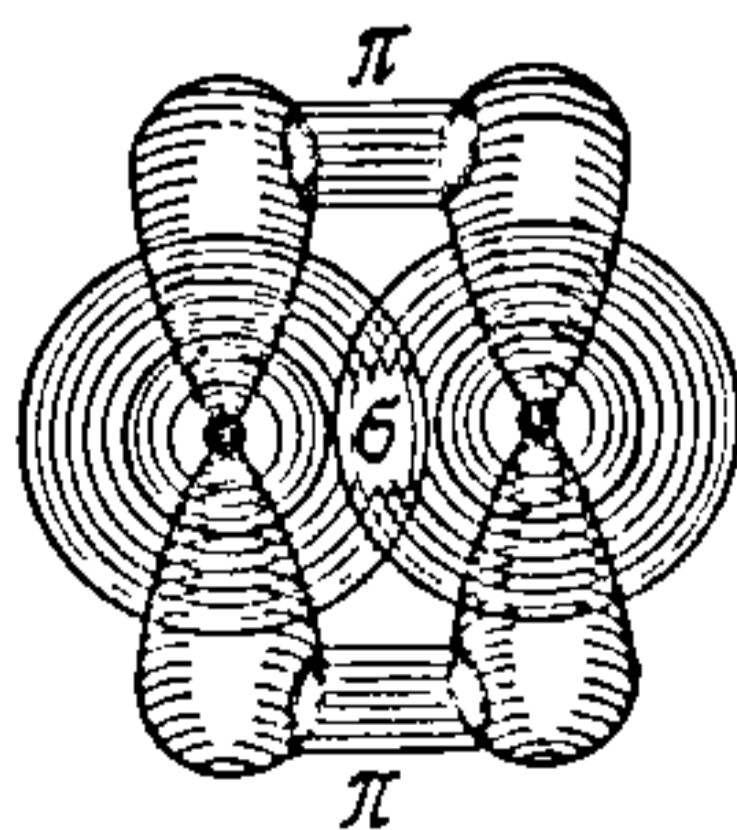
Рыс. 21.1.3. Схема малекулы \text{Be}_2 .
