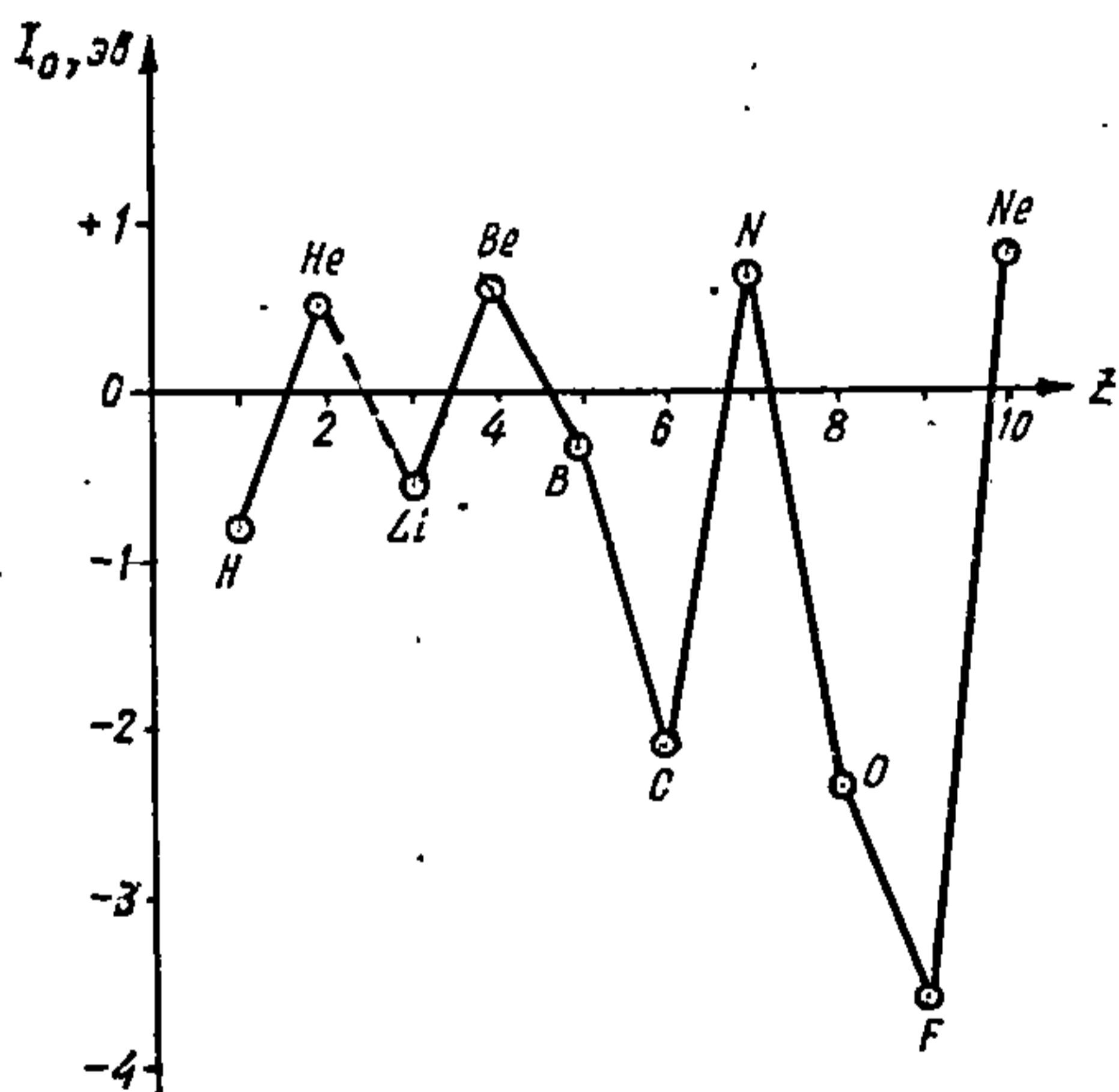
Рыс. 19.1.3. Залежнасць роднасці да электрона I_0 атамаў хімічных элементаў ад зараду ядра.
