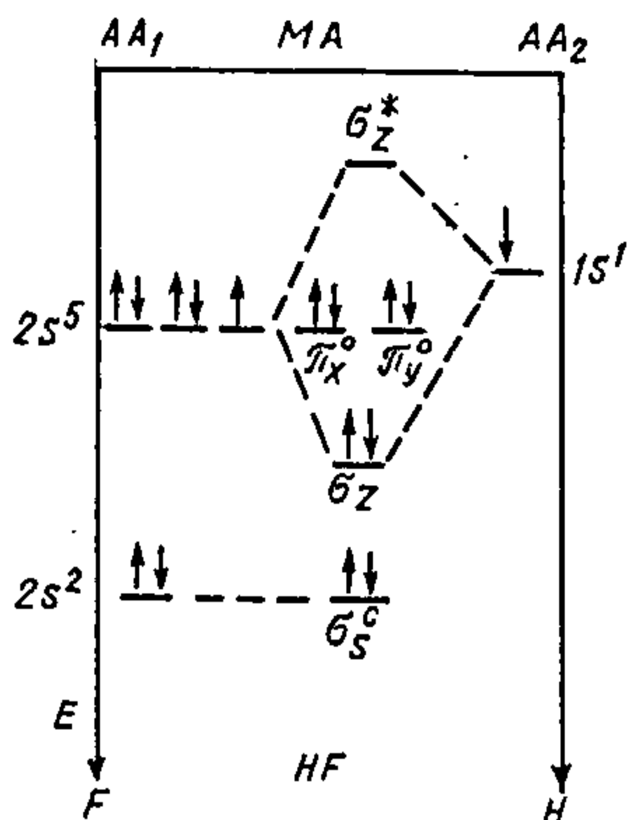
Рис. 24.7.2. Енергетична діаграма МА молекули HF.
