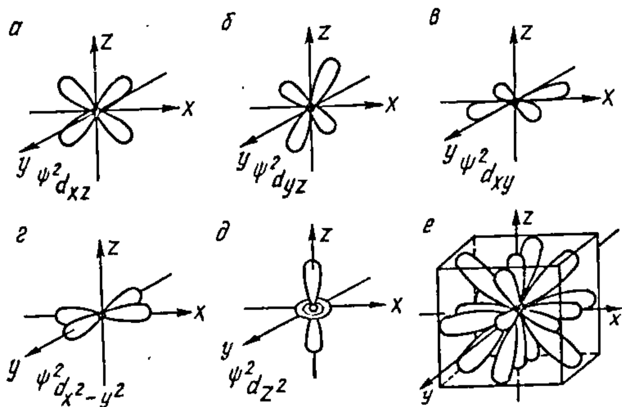
Рыс. 17.5.3. Формы d -арбіталей узбуджанага атома вадароду.
