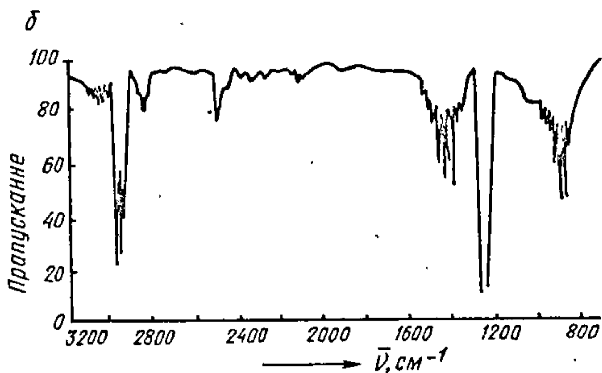
Рис. 25.7.2. ІЧ-спектр \text{CH}_3\text{I} ; а — вадкі ёдзісты метыл, б — газападобны.
