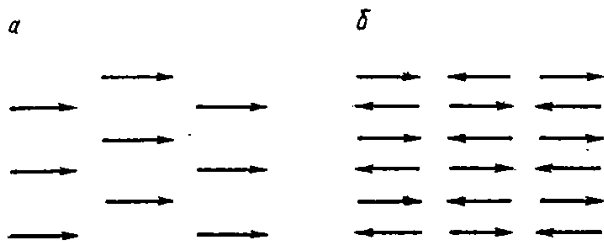
Рыс. 30.1.2. Розныя тыпы самаадвольнай арыентацыі парамагнітных часціц у крышталі.
