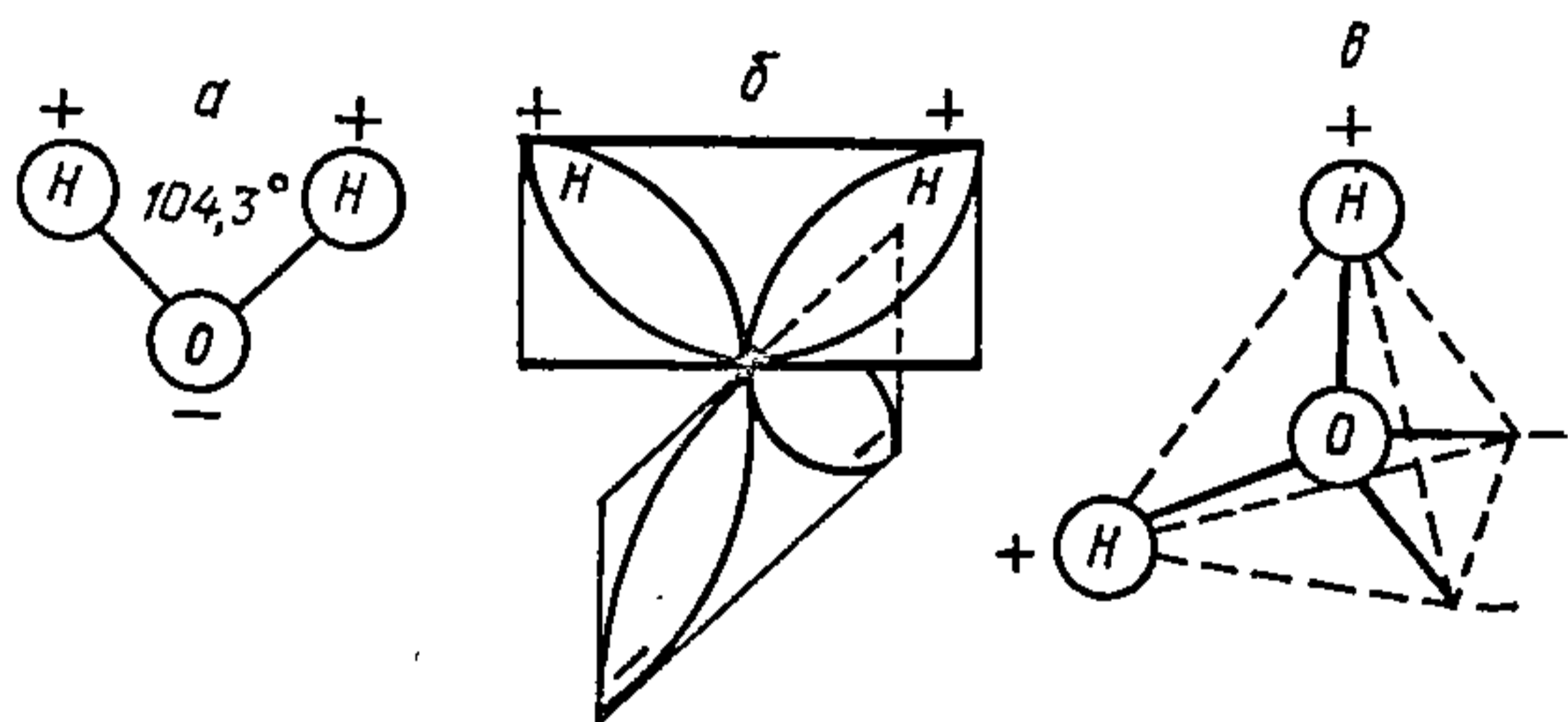
Рыс. 9.1.1. Структура малекулы вады:
