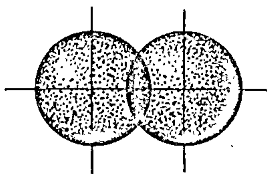
Рыс. 21.1.2. Схема \sigma -связі ў малекуле \text{Li}_2 .
