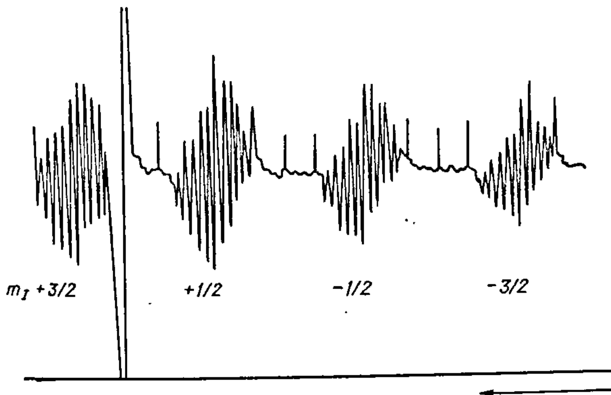
Рис. 30.3.5. Спектр біс-саліцылальдэгідімінату медзі (II).
