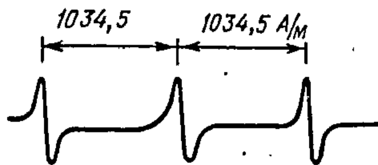
Рис. 30.3.4. Спектр анион-радикалу \text{ON}(\text{SO}_3)_2 у водном раствору 0,01 \text{ M } [\text{ON}(\text{SO}_3)_2\text{Na}_2] при 300 \text{ K} .
