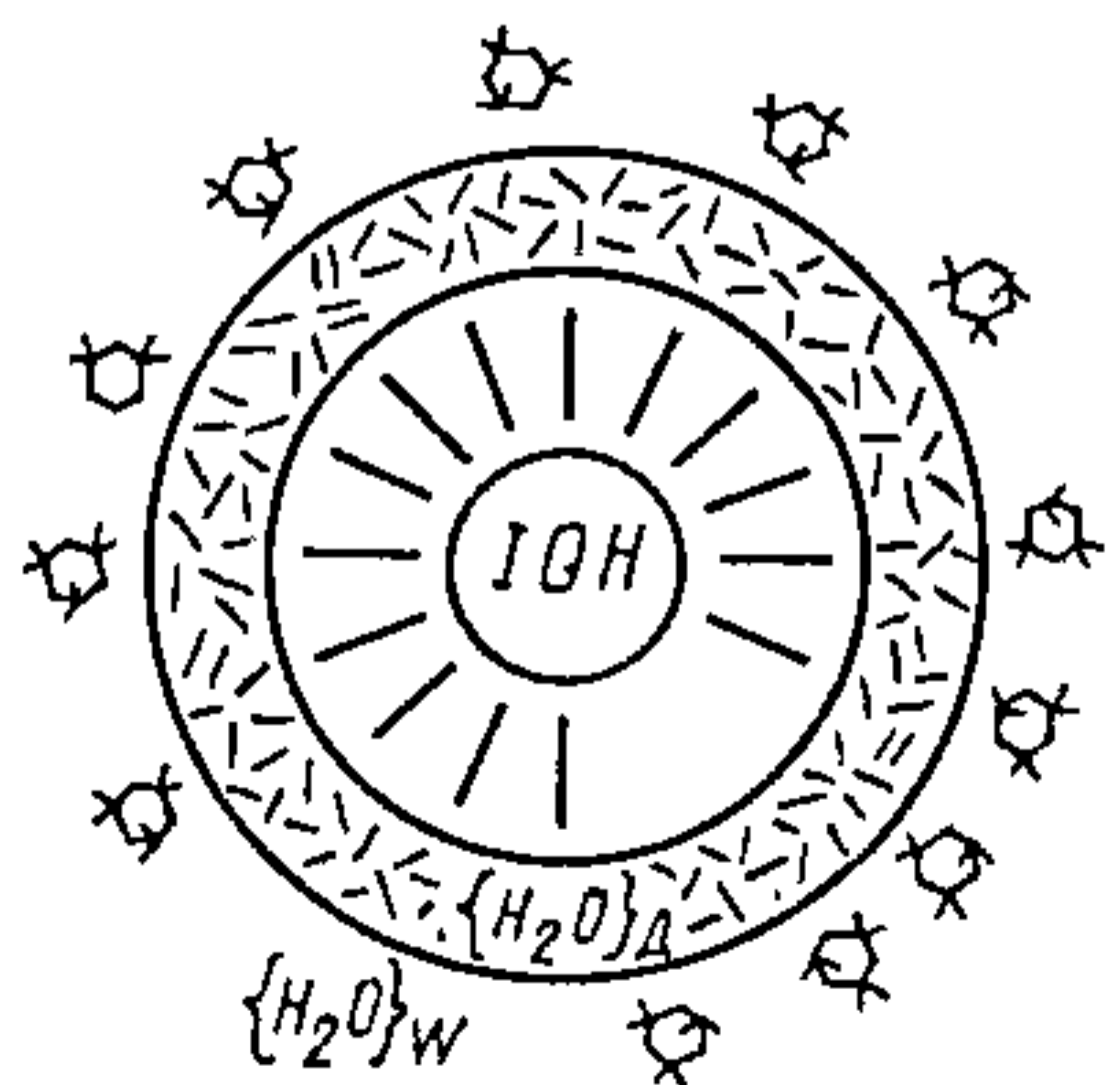
Рыс. 9.1.2. Змяненне структуры вады ў электростатычным полі іонаў.
