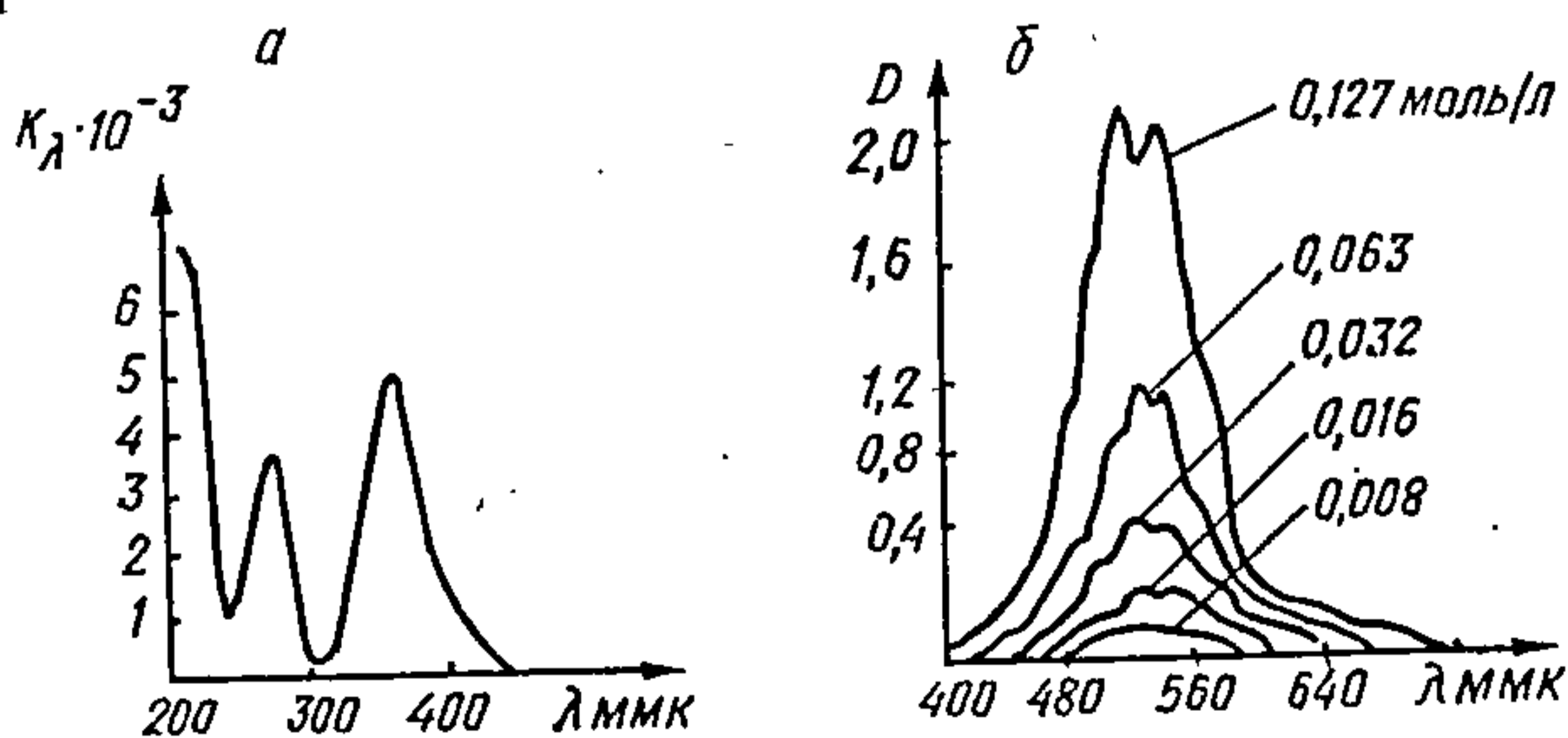
Рыс. 25.6.1. Спектры паглынання водных раствораў храмату калію (а) і перманганату калію (б).
