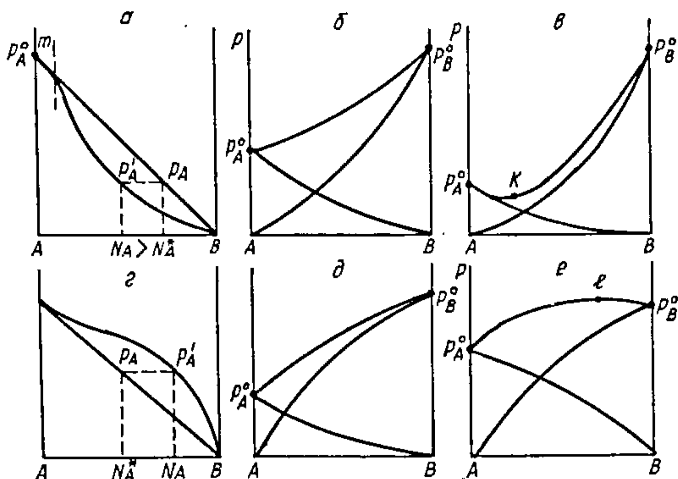
Рыс. 8.3.2. Характар дыяграм p=f(N) з адмоўным (а, б, в) і дадатным (г, д, е) адхіленнямі ад закону Рауля.
