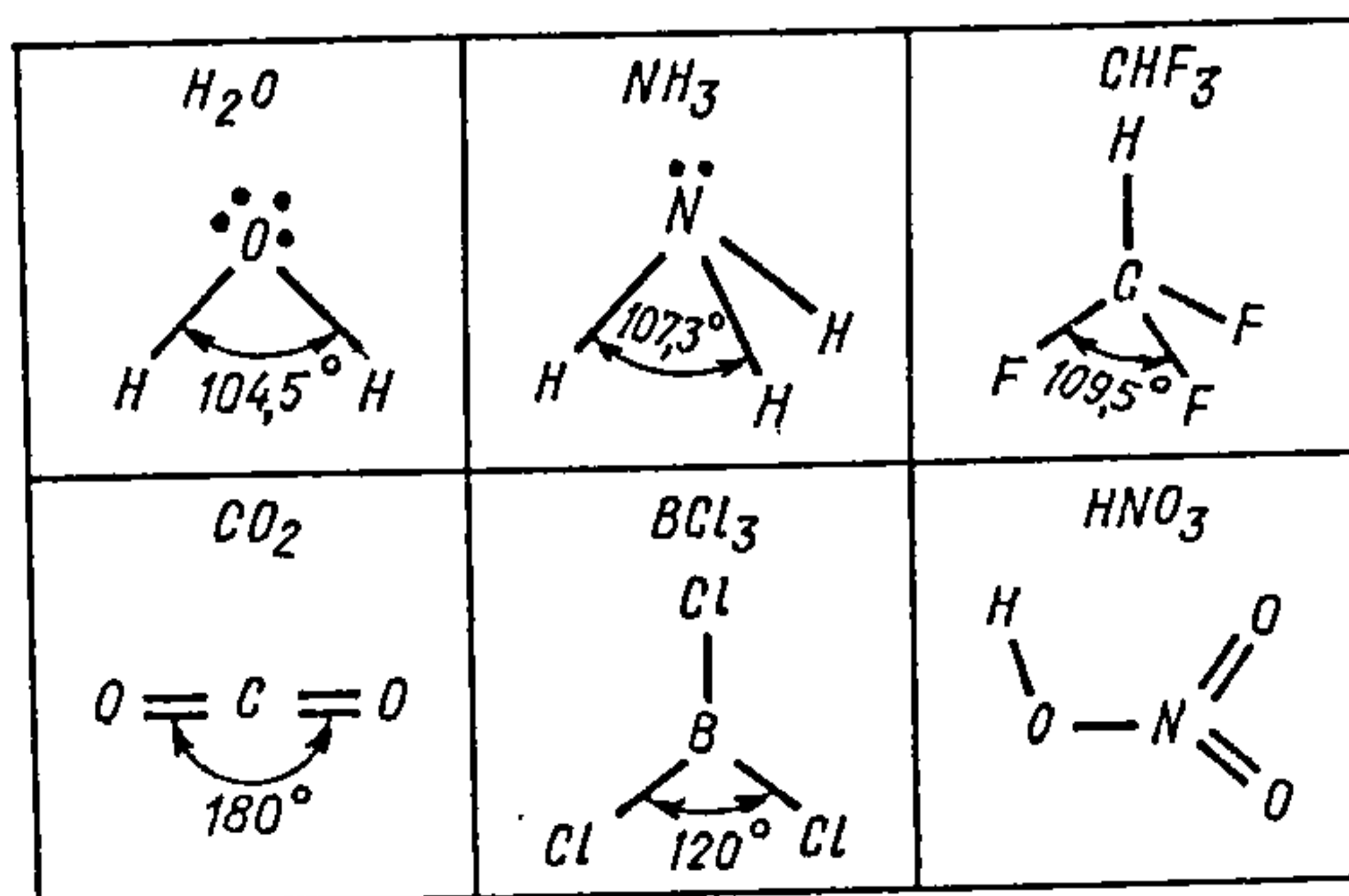
Рыс. 21.2.1. Структуры некаторых неарганічных малекул.
