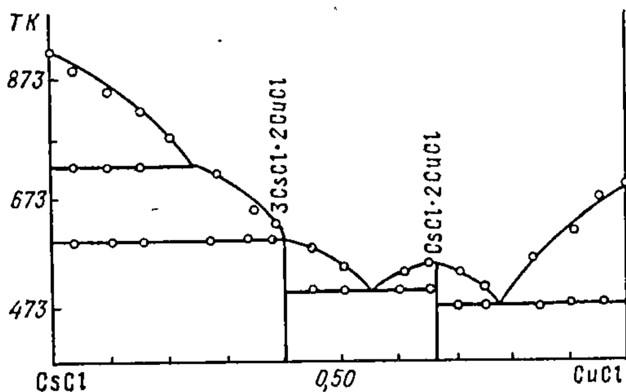
Рыс. 7.12.1. Дыяграма плаўкасці сістэмы CsCl—CuCl.
