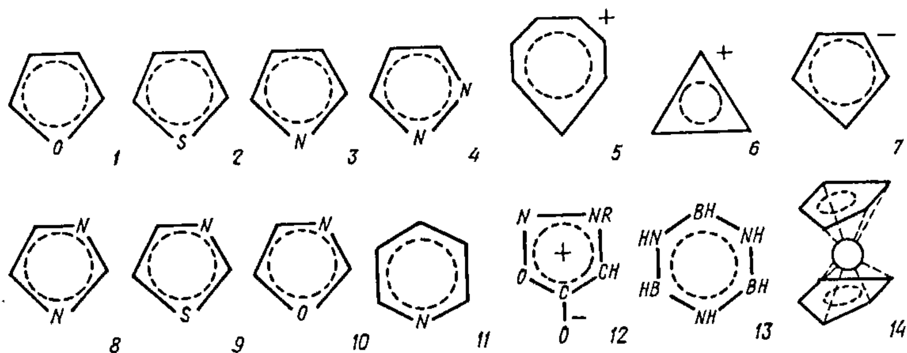
Рыс. 21.4.3. Схема структур гетэрацыклічных злучэнняў: 1 — фуран; 2 — тыёфен; 3 — пірол; 4 — піразол; 5 — імідазол; 6 — трызол; 7 — гексазол; 8 — пірыдзін; 9 — катыён трапілію; 10 — катыён цыклапрапенілію; 11 — аніён цыклапентадыенілію; 12 — біпалярны сіддон; 13 — боразол; 14 — ферацэн.
