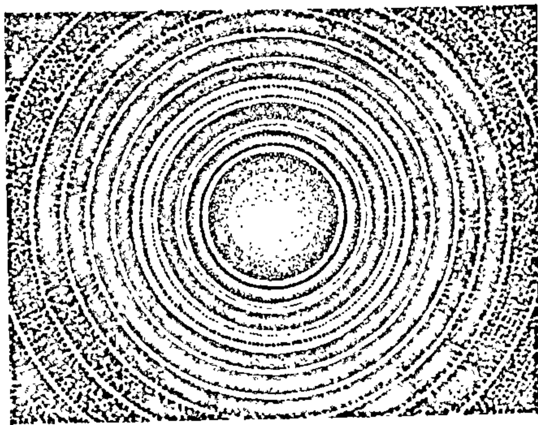
Рыс. 18.4.3. Электронаграма аксиду хрому.
