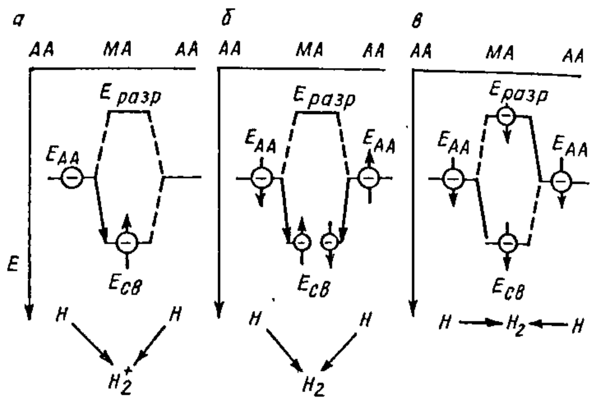
Рис. 23.3.3. Размеркаванне электронаў па МА ў іоне \text{H}_2^+ і ў малекуле \text{H}_2 з антыпаралельнымі і паралельнымі спінамі электронаў.
