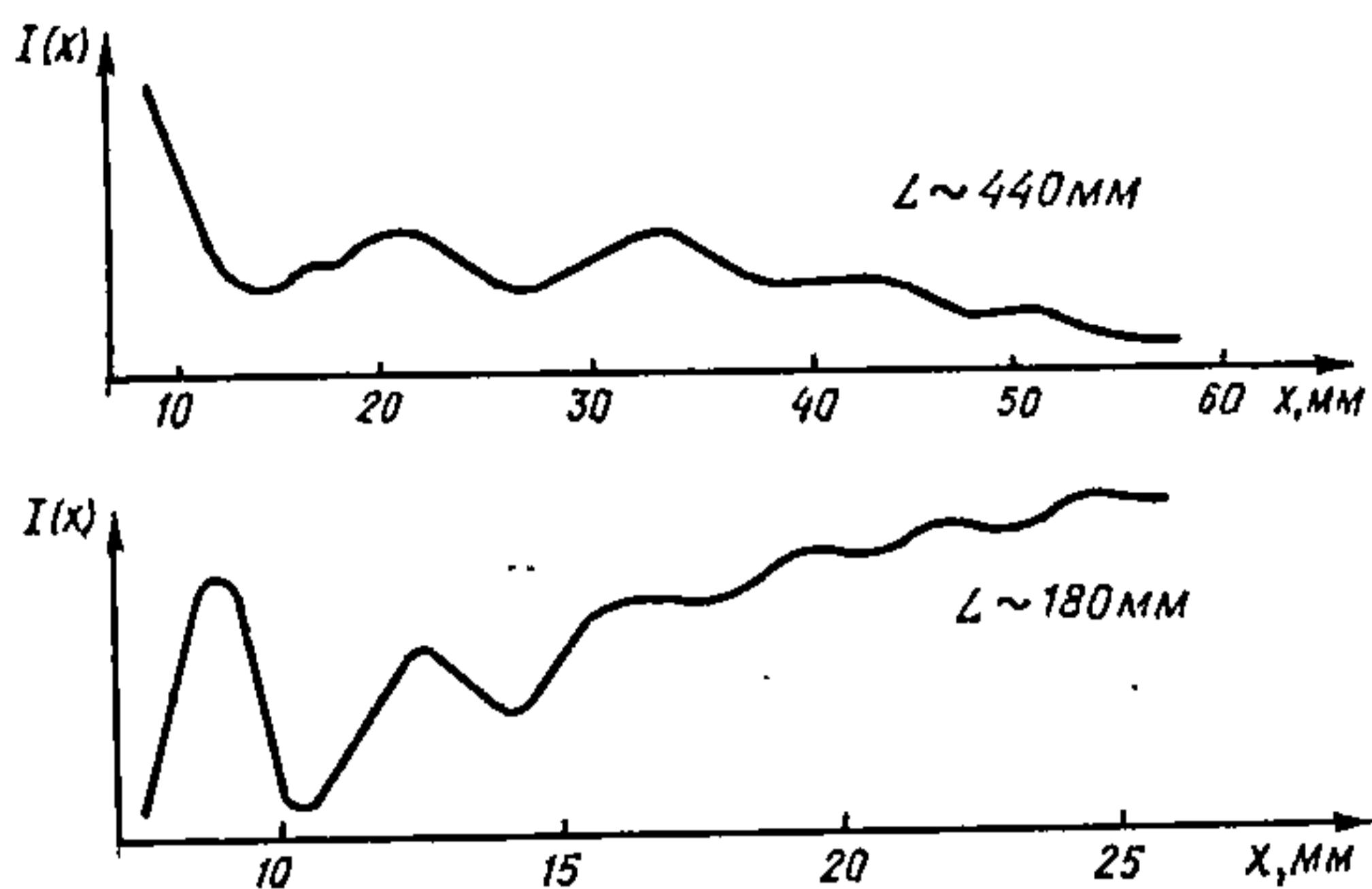
Рис. 18.5.3. Мікрофотограми електронаграми парою \text{WOb}_4 .
