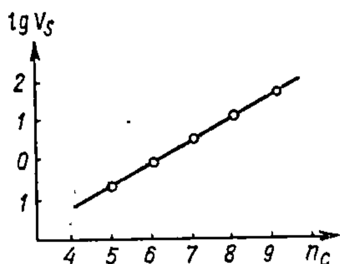
Рыс. 15.2.8. Залежнасць \lg V_s n -алканаў на графітаванай тэрмічнай сажы пры 423 К ад ліку атамаў вугляроду n_c .
