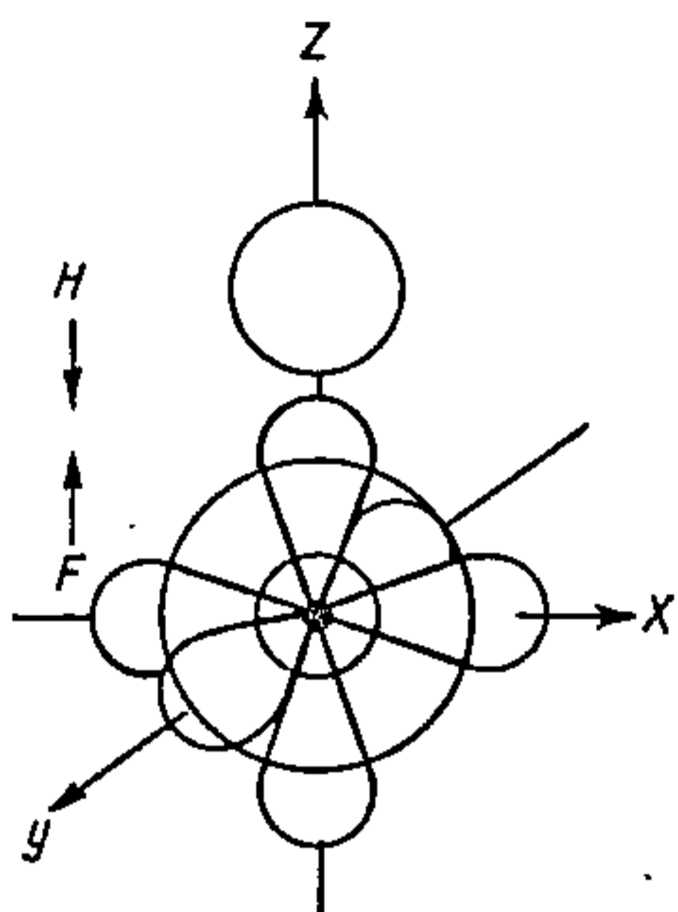
Рис. 24.7.1. Схема зблизження атома водороду і фтору при утворенні молекули HF.
