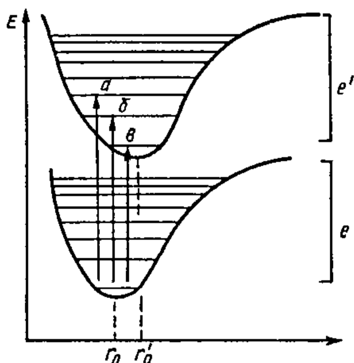
Рыс. 25.1.5. Крывыя патэнцыяльнай энергіі для асноўнага e і ўзбуджанага e' электронных станаў двухатамнай малекулы:
