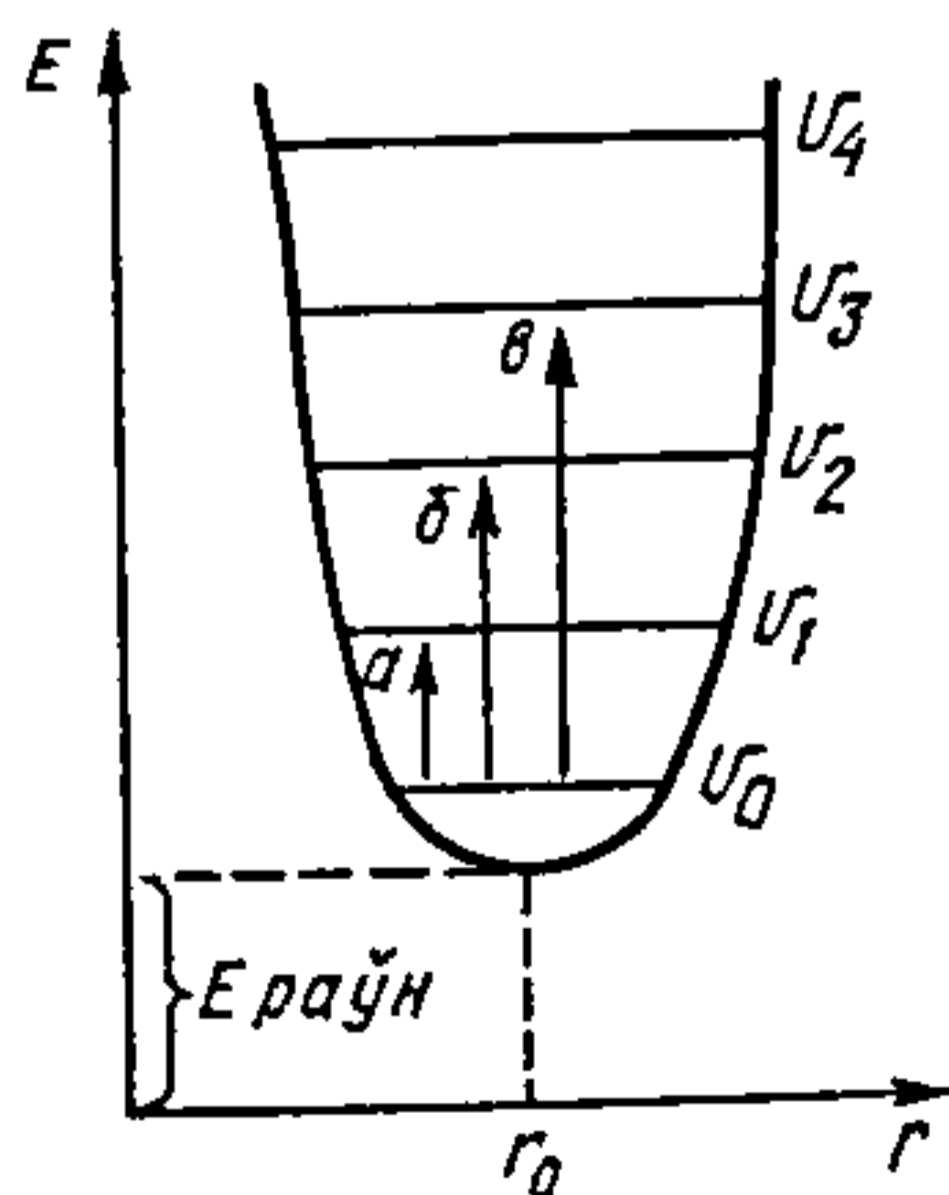
Рыс. 25.2.2. Залежнасць патэнцыяльнай энергіі E гарманічнага асцылятара ад міжатамнай адлегласці r :
