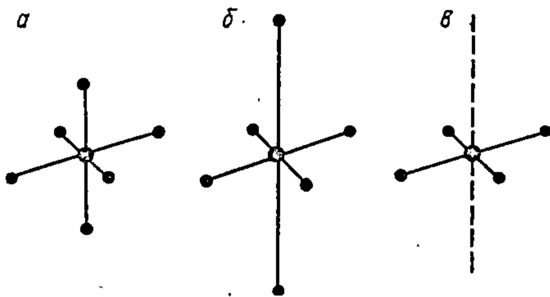
Рыс. 22.3.8. Пераход ад актаэдрычнага (а) да плоскаквadratнага размяшчэння лігандаў вакол іонаў з цалкам (б) і часткова заселенымі (в) d -арбіталямі.
