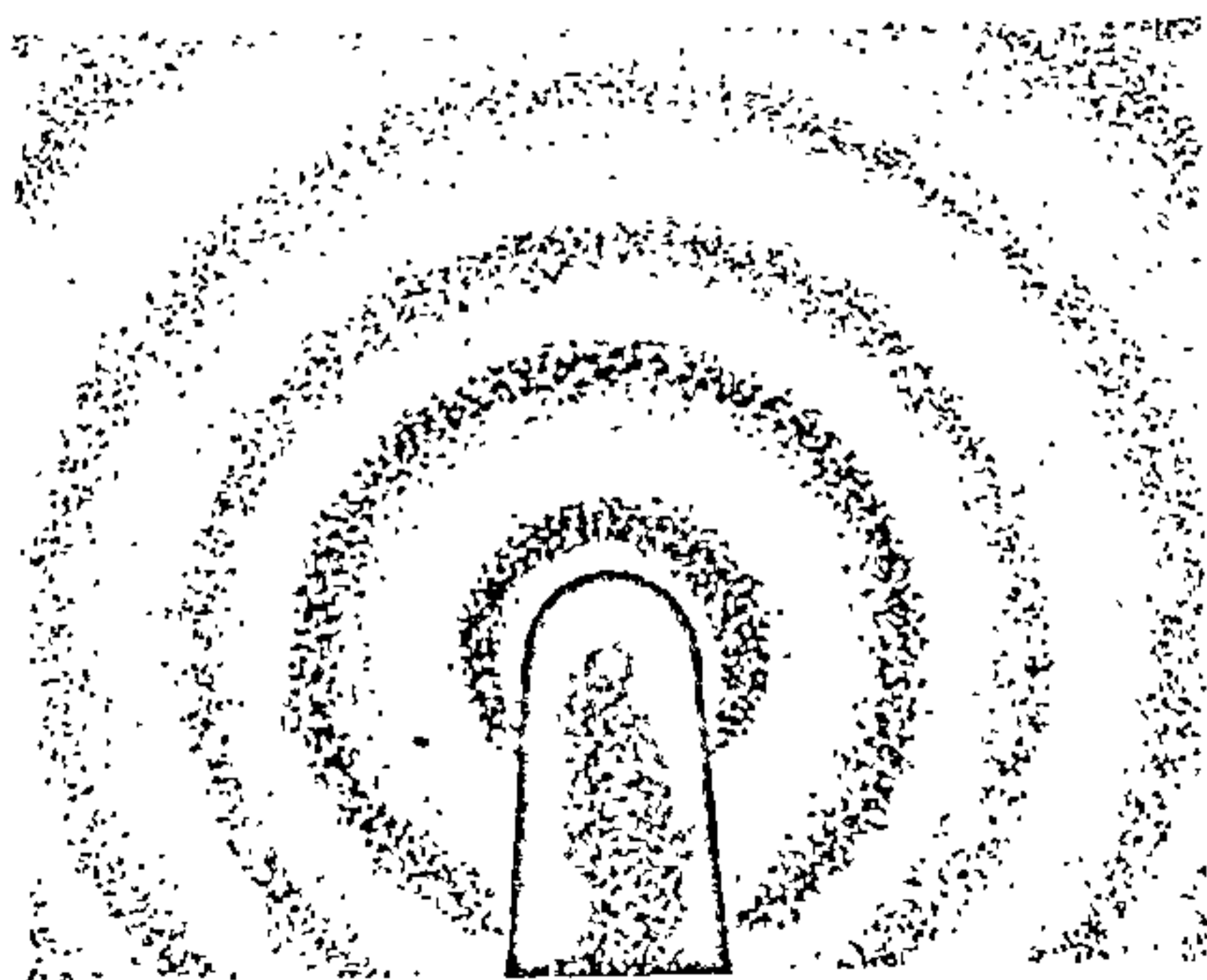
Рыс. 18.4.1. Электронаграма пары оксітэтрахларыду вальфраму.
