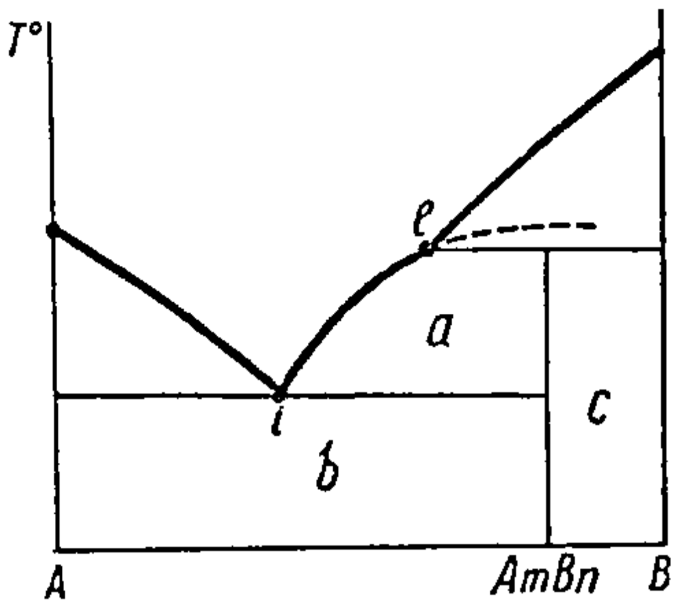
Рис. 7.6.4. Дыяграма плаўкасці з утварэннем у крышталічнай фазе дваінога злучэння, якое плавіцца інкангруэнтна: a, b, c — двухфазныя вобласці; l — перытэкта; i — эўтэкта.
