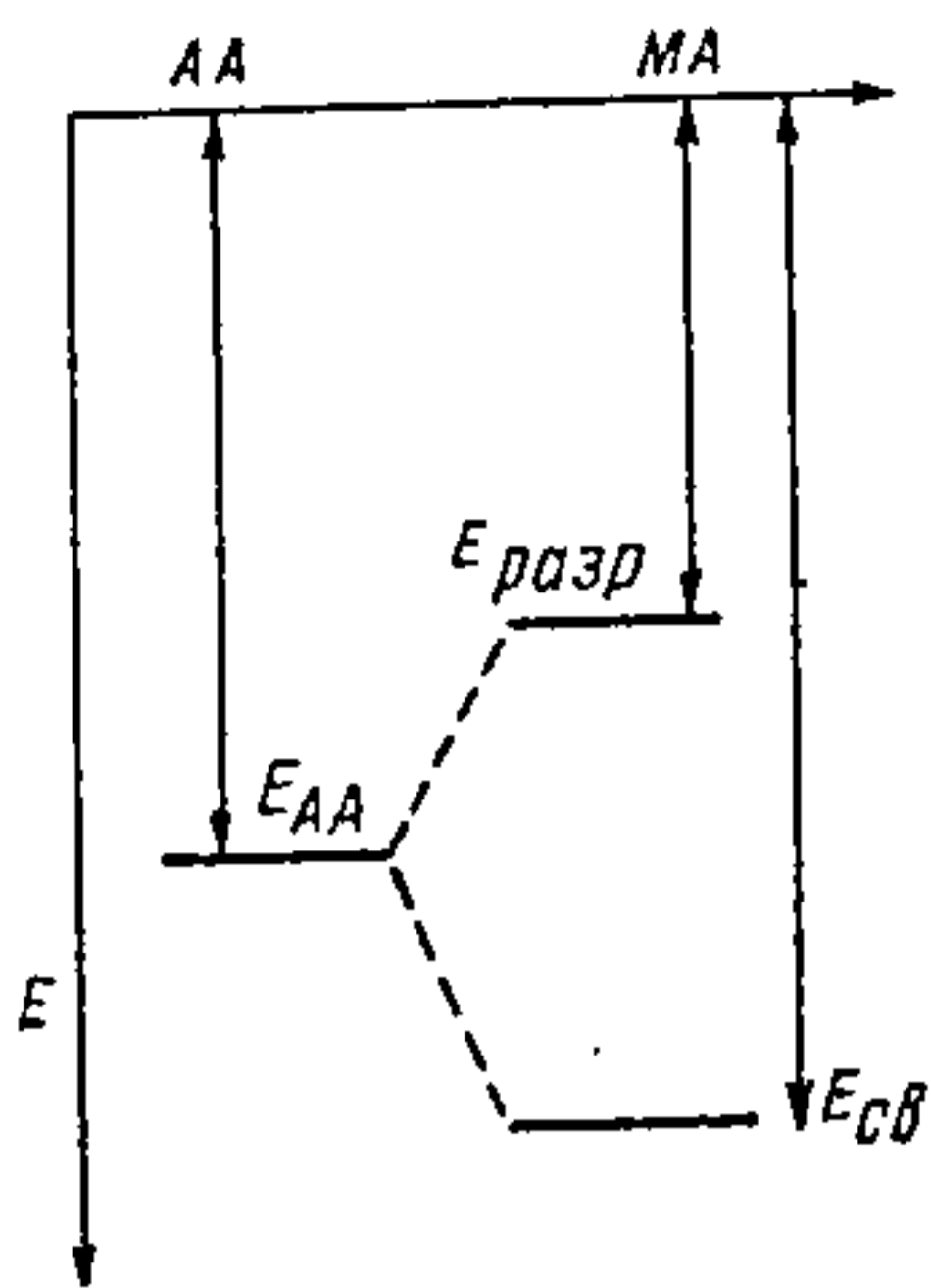
Рис. 23.3.2. Энергетичныя ўзроўні малекулярных арбіталей іона \text{H}_2^+ .
