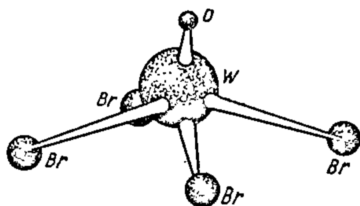
Рыс. 18.5.8. Структурная мадэль малекулы \text{WOBr}_4 сіметры C_{4v} .
