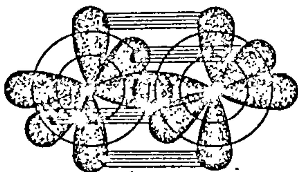
Рыс. 21.1.6. Схема сувязей у малекуле N_2 .
