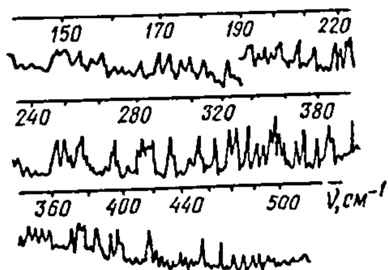
Рыс. 25.4.2. Вярчальны спектр малекул вады.
