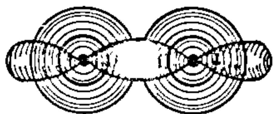
Рыс. 21.1.4. Схема малекулы \text{B}_2 , утворанай няўзбуджанымі атамамі бору.
