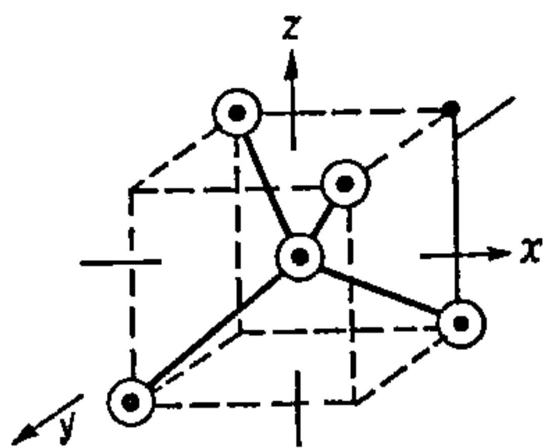
Рис. 22.3.5. Тэтраэдричнае размяшчэнне лігандаў каля цэнтральнага атама.
