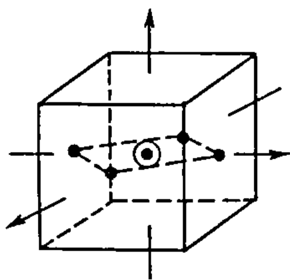
Рыс. 22.3.7. Плоскаквadratнае размяшчэнне лігандаў вакол іона \text{Cu}^{2+} .
