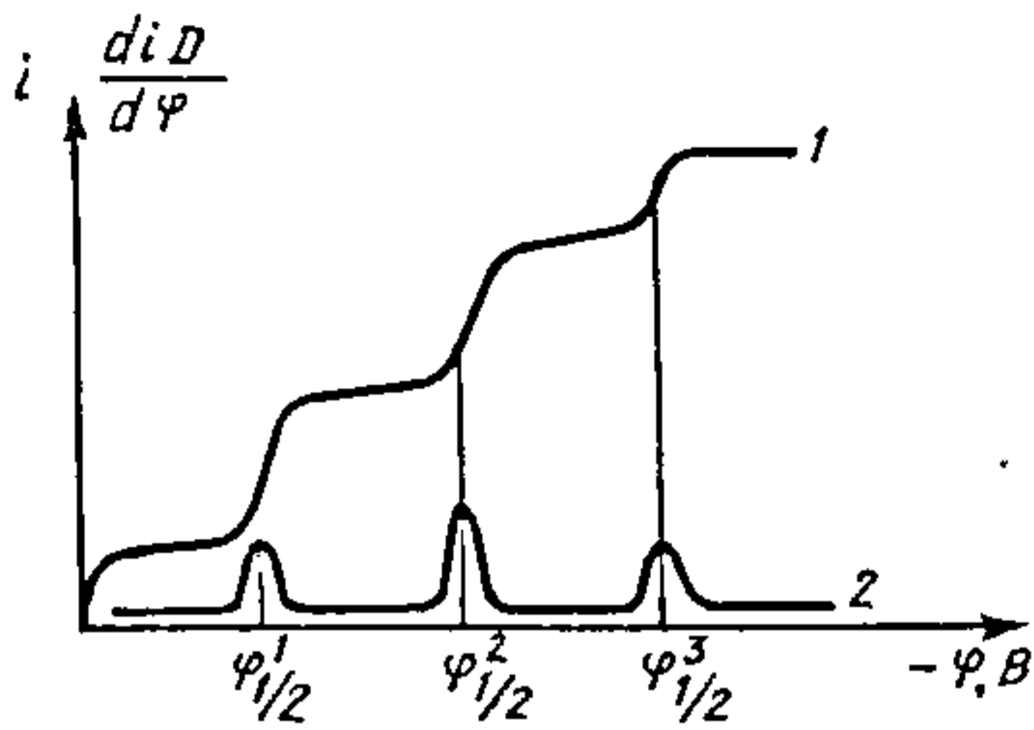
Рис. 13.6.1. Типовы вигляд диференціальнай паляраграмы: 1 — прамая паляраграма |i_D=f(-\varphi)| , 2 — диференціальная \left[ \frac{di_D}{d\varphi} = f(-\varphi) \right] .
