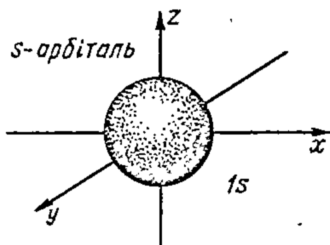
Рыс. 17.5.1. Электронная s -воблака ( l=0 ).
