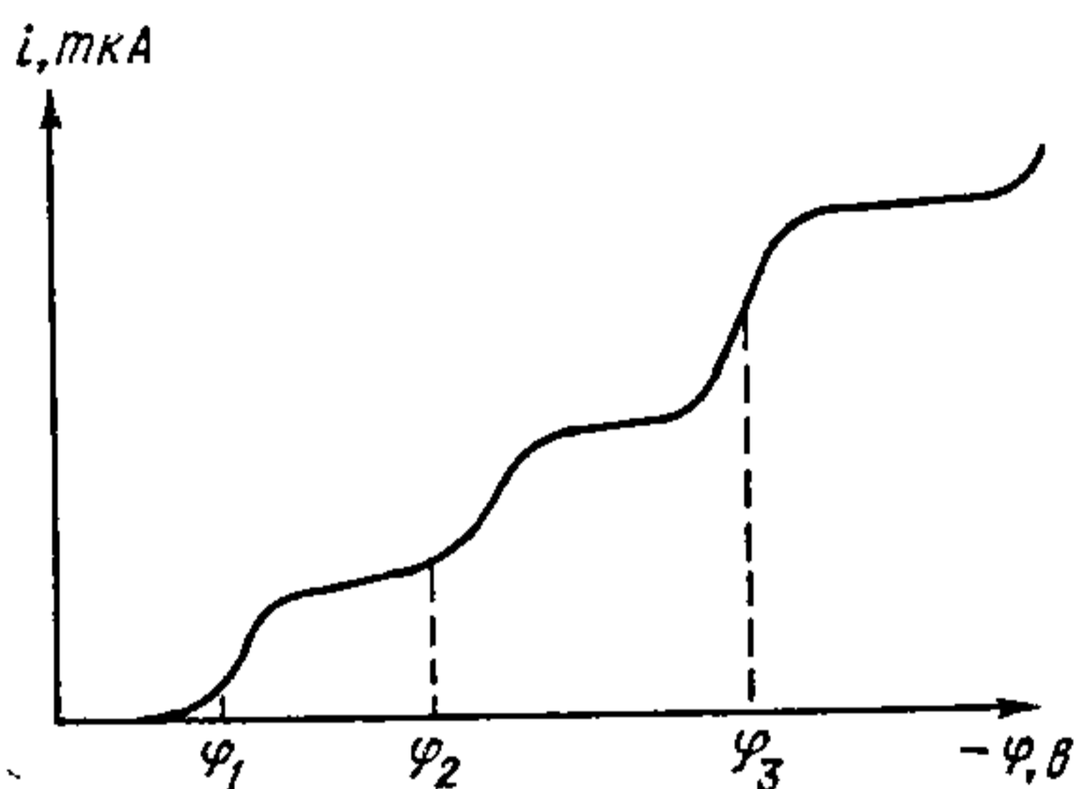
Рыс. 13.4.3. Паляраграма раствору, які ўтрымлівае некалькі іонаў.
