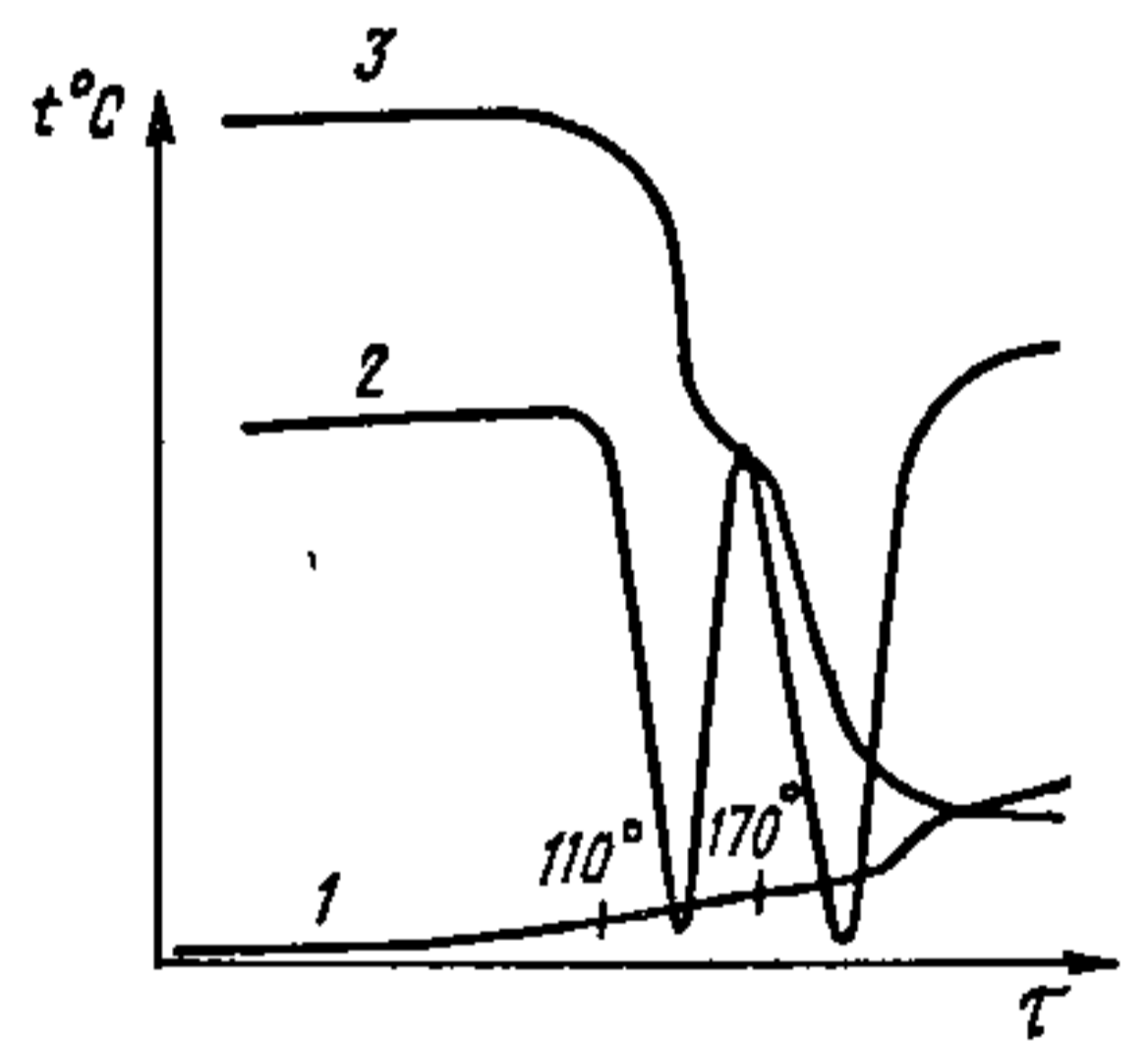
Рыс. 7.9.2. Тэрмаграма крышталегідрату \text{BaCl}_2 \cdot 2\text{H}_2\text{O} : 1 — крывая нагрэву; 2 — дыферэнцыяльная крывая; 3 — крывая гравіметрыі.
