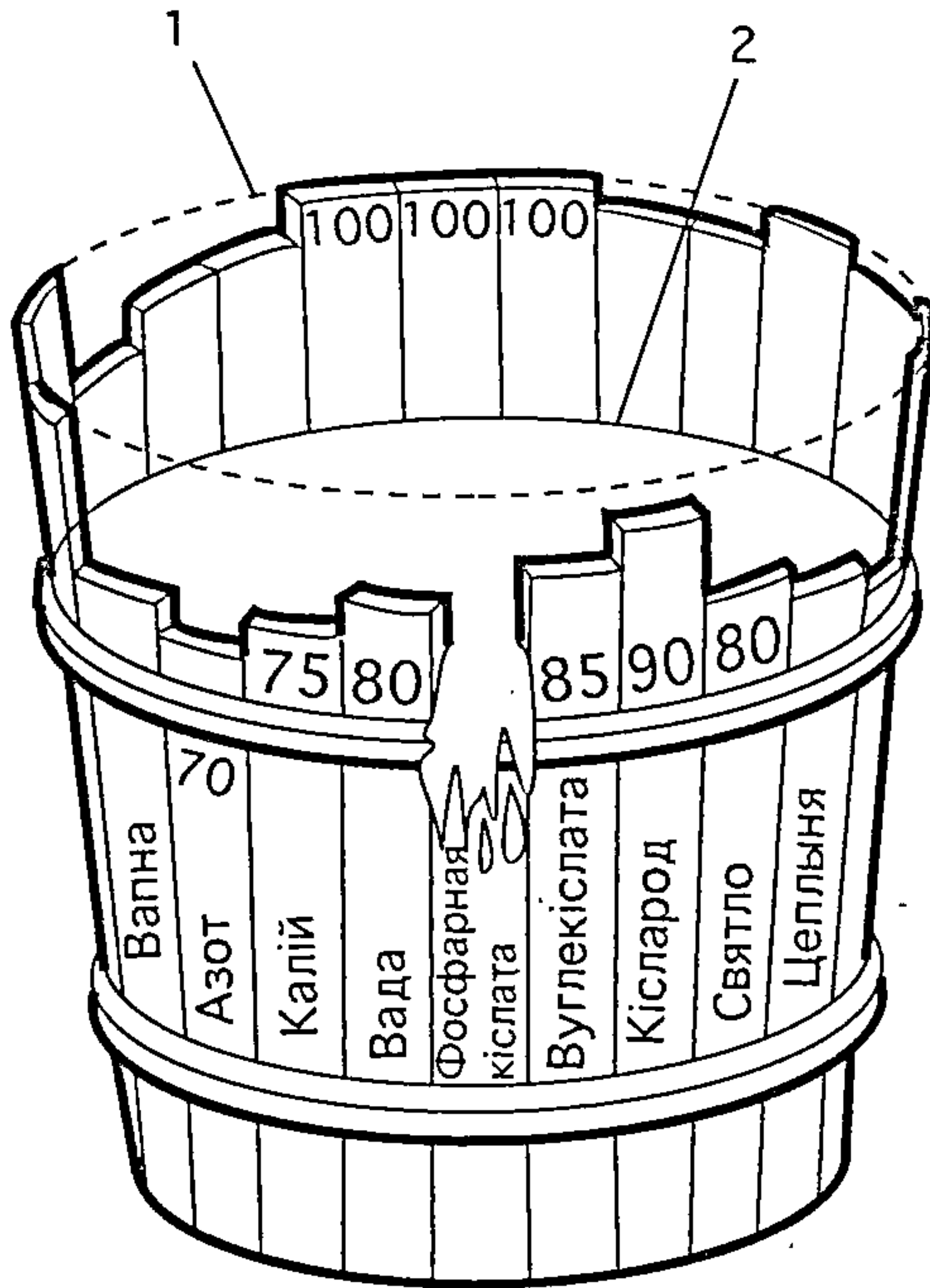
10.1. Графічнае адлюстраванне закона мінімуму (“бочка Дабенека”): 1 — максімальна магчымы ўраджай; 2 — фактычны ўраджай.
