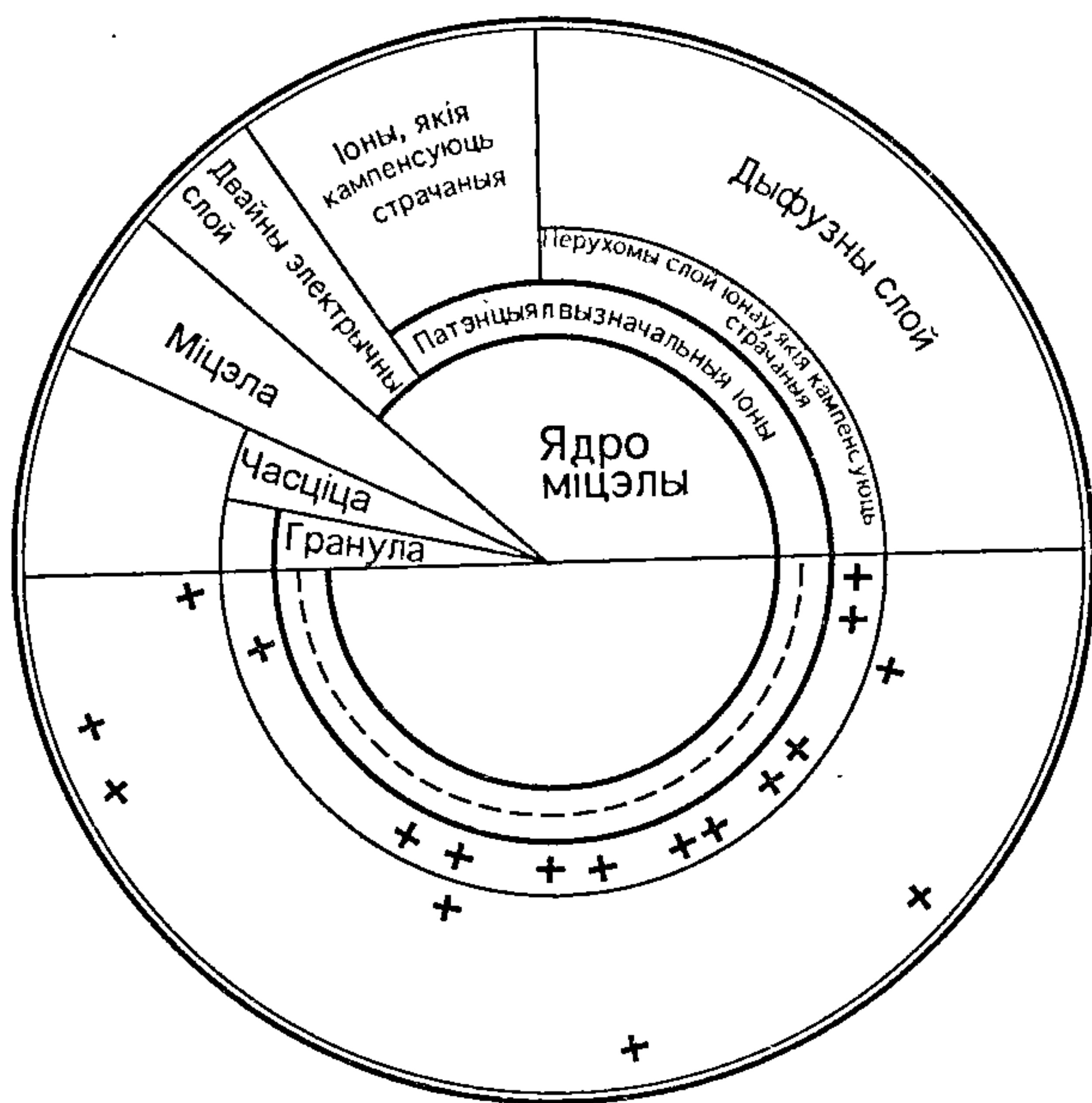
2.1. Схема будовы калоіднай міцэлы (па Гарбунову)
