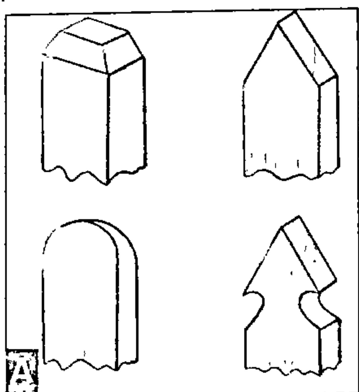
Агароджы. А. Прыклады афармлення верху штыкетцін. Б. Спосабы мацавання слупкоў. В. Агароджа з цэглы. Г. Агароджа з цагляных слупоў і дрэва. Д. Агароджа з бетонных слупкоў і дрэва. Е. Прыклады агароджаў з дрэва (а—е). Ж. Прыклады дэкаратыўных агароджаў: а — з цэглы (каменю) ці дрэва; б — з керамікі і металу; в — з неакораных жордак.
