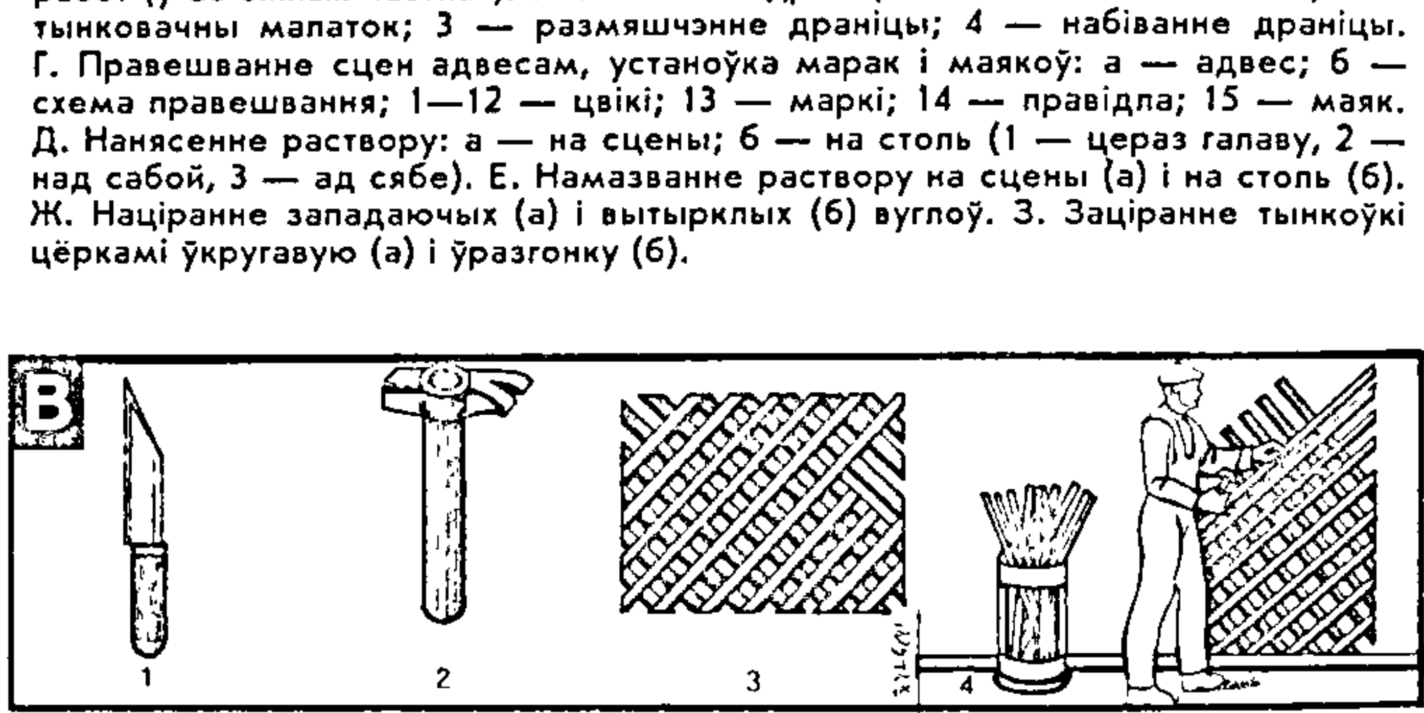
Тынкавальныя работы. А. Інструменты для тынкавальных работ: 1 — кельня тынкавальная; 2 — цёрка; 3 — паўцёрка; 4 — правідла; 5 — шпатэлі; 6 — фасонныя паўцёркі; 7 — пэндзаль-маклавіца. Б. Саставы раствораў для тынкавальных работ (у аб'ёмных частках). В. Набіванне драніцы: 1 — тынкавачны нож; 2 — тынкавачны малаток; 3 — размяшчэнне драніцы; 4 — набіванне драніцы. Г. Правешванне сцен адвесам, устаноўка марак і маякоў: а — адвес; б — схема правешвання; 1—12 — цвікі; 13 — маркі; 14 — правідла; 15 — маяк. Д. Нанясенне раствора: а — на сцены; б — на столь (1 — цераз галаву, 2 — над сабой, 3 — ад сябе). Е. Намазанне раствора на сцены (а) і на столь (б). Ж. Націранне западаючых (а) і вытырклых (б) вуголь. З. Заціранне тынкоўкі цёркамі ўкругавую (а) і ўразгонку (б).
