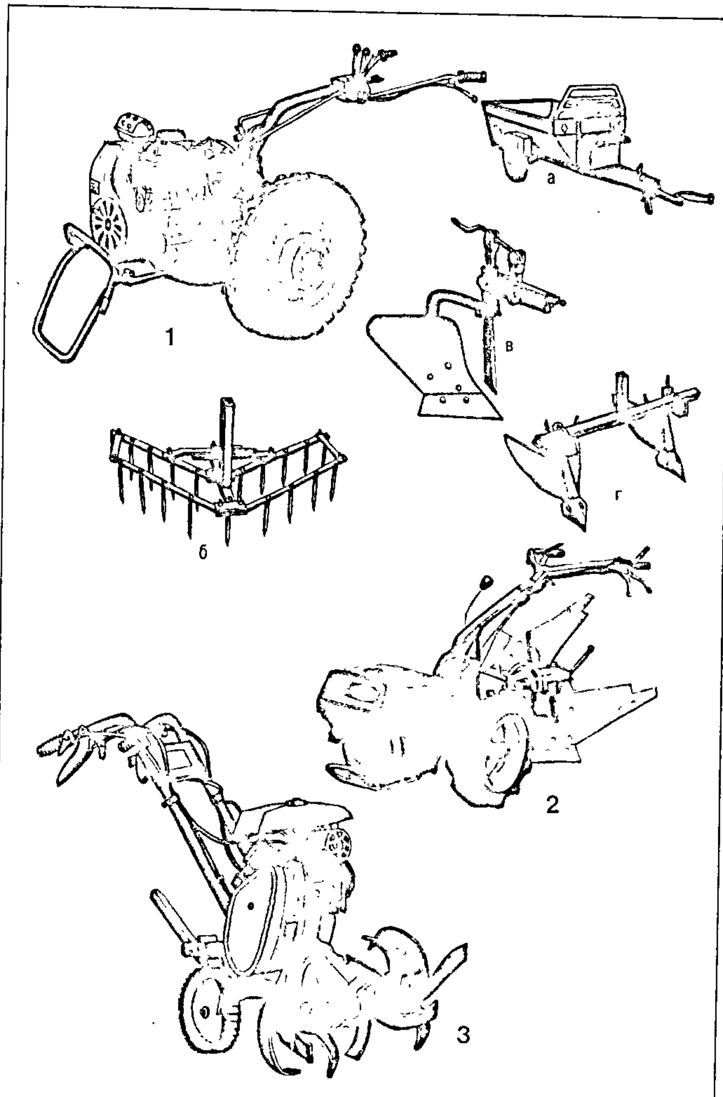
Мотамалышы на падвор'і. 1. Мотаблок МТЗ-0,5 "Беларусь" і прылады да яго: а — цялежка, б — барана, в — плуг, г — акучнік. 2. Мотаблок "Супер-600". 3. Мотакультыватар МК-1 "Крот".
