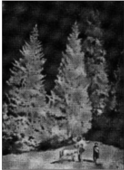
Мал. 12. Елка цянь-шаньская. Здымак у інфрачырвоных промнях
