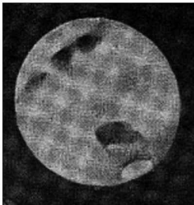
Мал. 1. Пулкава. 13 красавіка 1918 г. Светлачырвоны святлафільтр
