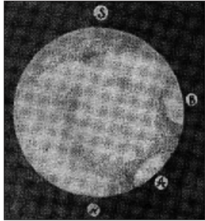
Мал. 6. Ташкент. 10 лютага 1948 г. Чырвоны святлафільтр. А — паўночная палярная шапка. В — светлая пляма ў месцы ўсходу Сонца
